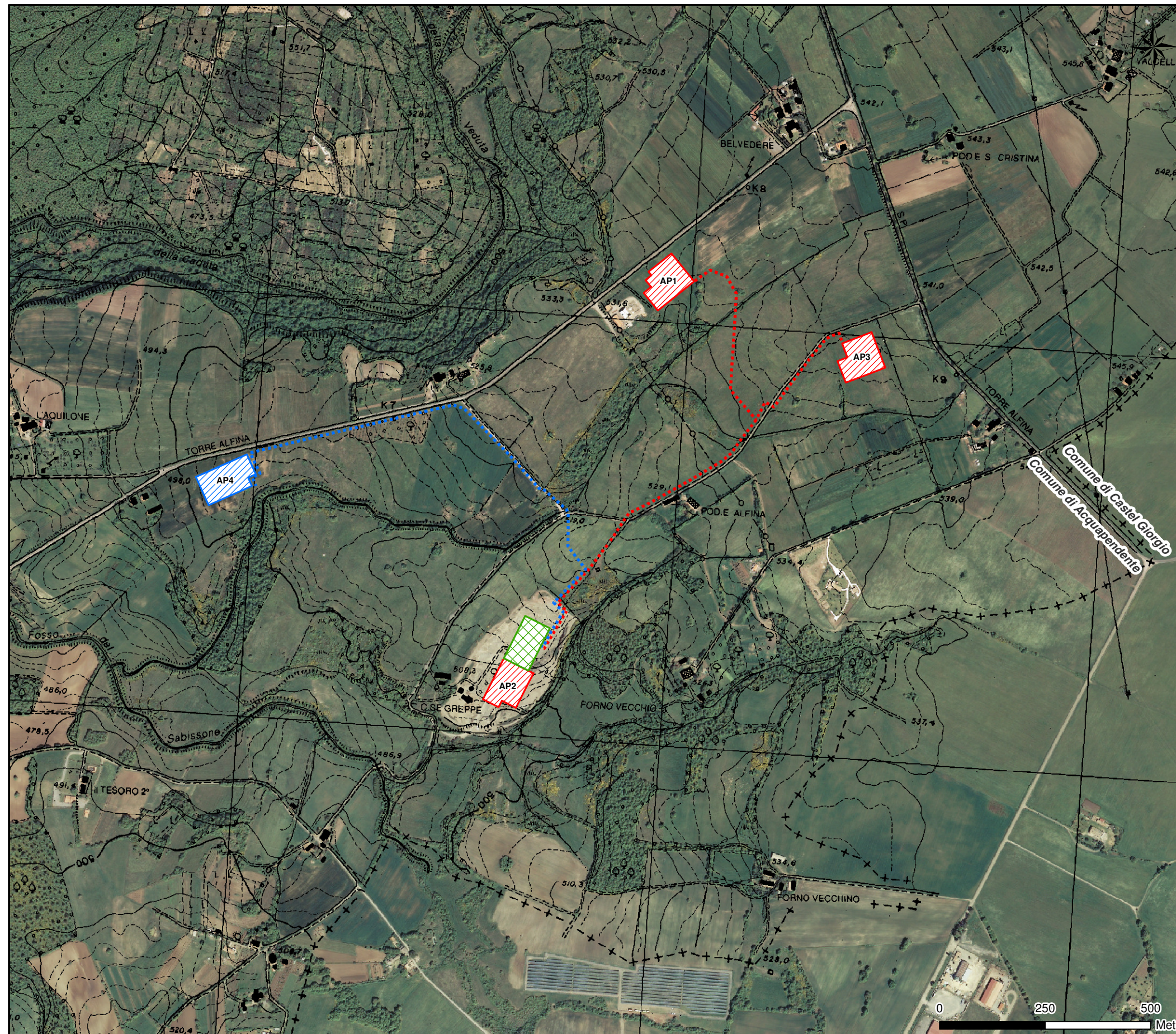
Figura 1a Localizzazione Impianto Pilota Geotermico "Torre Alfina" su Carta Tecnica Regionale e Ortofoto (Scala 1:10.000)
