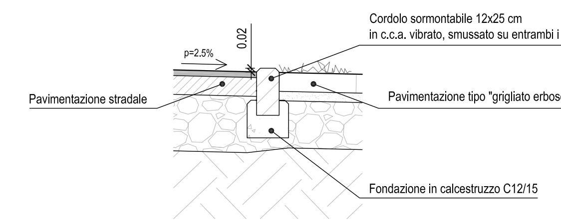
- PARTICOLARE 1 - DETTAGLIO CORDOLO SORMONTABILE SCALA 1:20
