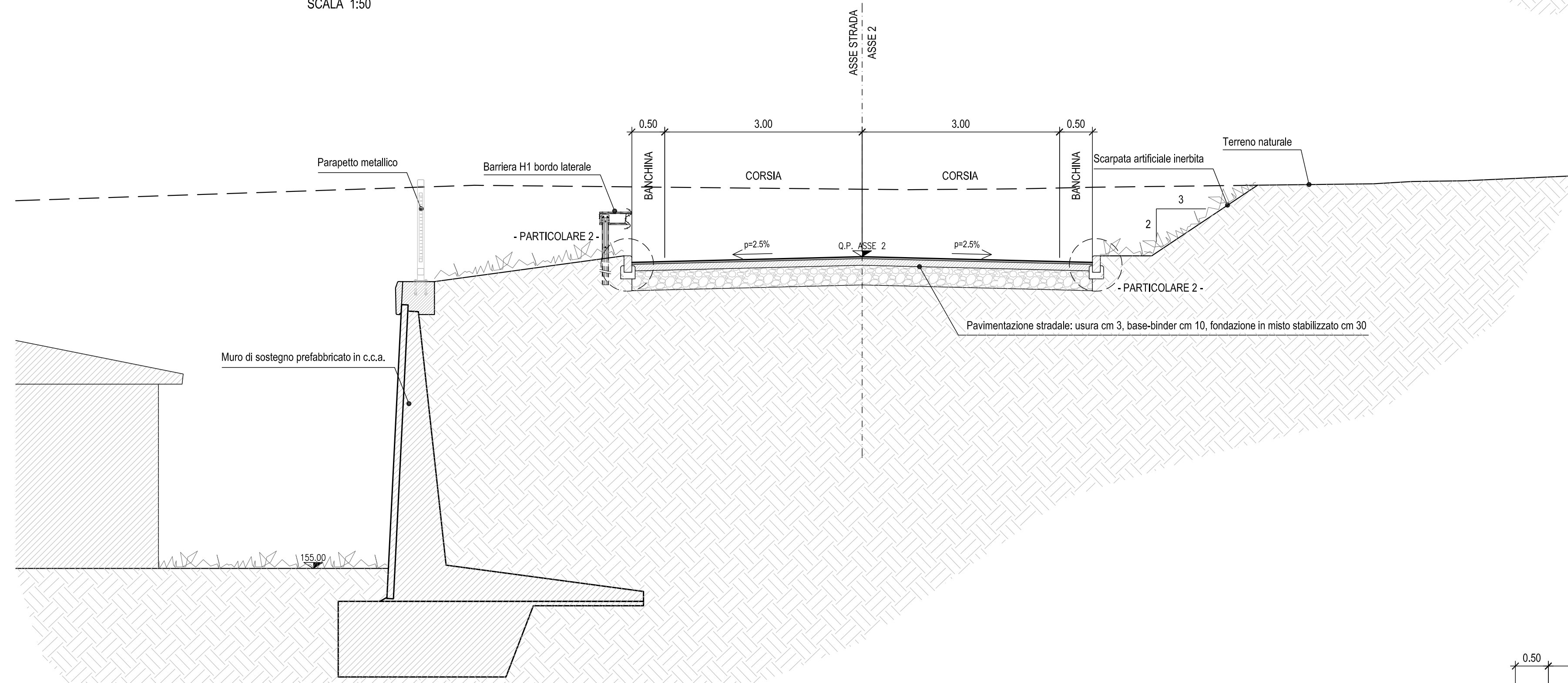
SEZIONE TIPO - ASSE 2 RAMPA SCALA 1:50
