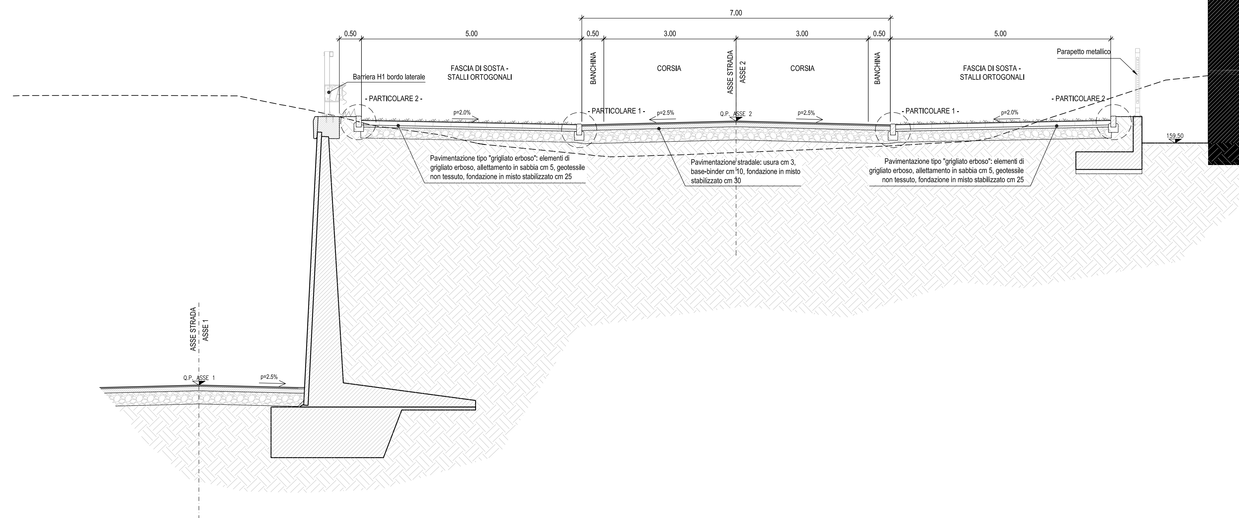
SEZIONE TIPO - ASSE 2 PARCHEGGIO SCALA 1:50
