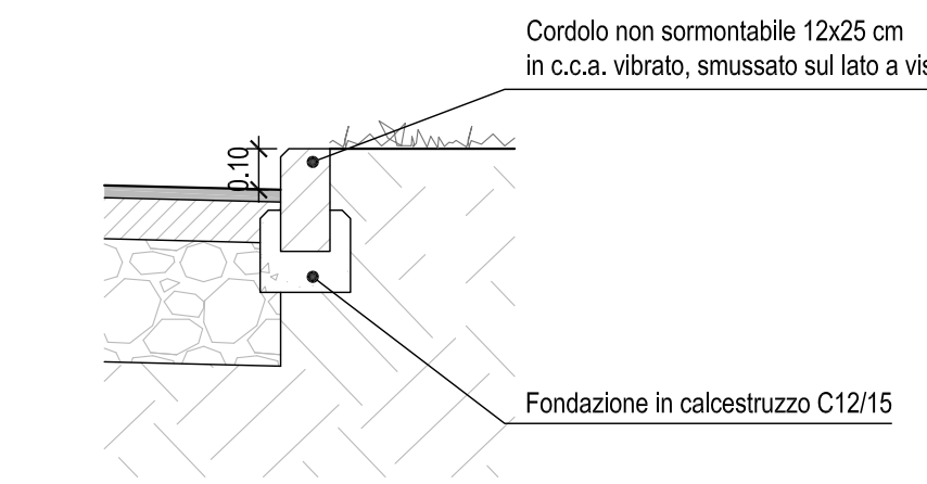
- PARTICOLARE 2 - DETTAGLIO CORDOLO NON SORMONTABILE SCALA 1:20
