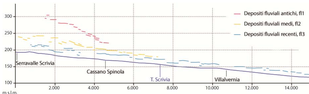
Figura 7: Profilo morfostratigrafico del Torrente Scrivia realizzato nel tratto compreso tra gli abitati di Serravalle Scrivia e Villalvernia e riferito al versante idrografico sinistro della Valle Scrivia (non sono stati rappresentati gli ordini di terrazzi riferibili all'evoluzione recente del T. Scrivia - depositi fluviali attuali (a) - in quanto scarsamente rilevanti ai fini dell'opera).
