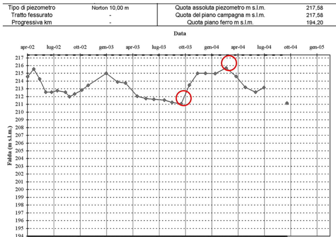
Figura 12 – Grafico delle fluttuazioni del livello piezometrico nel foro EA301R044; i cerchi indicano la soggiacenza minima e massima (cfr. tabella seguente).
