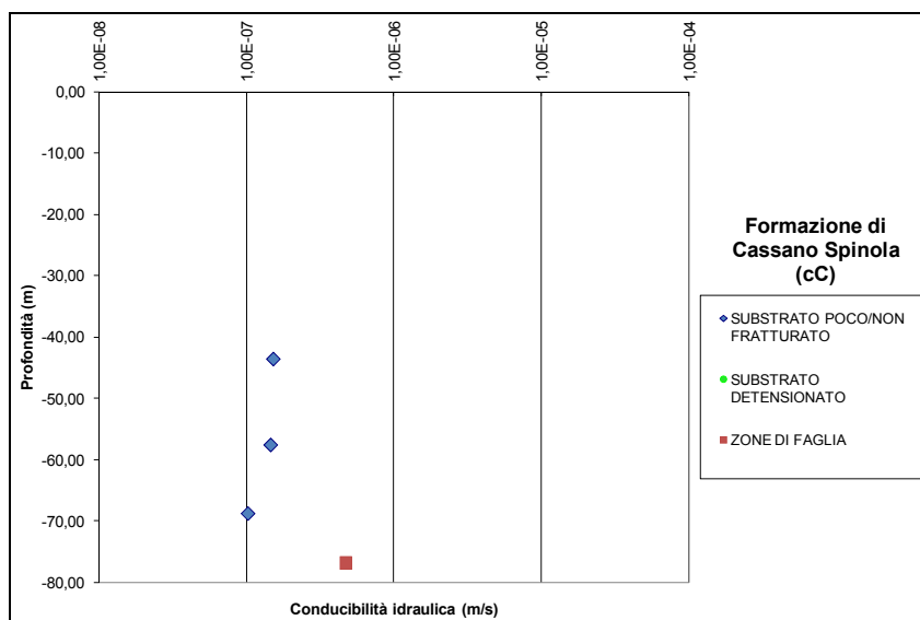
Figura 10 - Grafico delle conducibilità idrauliche per la formazione di Cassano Spinola da prove sui sondaggi del PP, PD e PE.
