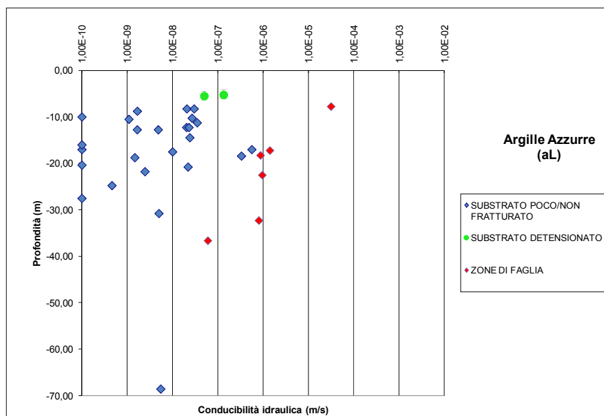
Figura 9 - Grafico delle conducibilità idrauliche per le Argille Azzurre da prove sui sondaggi del PP, PD e PE. (N.B.: i dati relativi alle “zone di faglia” sono attendibili solo per i valori di permeabilità inferiori).
