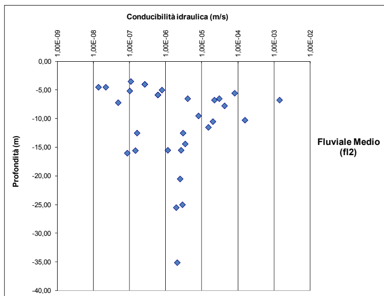
Figura 8 - Grafico delle conducibilità idrauliche per i depositi alluvionali medi (f12) da prove sui sondaggi del PP, PD e PE.
