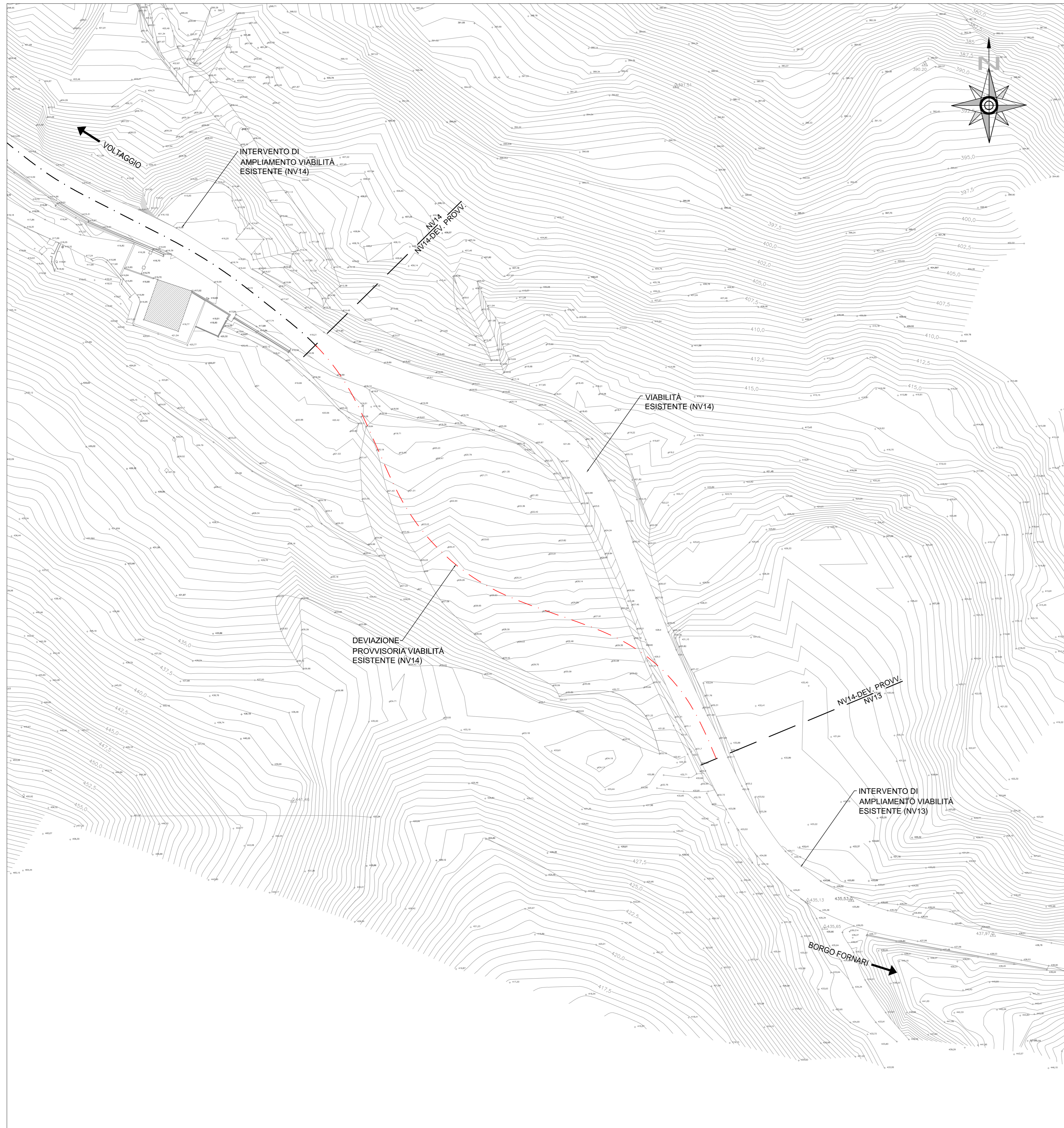
PLANIMETRIA STATO ATTUALE (Scala1:500)
