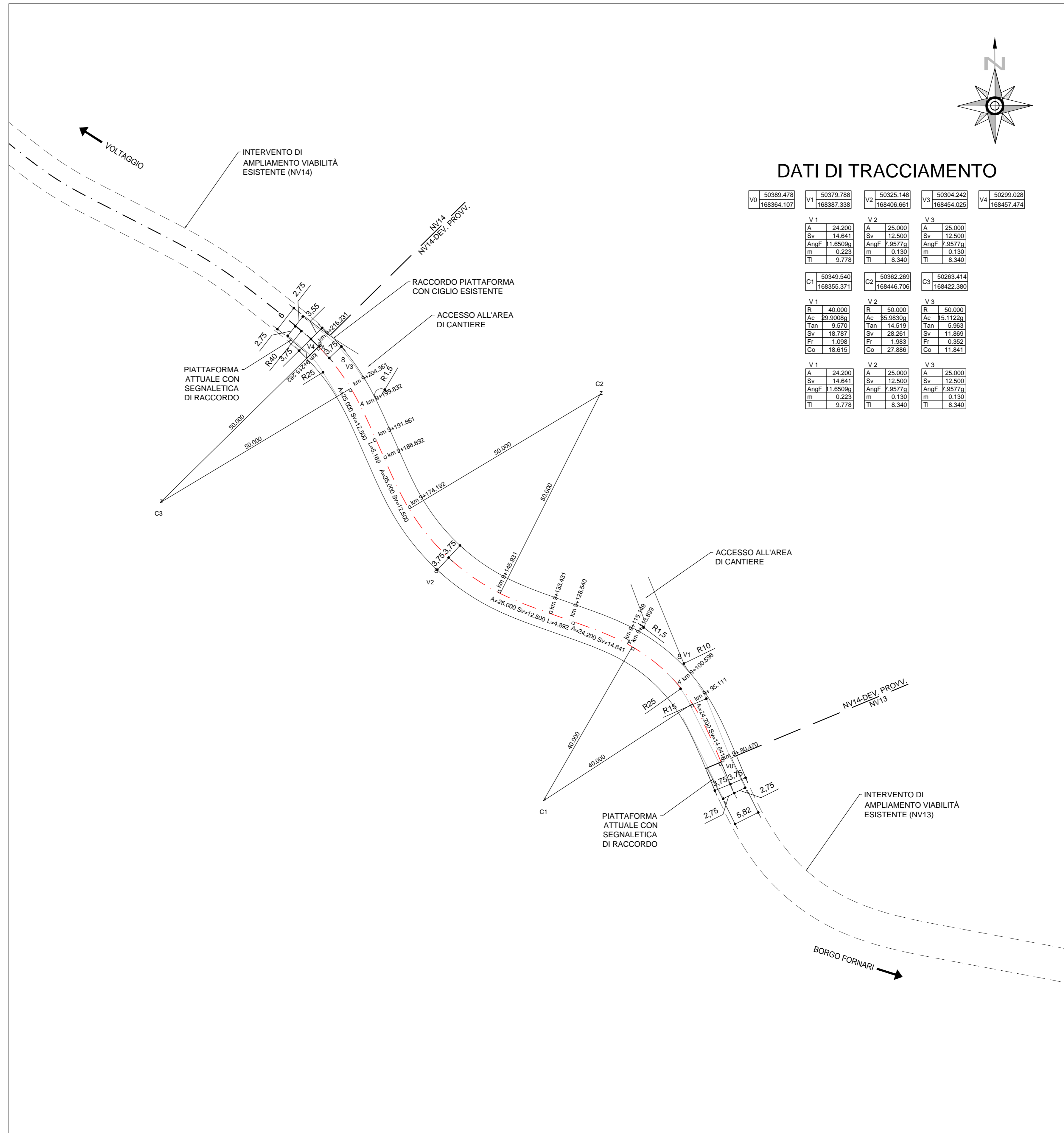
PLANIMETRIA DI TRACCIAMENTO (Scala1:500)
