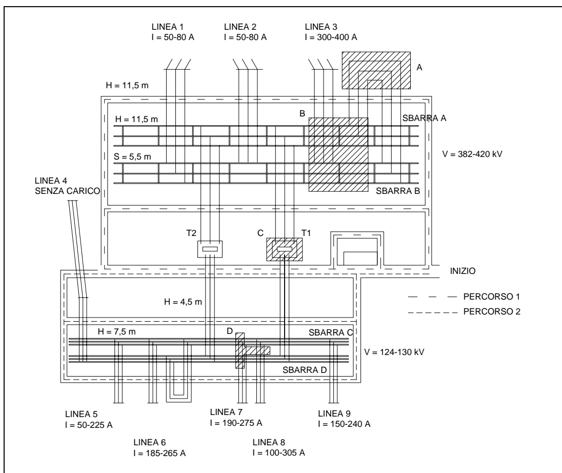
Fig. 1 – Pianta di una tipica stazione 380/132 kV con l'indicazione delle principali distanze fase-fase (S) e fase-terra (H) e delle variazioni delle tensioni e delle correnti durante la fasi di misurazioni di campo elettrico e magnetico.
