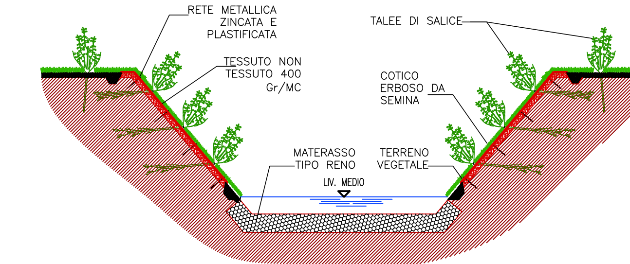
RIPROFILATURA FOSSO IN TERRA ESISTENTE – TIPOLOGICO
