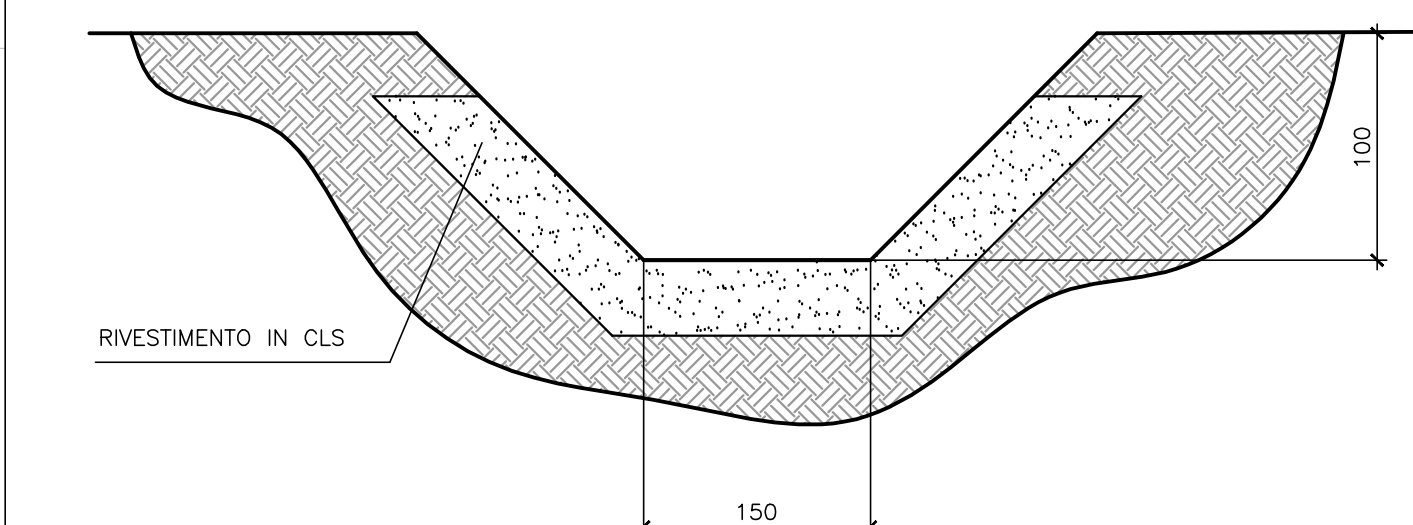
CANALE DI GRONDA IN CLS – TIPOLOGICO
