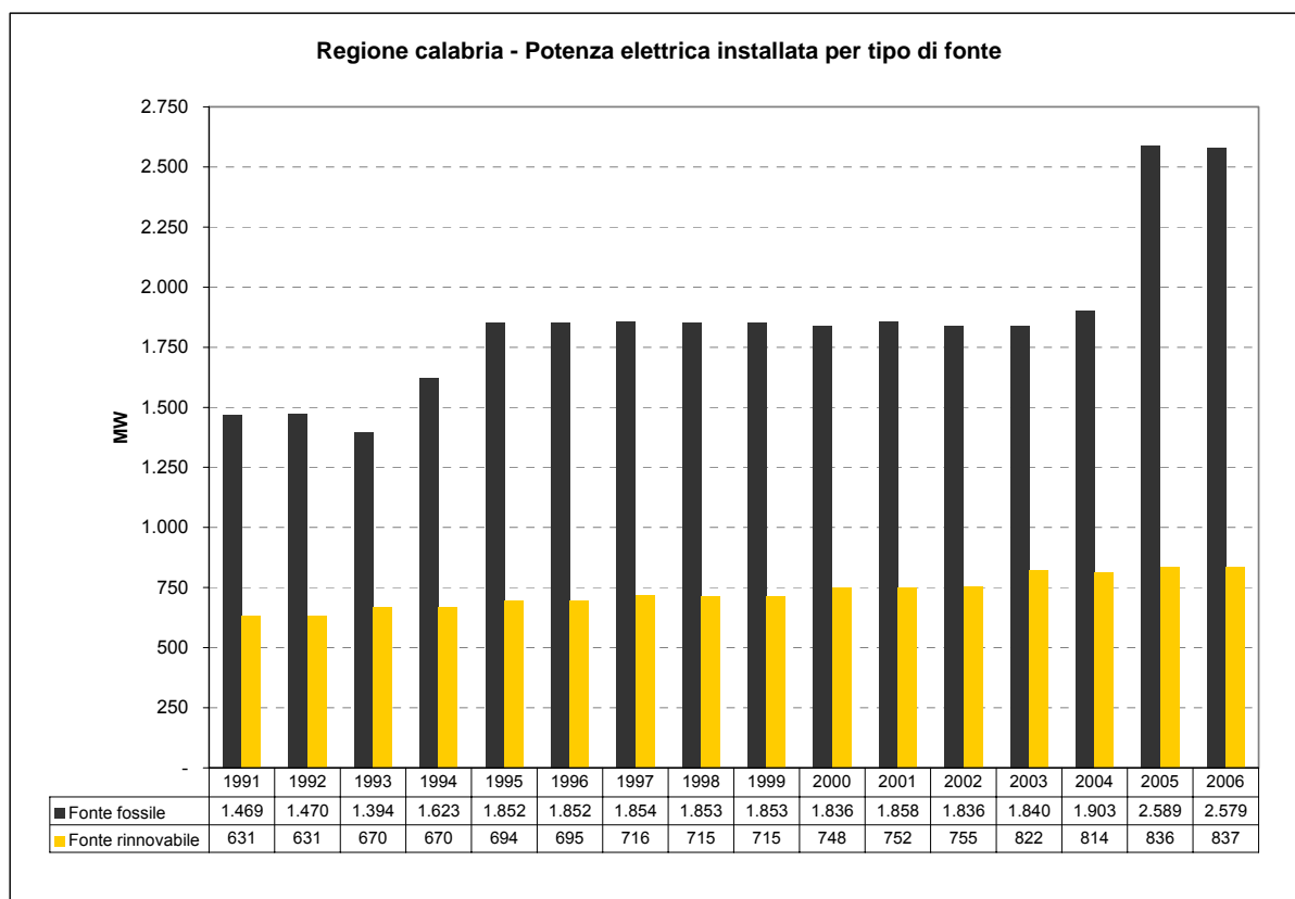
Grafico 3.13 Elaborazioni Ambiente Italia su dati Terna
