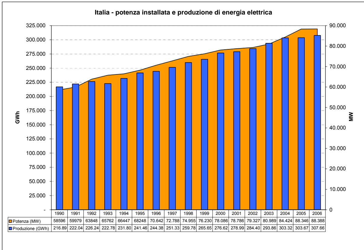
Grafico 3.1 Elaborazioni Ambiente Italia su dati Terna
