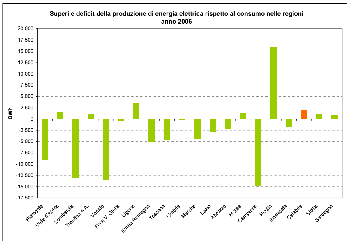
Grafico 3.12 Elaborazioni Ambiente Italia su dati Terna
