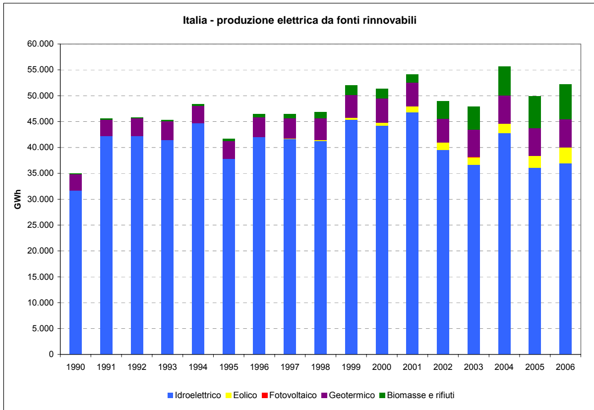
Grafico 3.7 Elaborazioni Ambiente Italia su dati Terna
