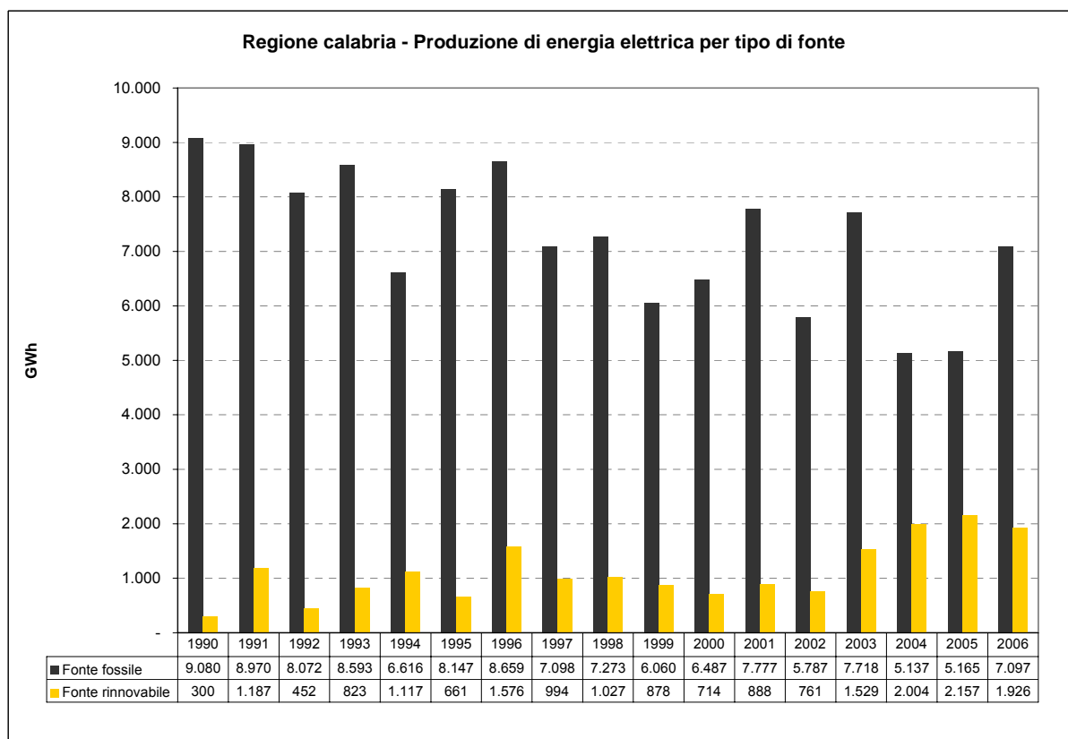
Grafico 3.14 Elaborazioni Ambiente Italia su dati Terna
