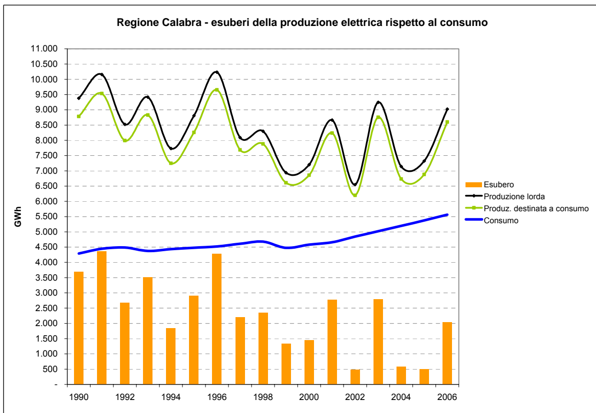
Grafico 3.11 Elaborazioni Ambiente Italia su dati Terna
