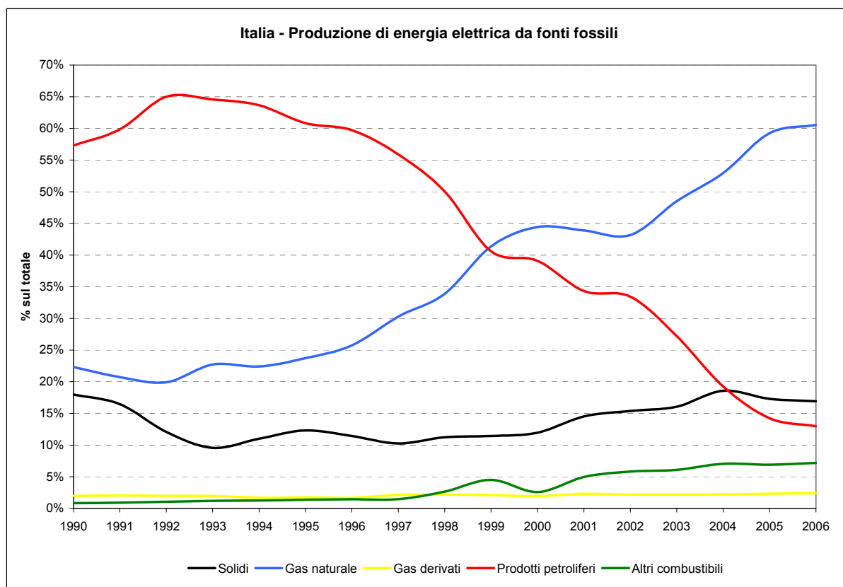
Grafico 3.6 Elaborazioni Ambiente Italia su dati Terna
