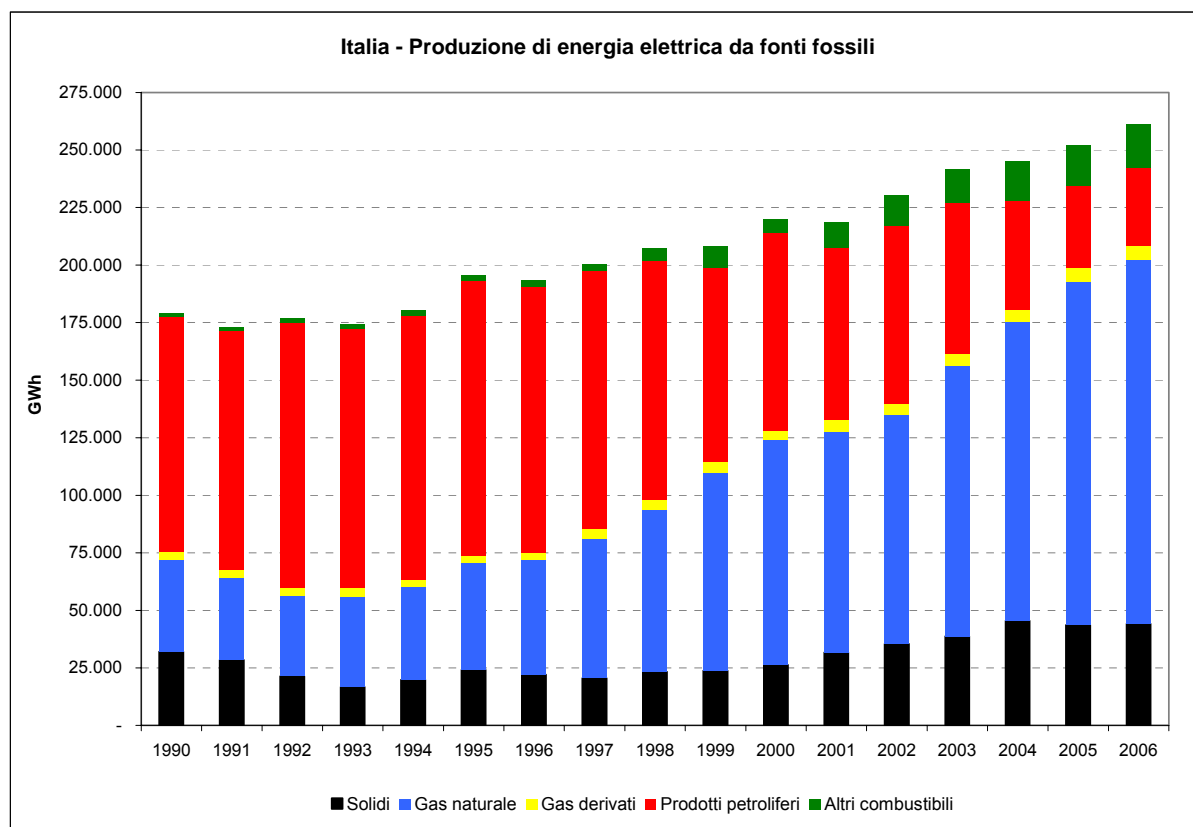
Grafico 3.5 Elaborazioni Ambiente Italia su dati Terna
