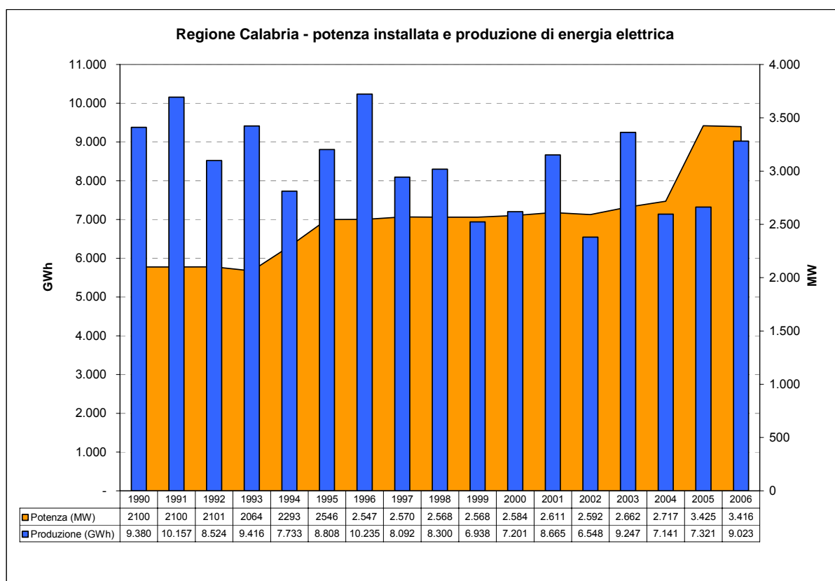
Grafico 3.9 Elaborazioni Ambiente Italia su dati Terna
