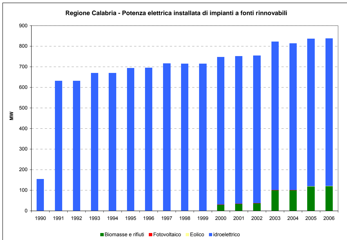
Grafico 3.16 Elaborazioni Ambiente Italia su dati Terna
