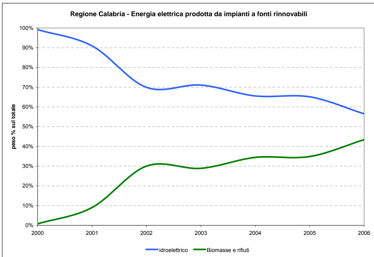
Grafico 3.18 Elaborazioni Ambiente Italia su dati Terna
