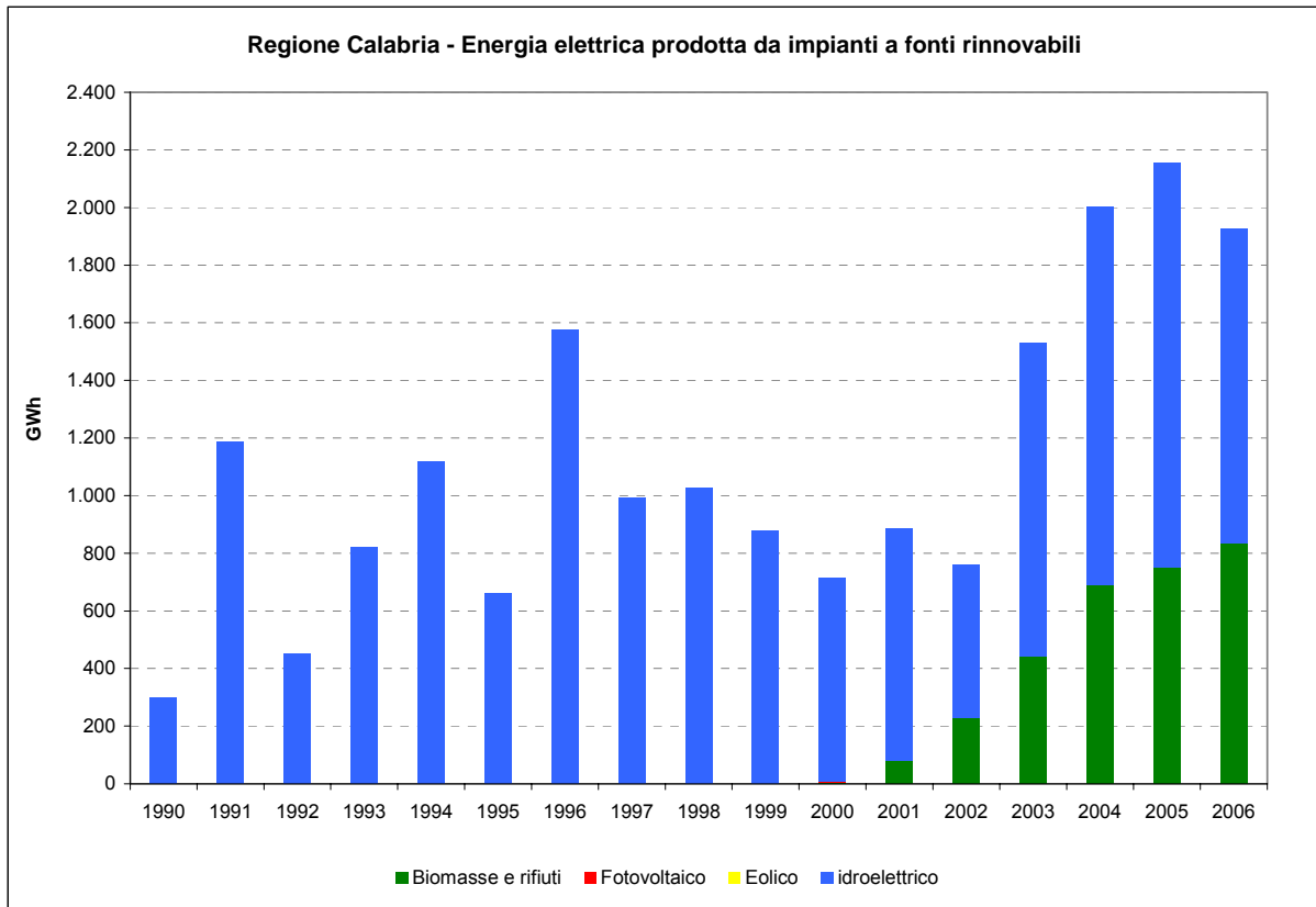
Grafico 3.17 Elaborazioni Ambiente Italia su dati Terna
