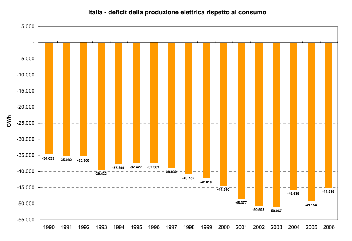
Grafico 3.2 Elaborazioni Ambiente Italia su dati Terna
