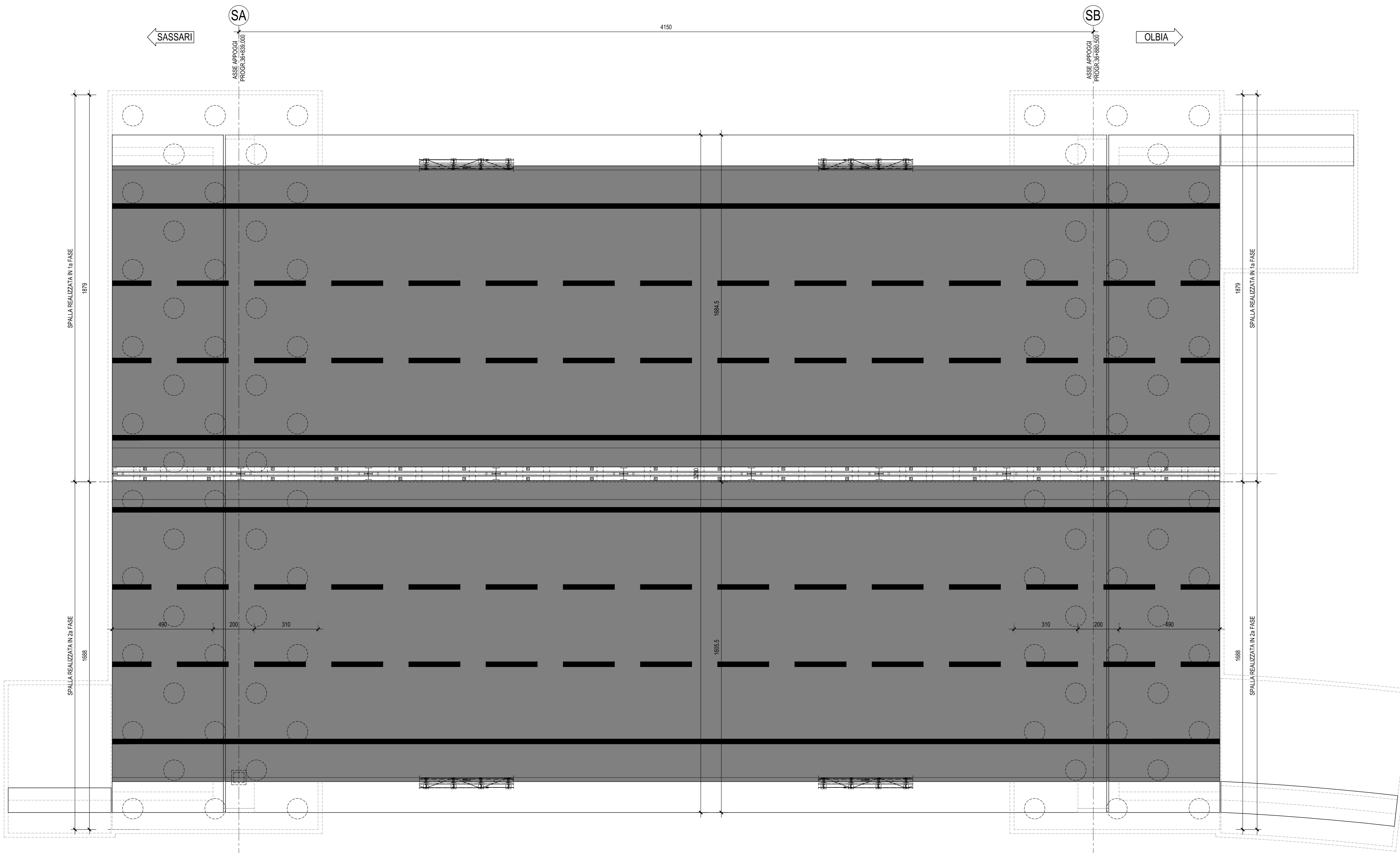
PIANTA IMPALCATO-Scala 1:100
