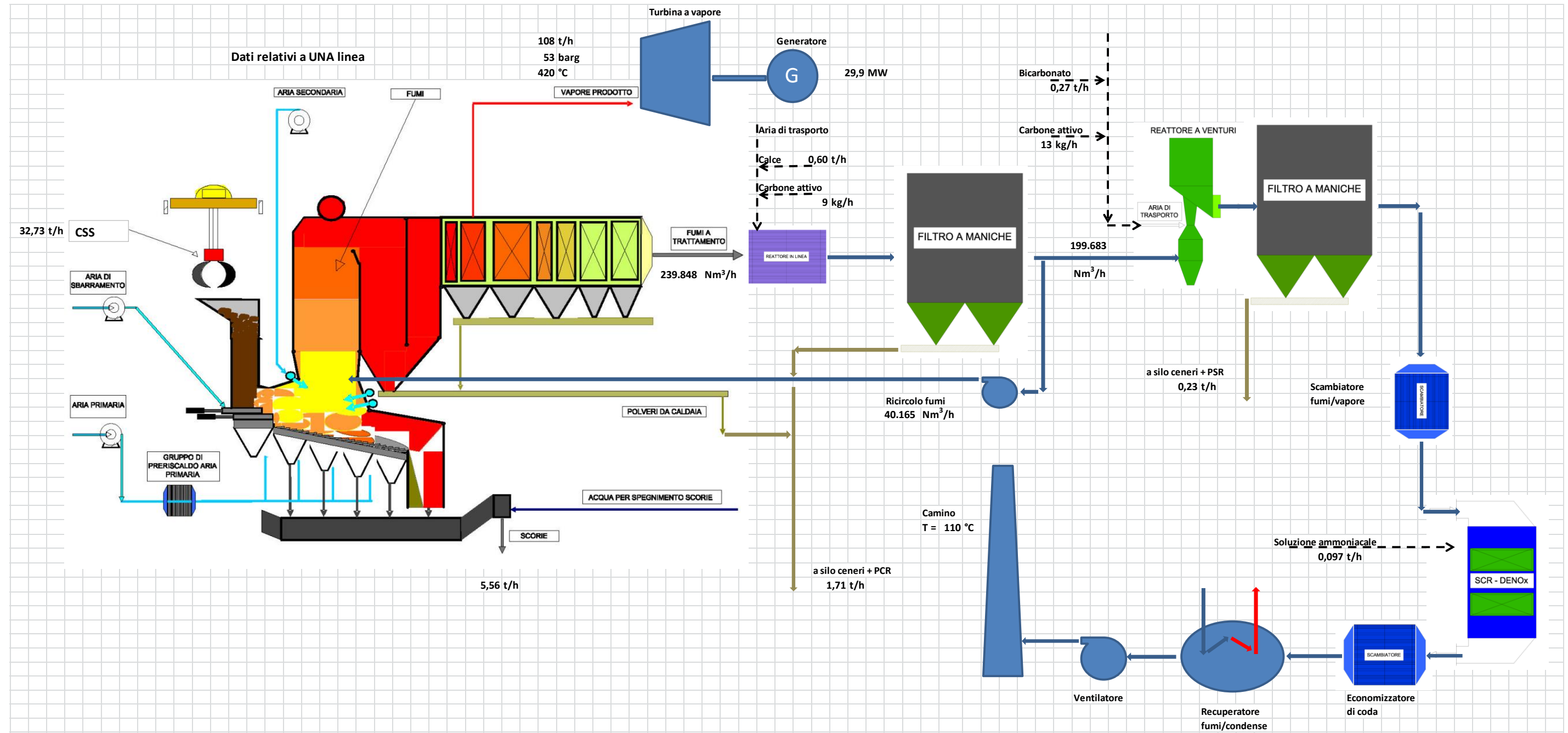
Figura 3.3.4a Schema di funzionamento TMV
