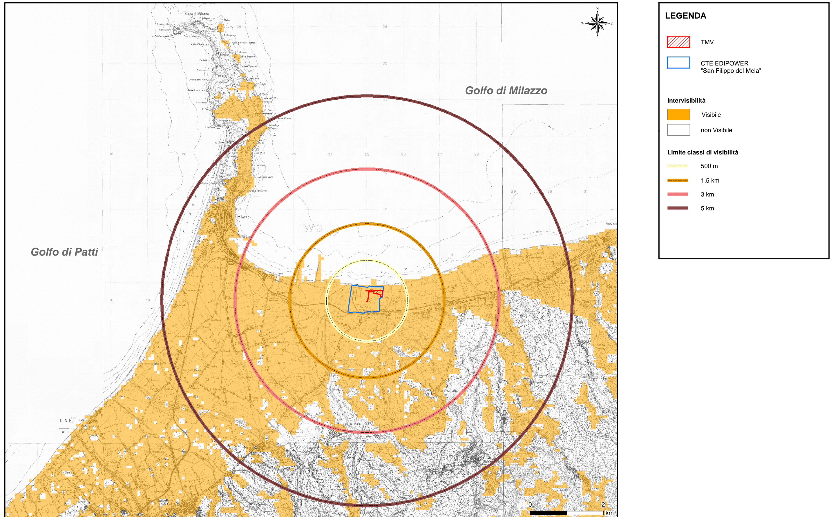
Figura 4.3.8.2b Elaborazione carta dell'intervisibilità
