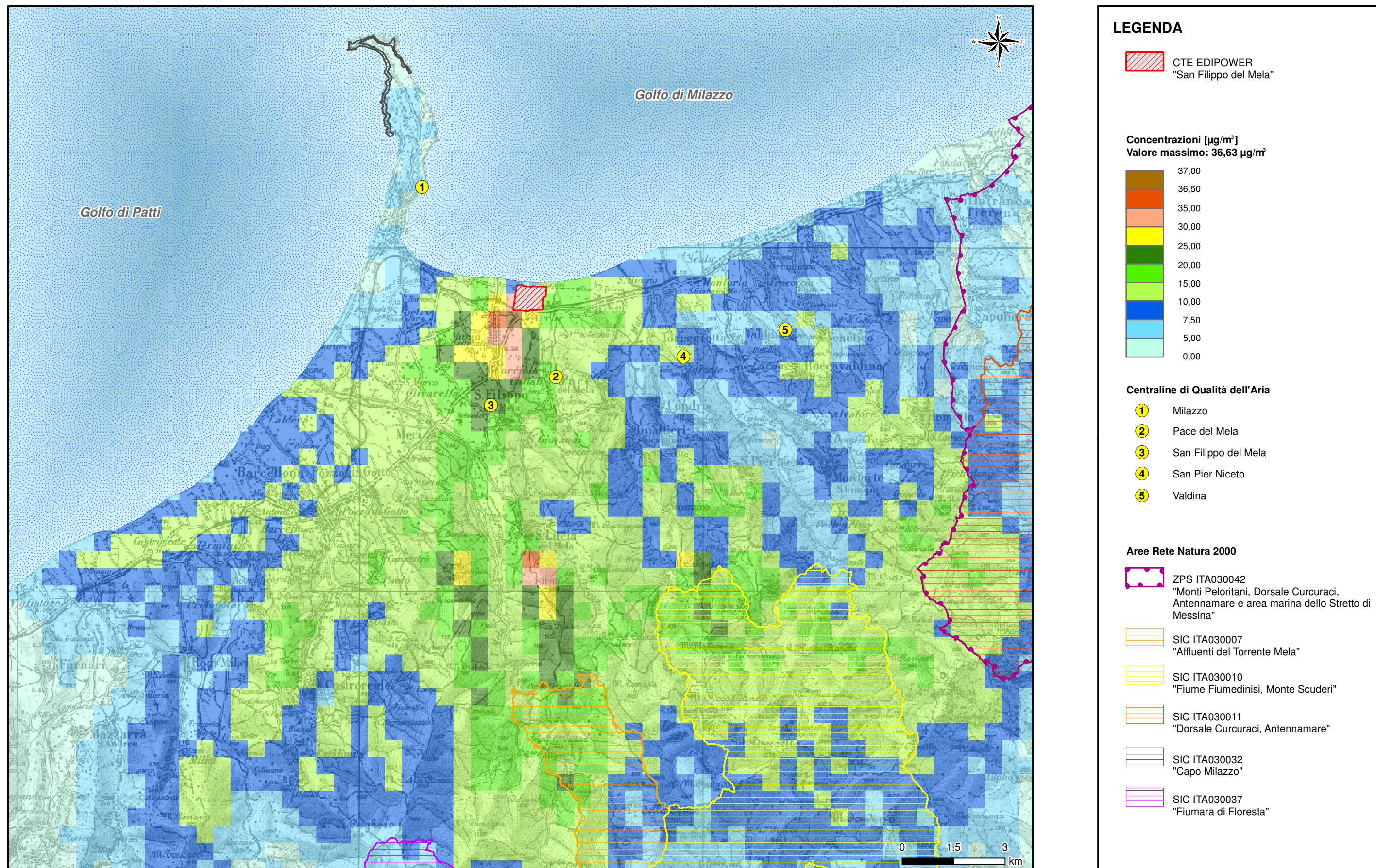
Figura 4.6.1f 99,2° Percentile delle Concentrazioni Medie Giornaliere di SO 2 - Scenario Attuale Autorizzato
