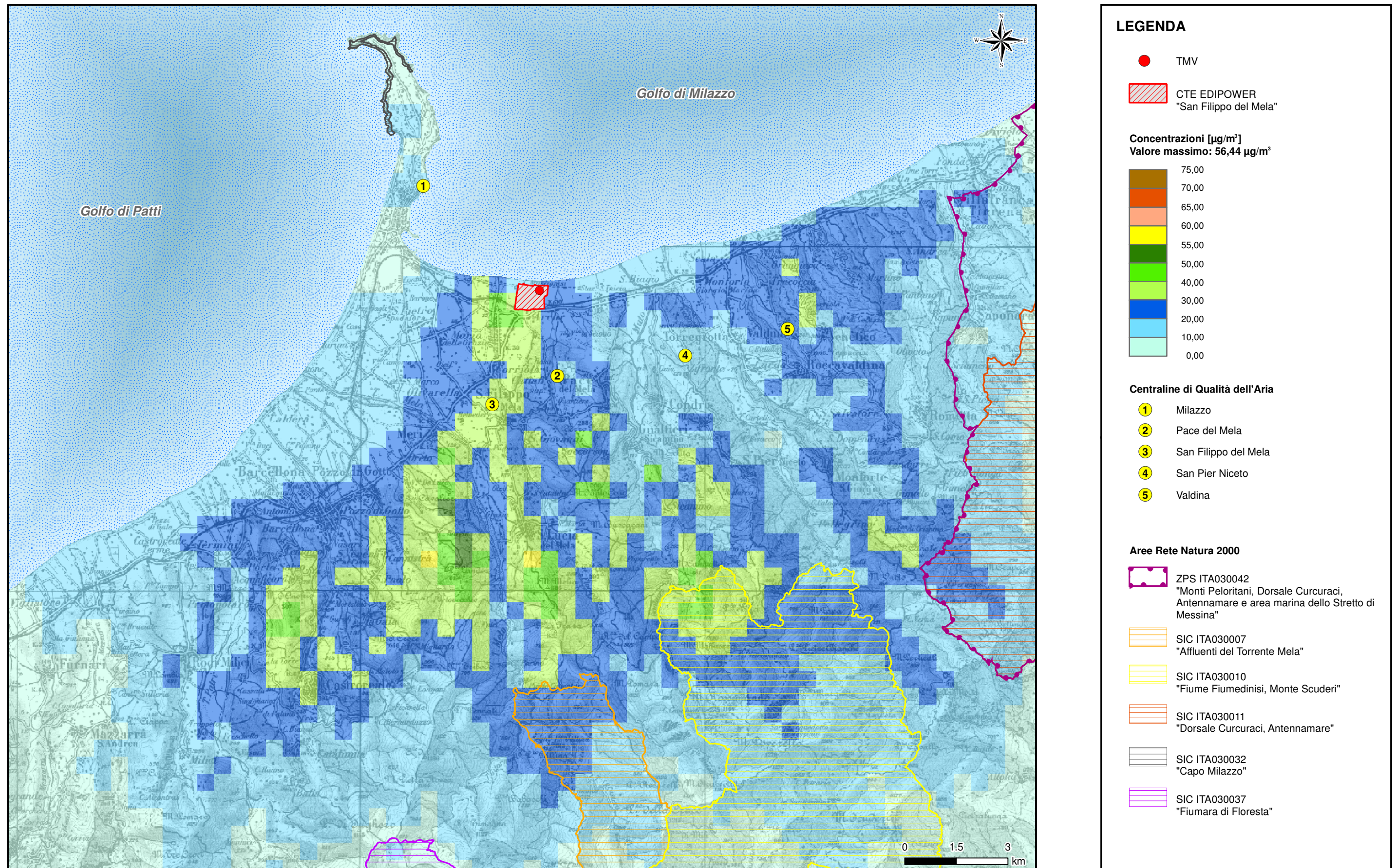
Figura 4.6.2.1a 99,8° Percentile delle Concentrazioni Medie Orarie di NOx - Scenario Futuro
