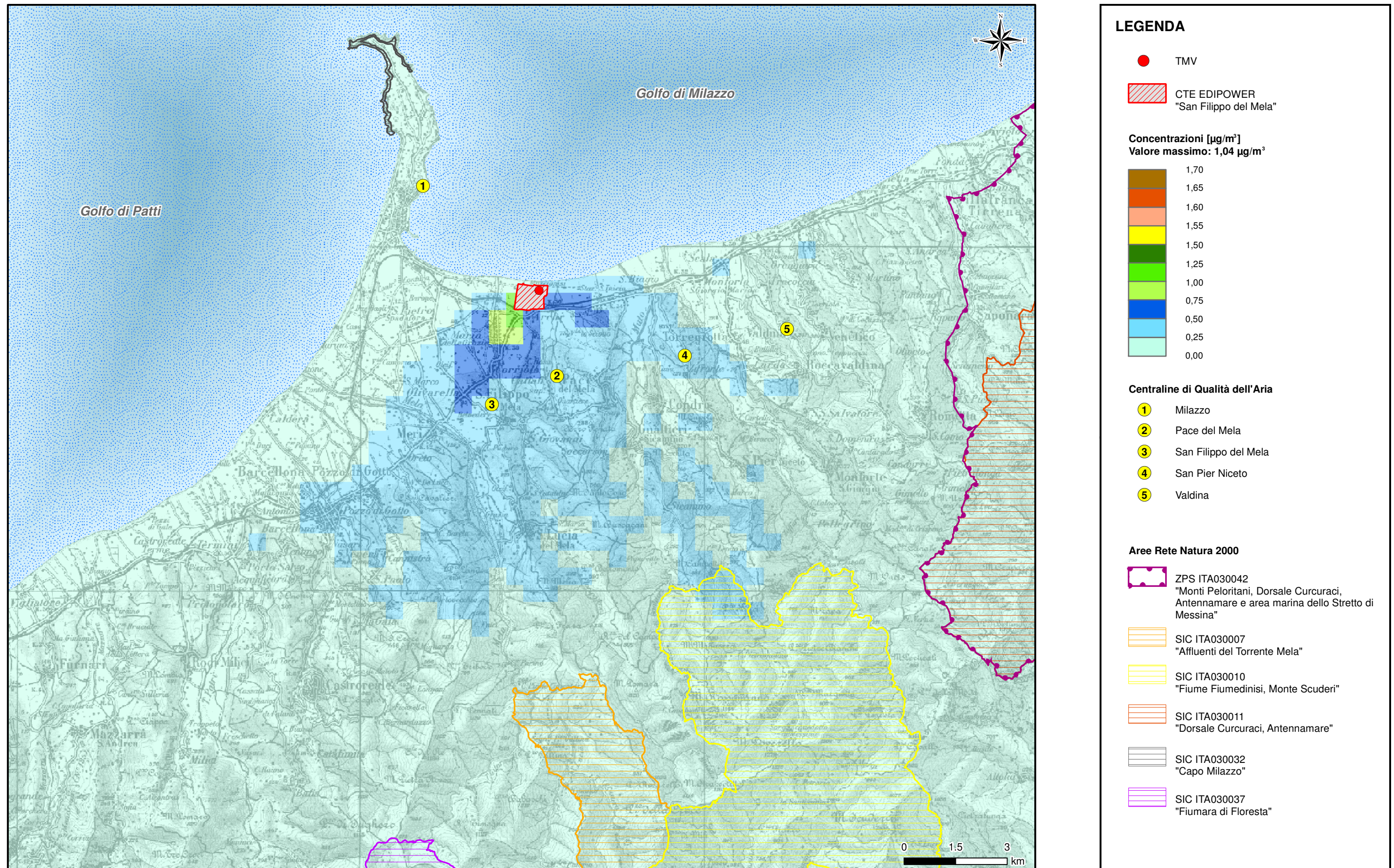
Figura 4.6.2.1c 90,4° Percentile delle Concentrazioni Medie Giornaliere di PTS - Scenario Futuro
