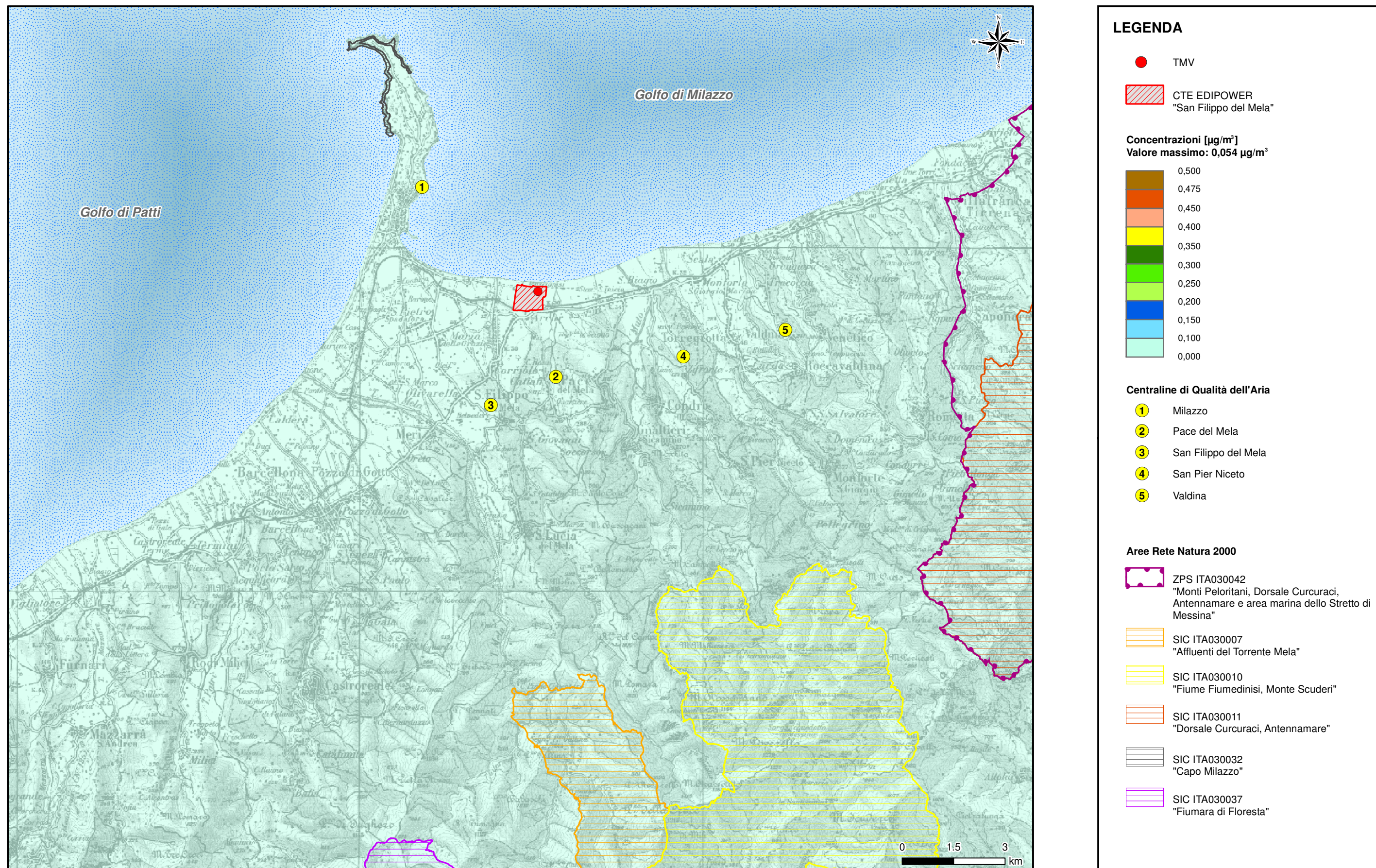
Figura 4.6.2.1d Concentrazione Media Annua di PTS - Scenario Futuro
