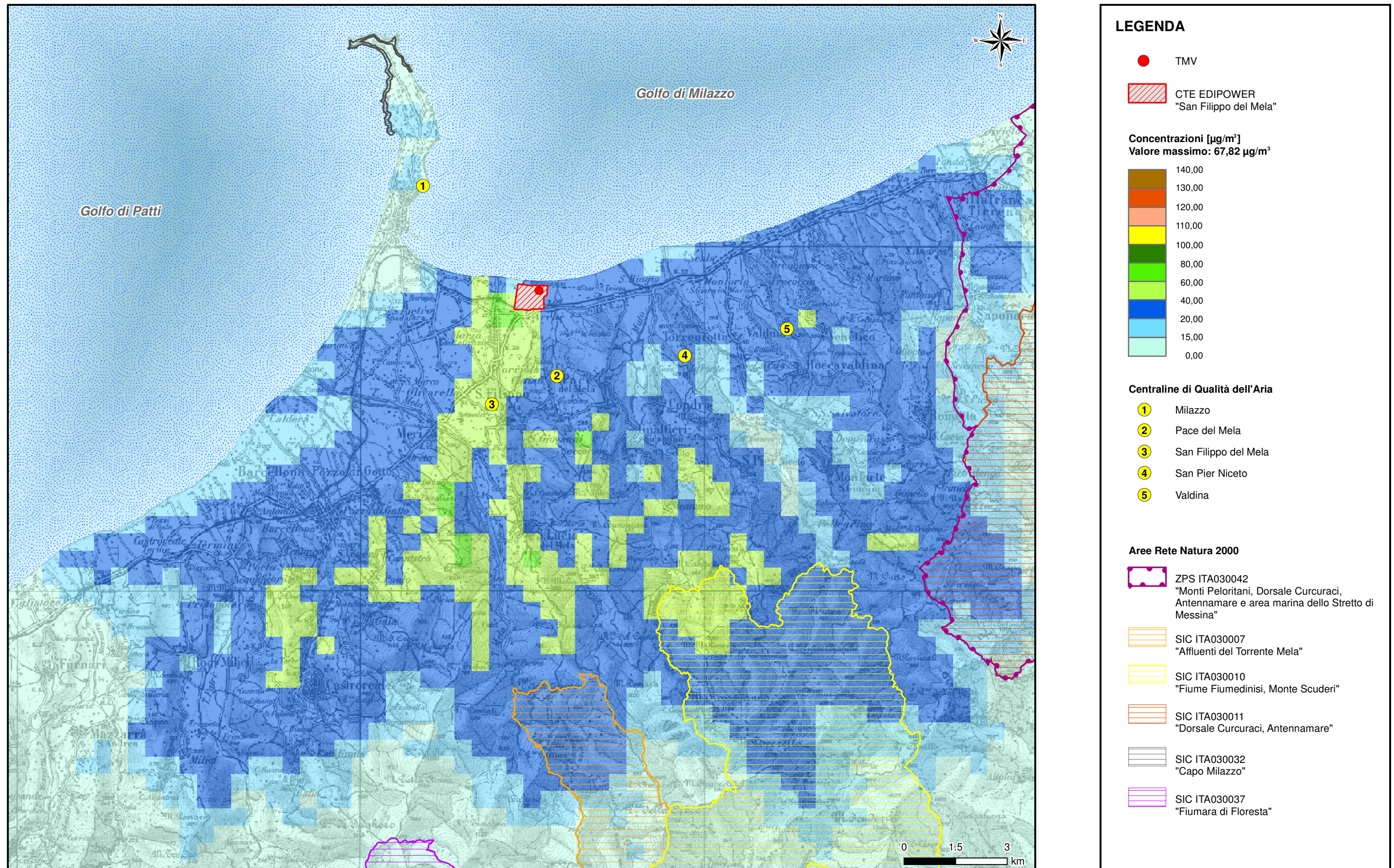
Figura 4.6.2.1e 99,73° Percentile delle Concentrazioni Medie Orarie di SO 2 - Scenario Futuro
