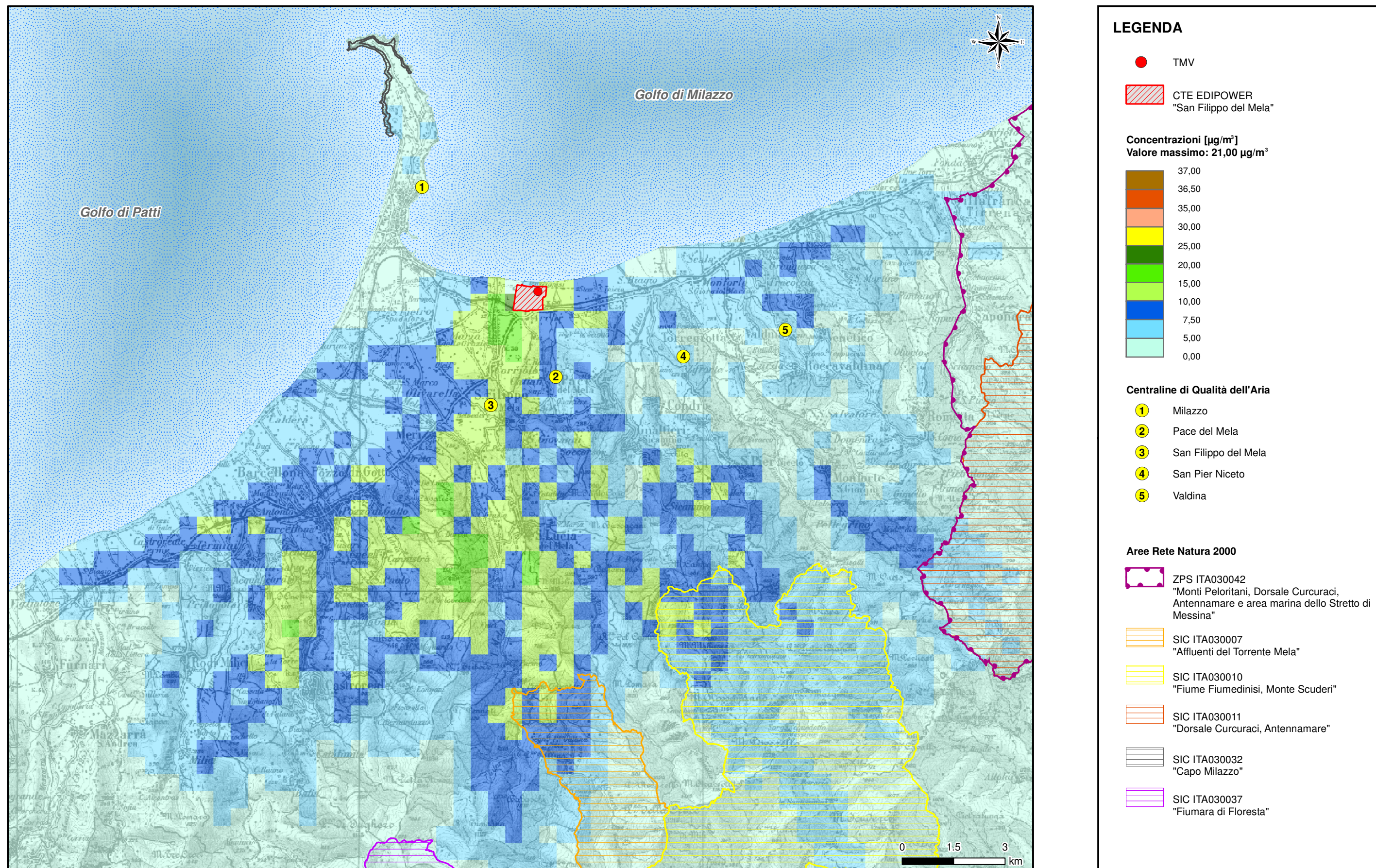
Figura 4.6.2.1f 99,2° Percentile delle Concentrazioni Medie Giornaliere di SO 2 - Scenario Futuro
