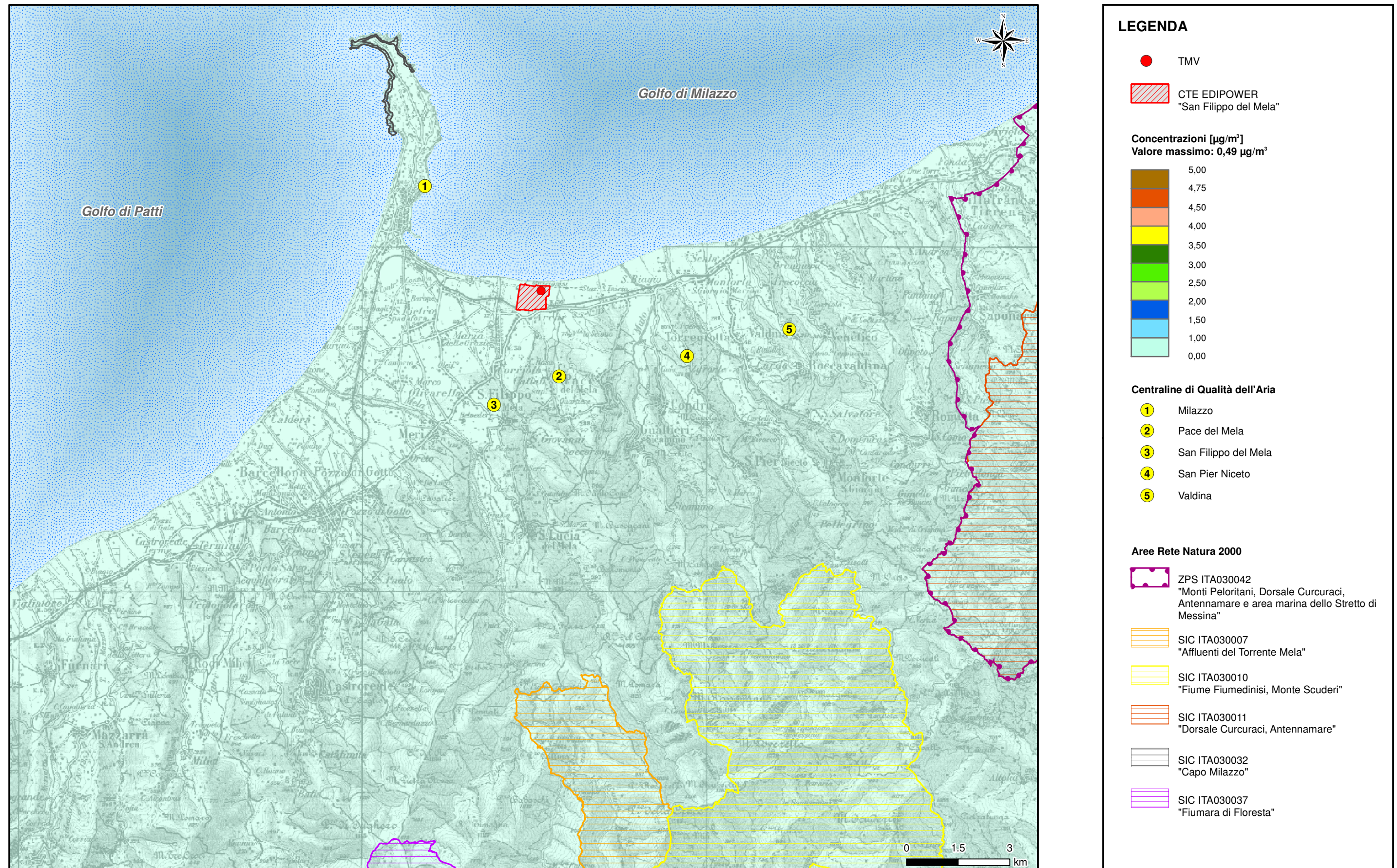
Figura 4.6.2.1g Concentrazione Media Annua di SO 2 - Scenario Futuro
