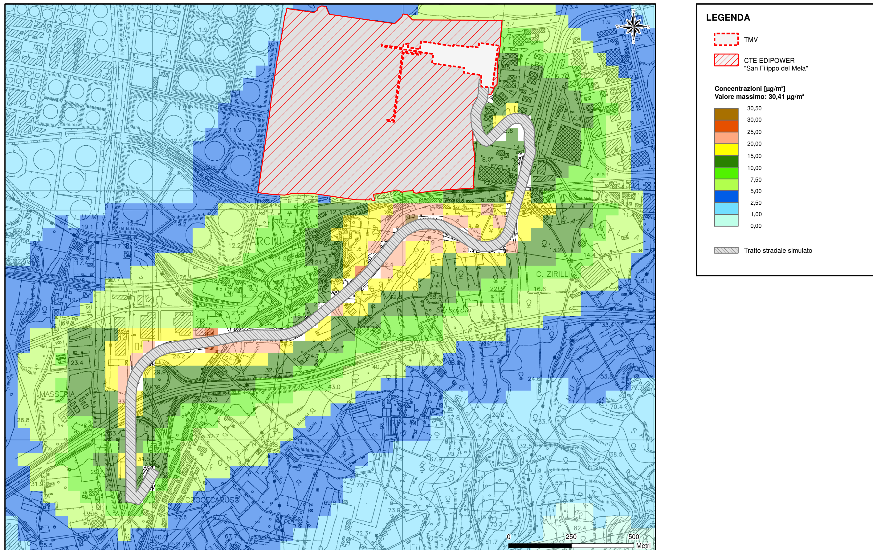
Figura 4.6.2.2a 99,8° Percentile delle Concentrazioni Medie Orarie di NOx emesso dal traffico indotto dal TMV - Scenario Futuro
