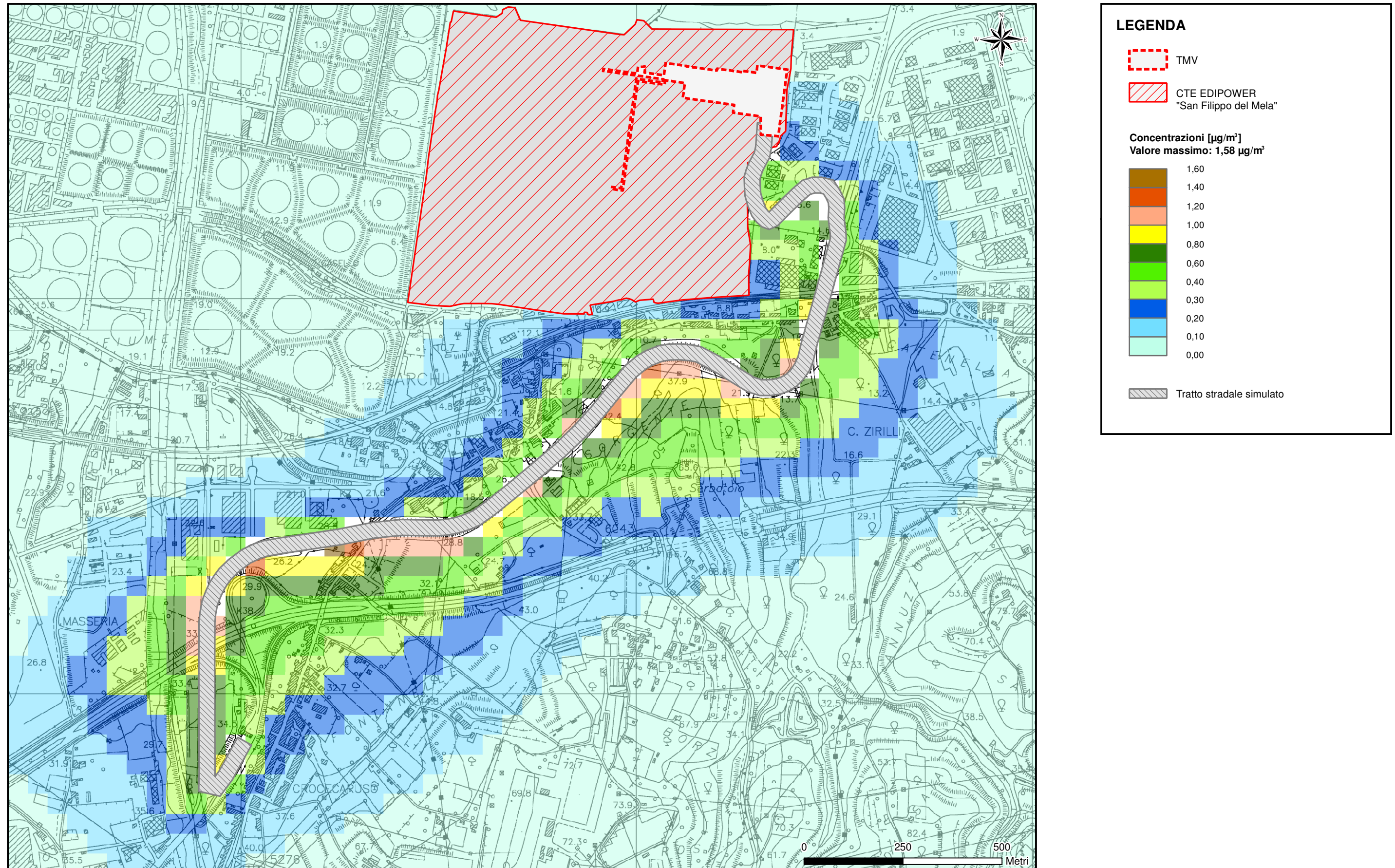
Figura 4.6.2.2b Concentrazione Media Annua di NOx emesso dal traffico indotto dal TMV - Scenario Futuro
