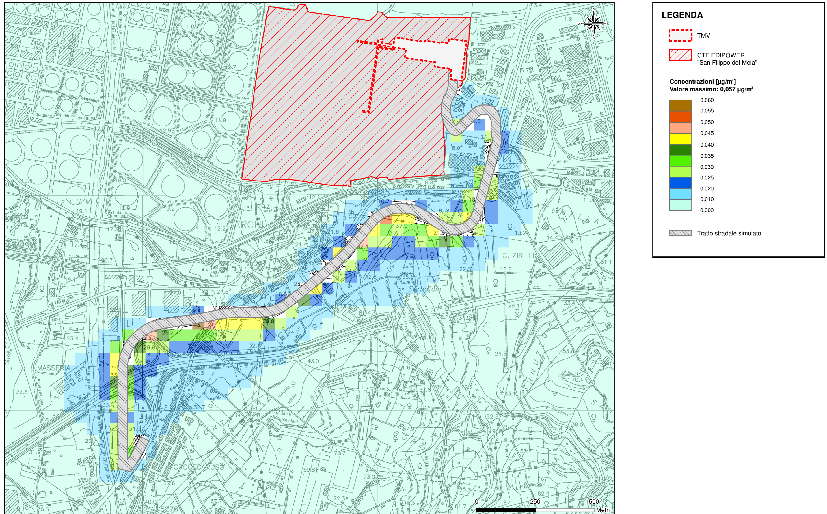
Figura 4.6.2.2d Concentrazione Media Annua di PM10 emesso dal traffico indotto dal TMV - Scenario Futuro
