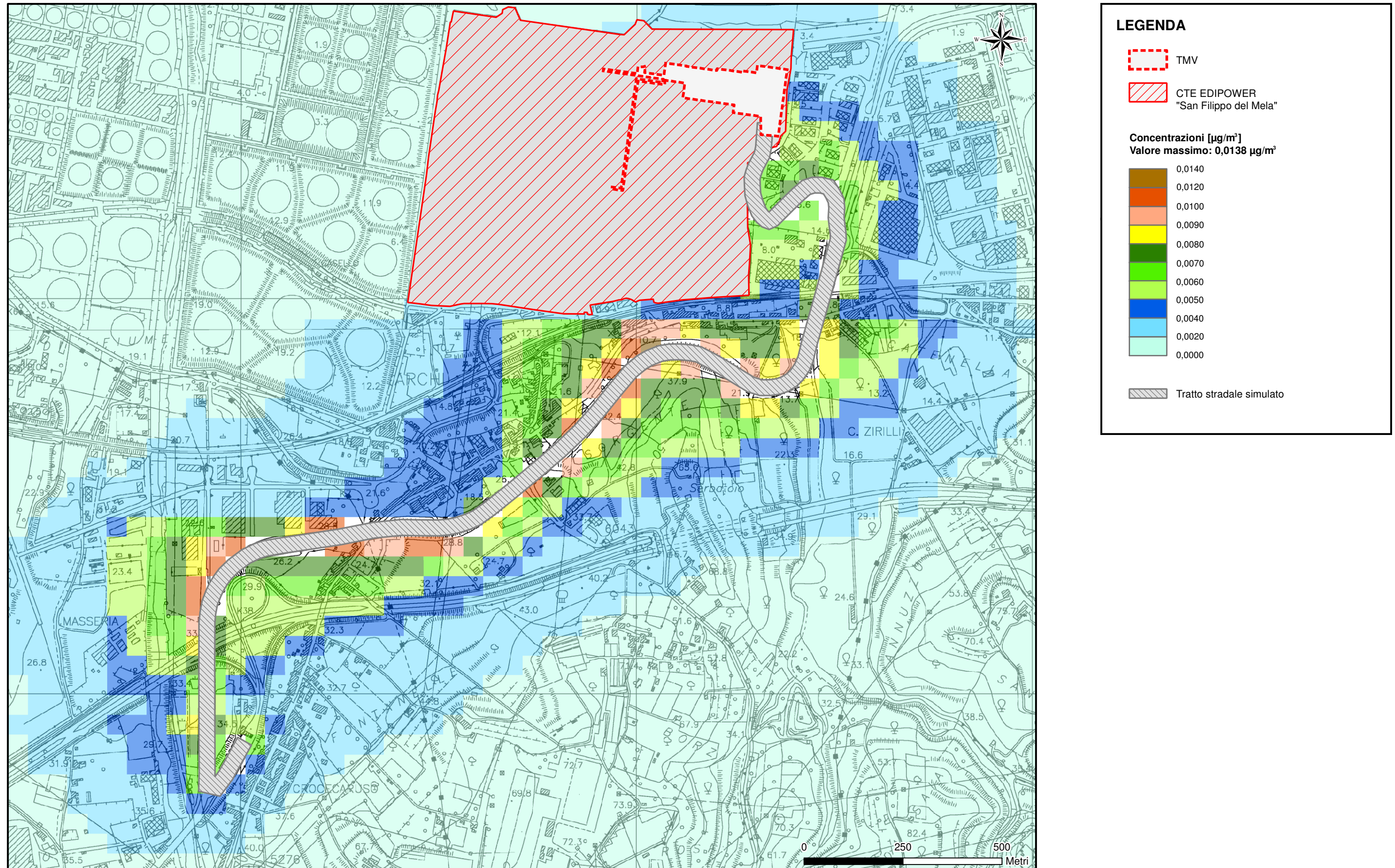
Figura 4.6.2.f 99,73° Percentile delle Concentrazioni Medie Orarie di SO 2 emesso dal traffico indotto dal TMV - Scenario Futuro
