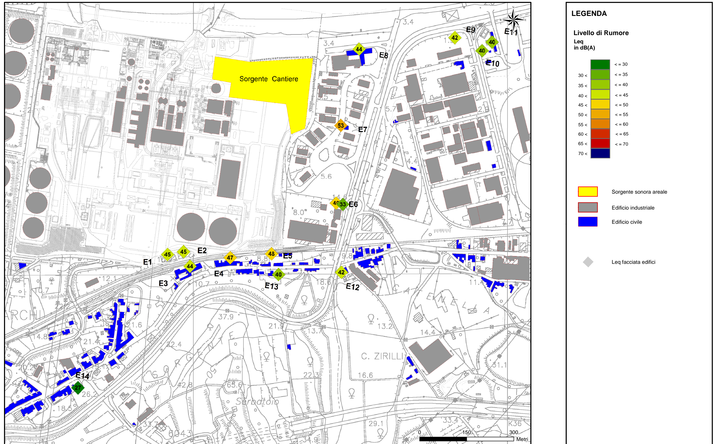
Figura 5.2a Livello Equivalente dBA ai Ricettori Limitrofi al TMV nella Fase di Cantiere
