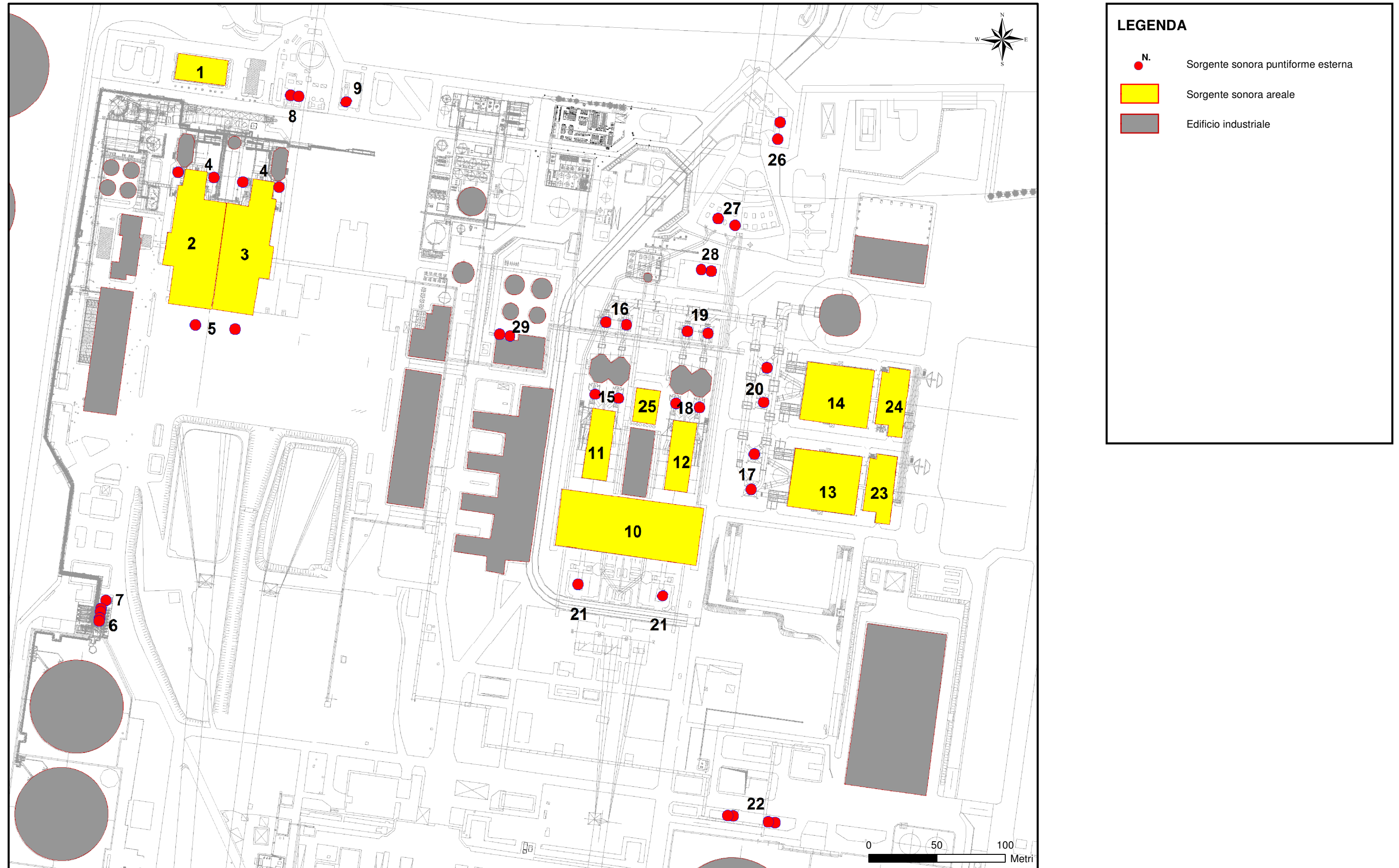
Figura 5.3.1.1a Ubicazione delle Sorgenti Sonore presenti nella Centrale di San Filippo del Mela nella Situazione Attuale
