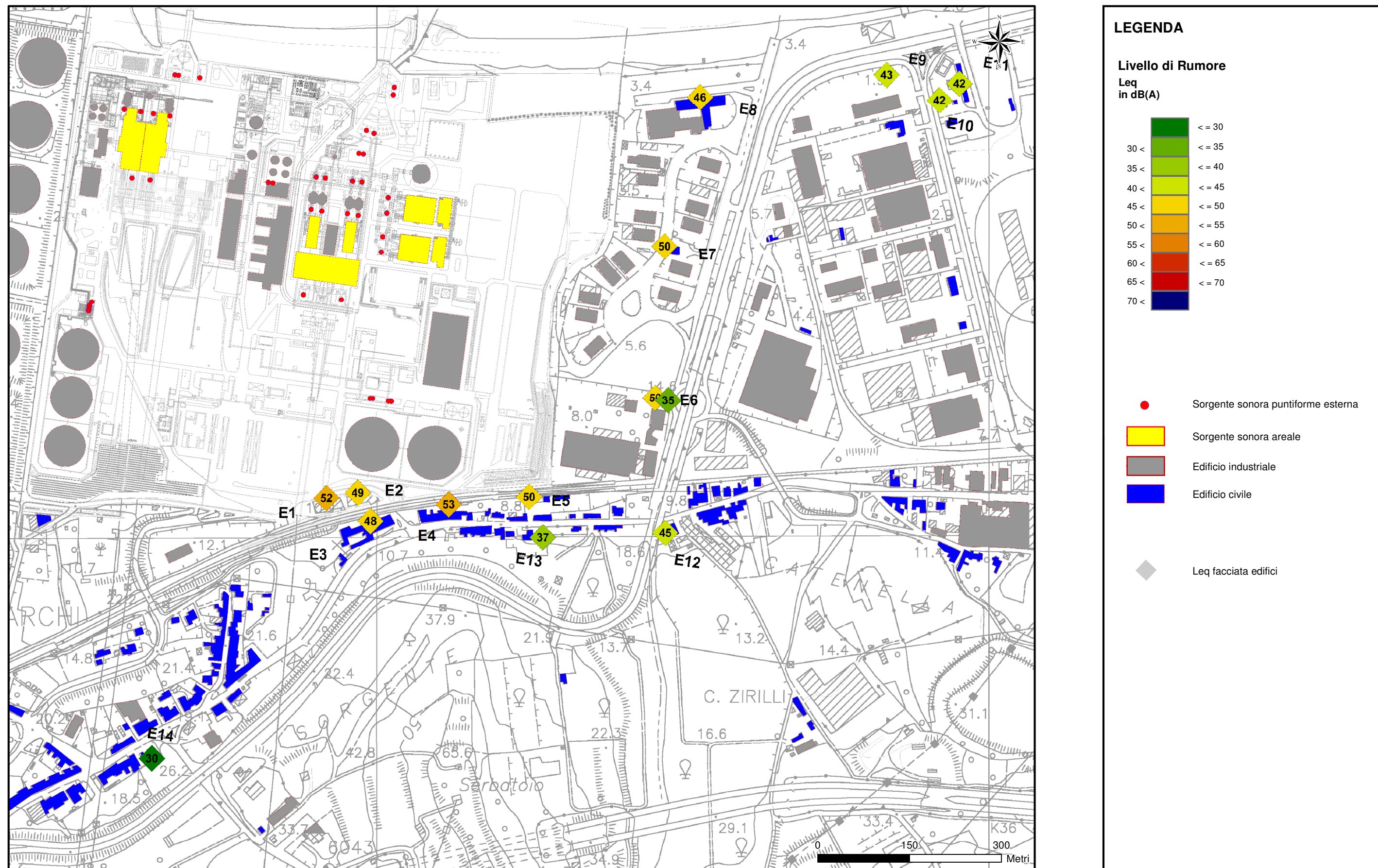
Figura 5.3.1.2a Livello Equivalente Edifici Limitrofi alla Centrale di San Filippo del Mela nella Situazione Attuale nel Periodo Diurno e Notturno
