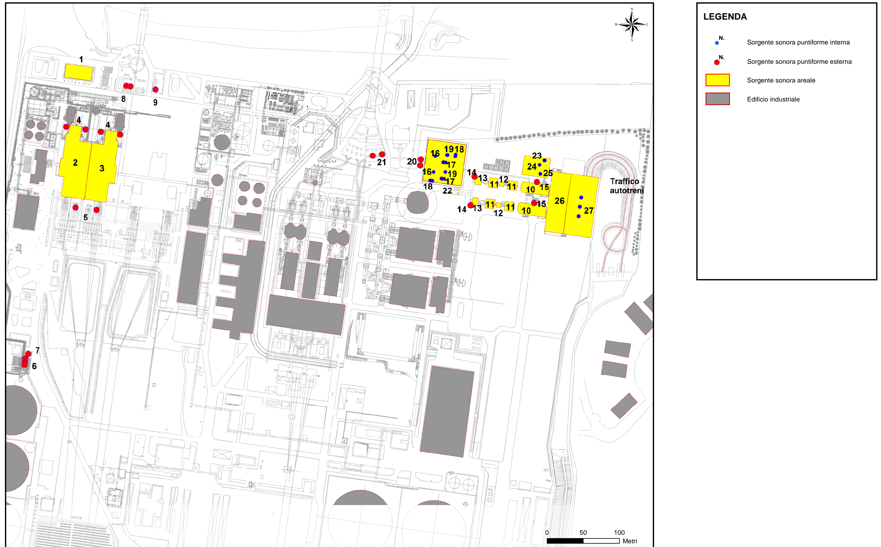
Figura 5.3.2.1a Ubicazione delle Sorgenti Sonore presenti nella Centrale di San Filippo del Mela e nel TMV nella Situazione Futura
