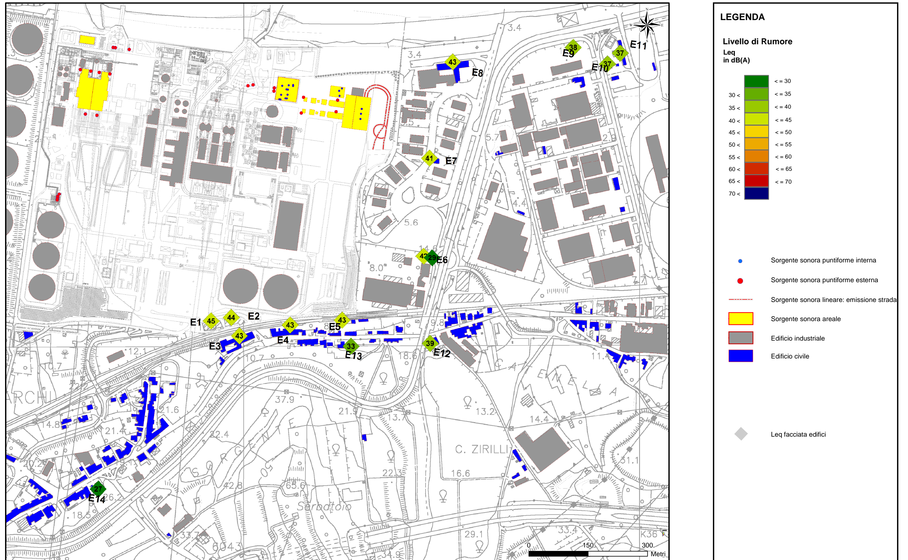
Figura 5.3.2.2a Livello Equivalente Edifici Limitrofi alla Centrale e al TMV di San Filippo del Mela nella Situazione Futura nel Periodo Diurno
