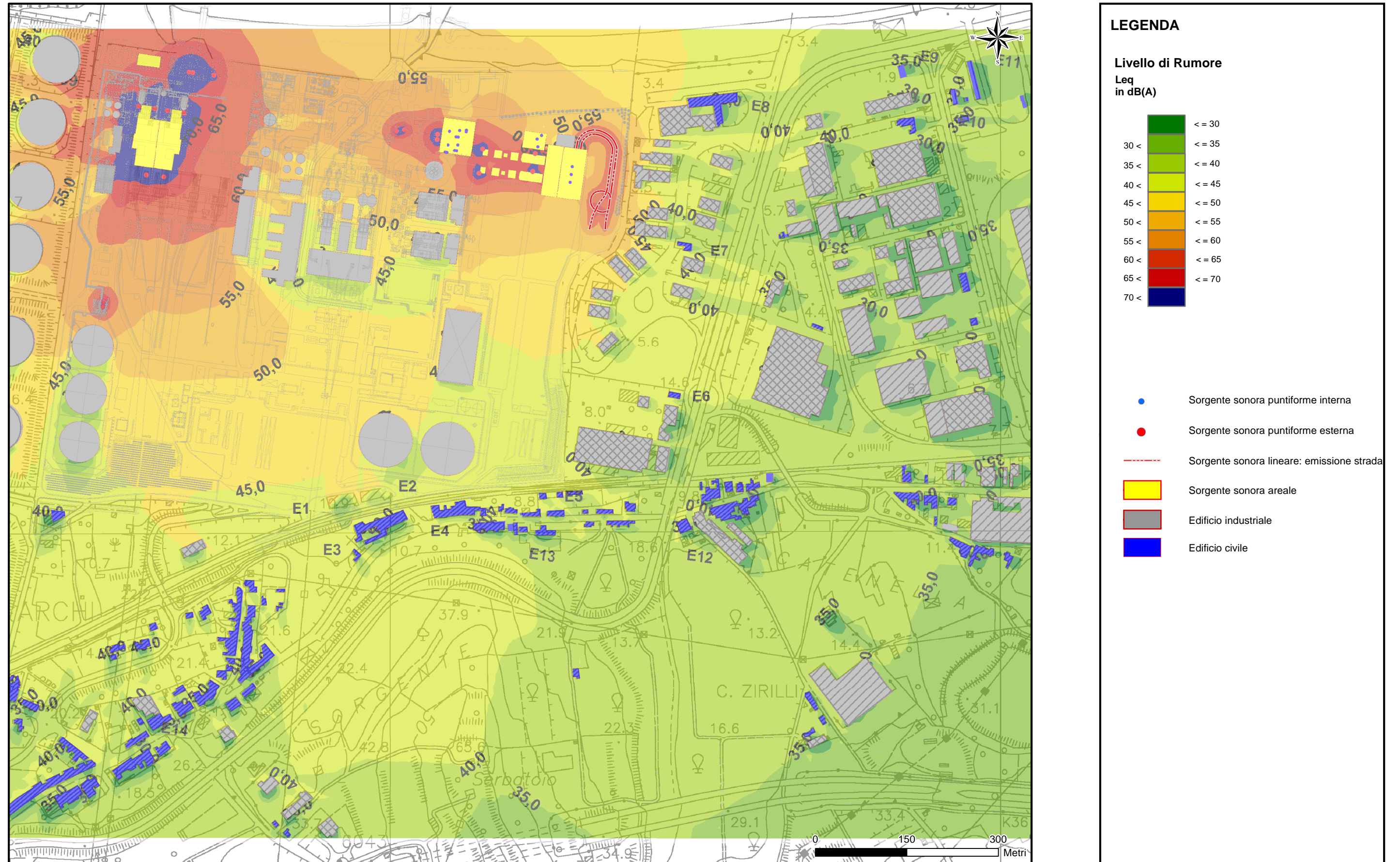
Figura 5.3.2.2c Isofoniche nell'Area Limitrofa alla Centrale e al TMV di San Filippo del Mela nella Situazione Futura nel Periodo Diurno
