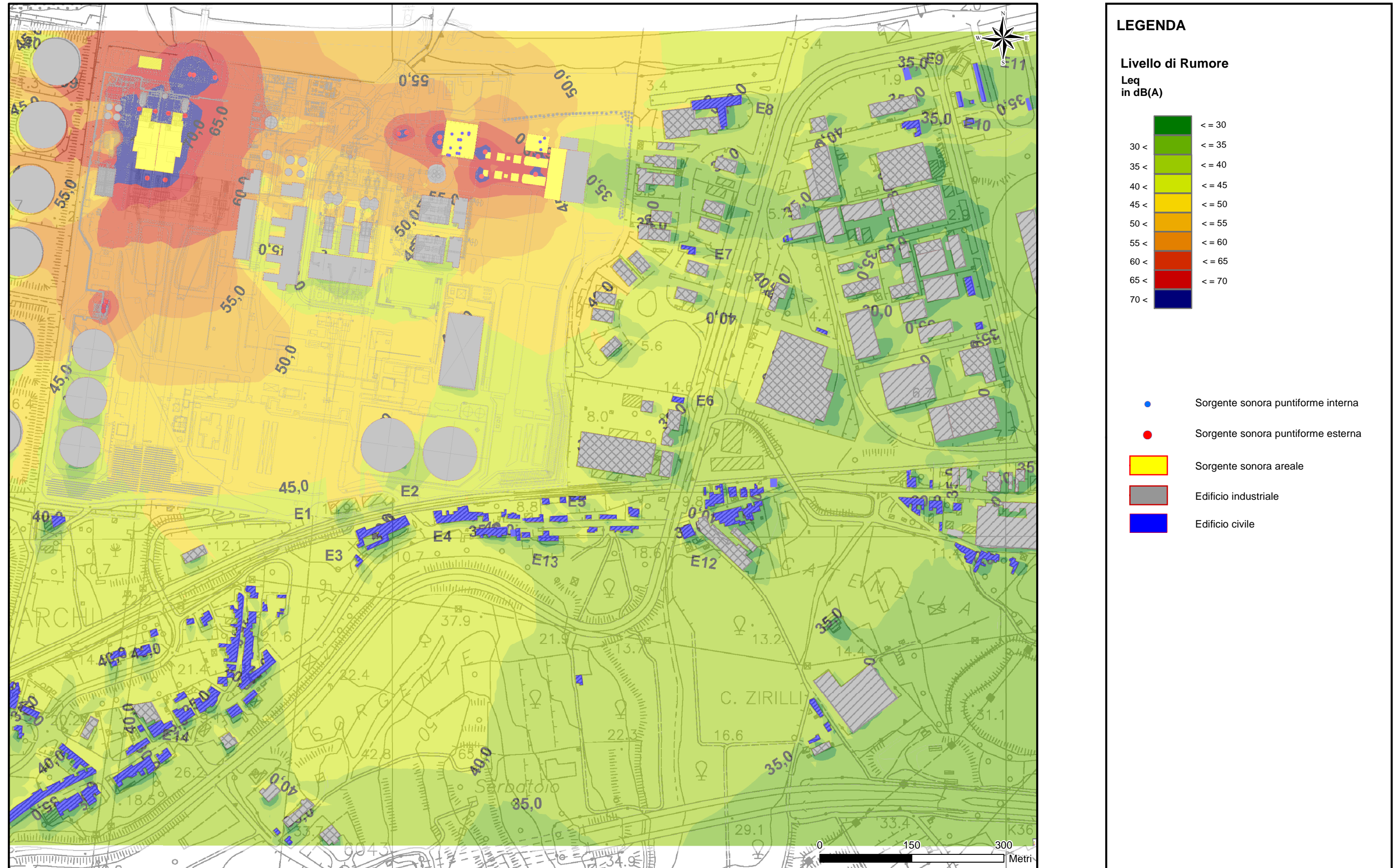
Figura 5.3.2.2d Isofoniche nell'Area Limitrofa alla Centrale e al TMV di San Filippo del Mela nella Situazione Futura nel Periodo Notturno
