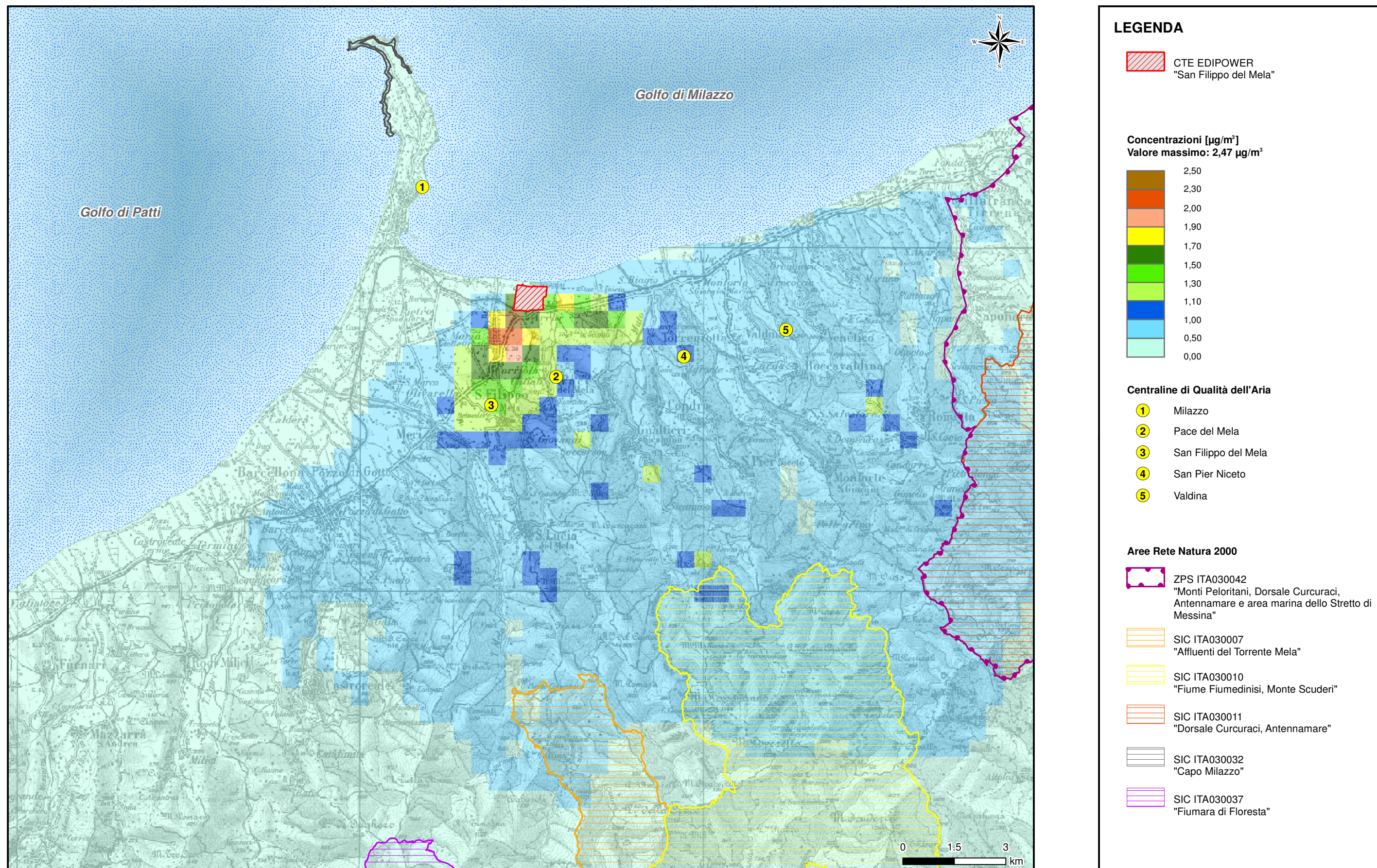
Figura 4.3.1.2a Concentrazione Media Annua di NOx - Scenario Attuale Autorizzato
