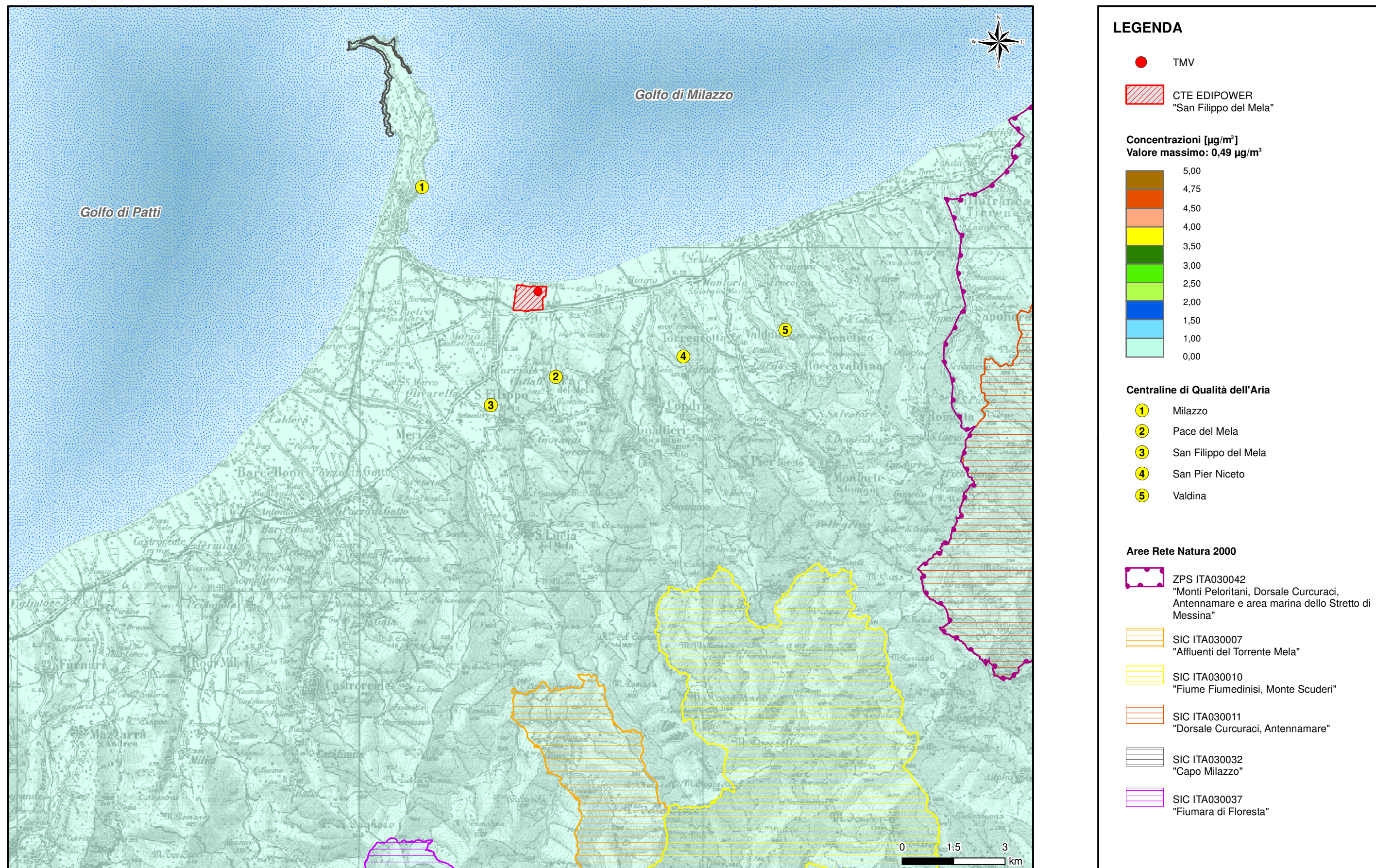
Figura 4.3.1.2f Concentrazione Media Annua di SO 2 - Scenario Futuro
