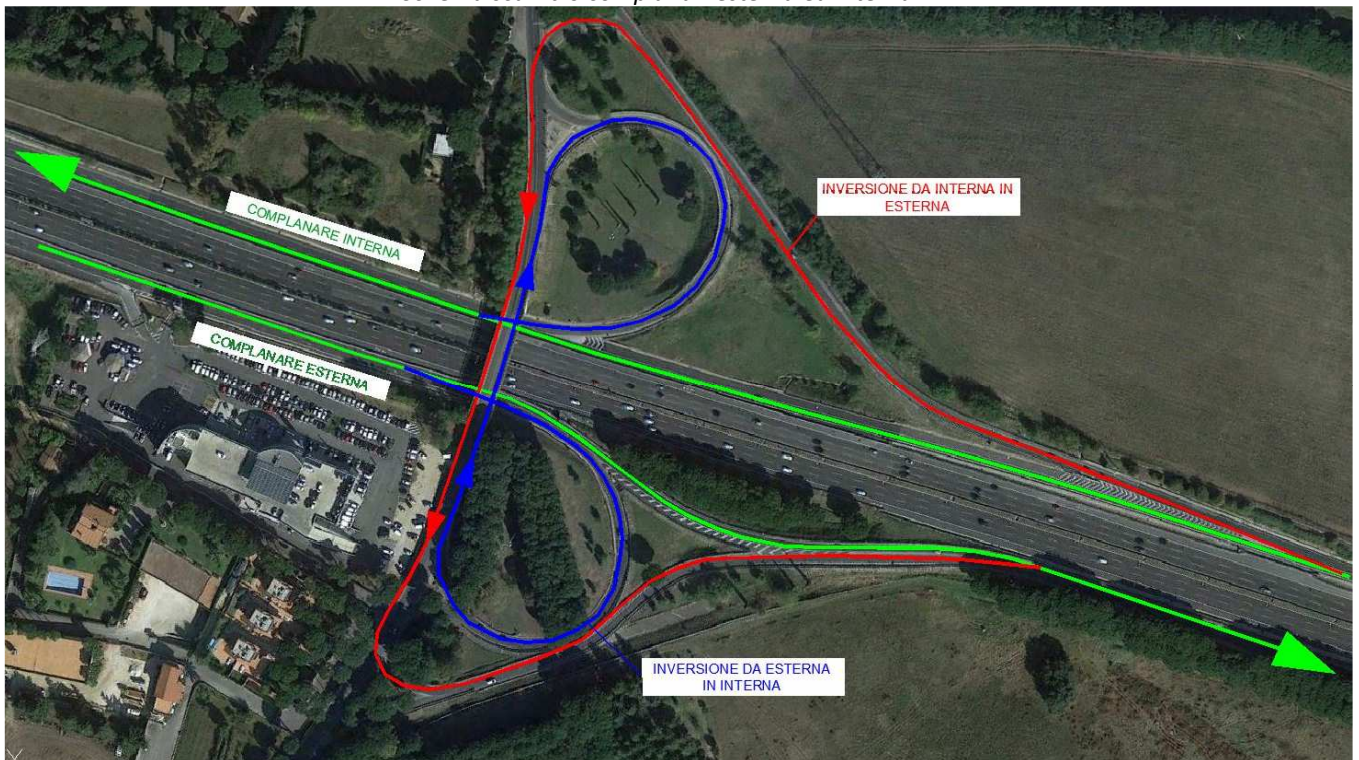
Schema scambio complanari esterna ed interna
