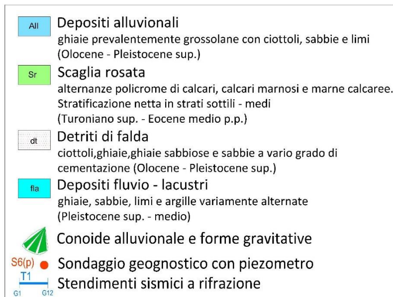
Figura 4 – Stralcio della Carta geologica dell'area
