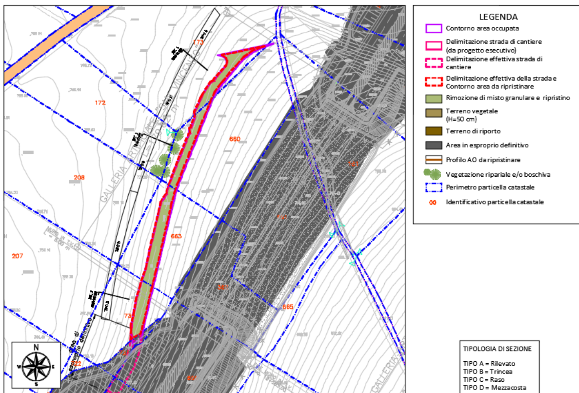
Figura 9 – Sistemazione paesaggistica della pista
