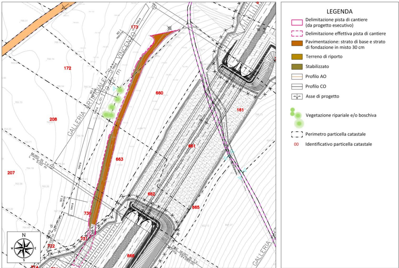
Figura 1 – Planimetria stato di fatto
