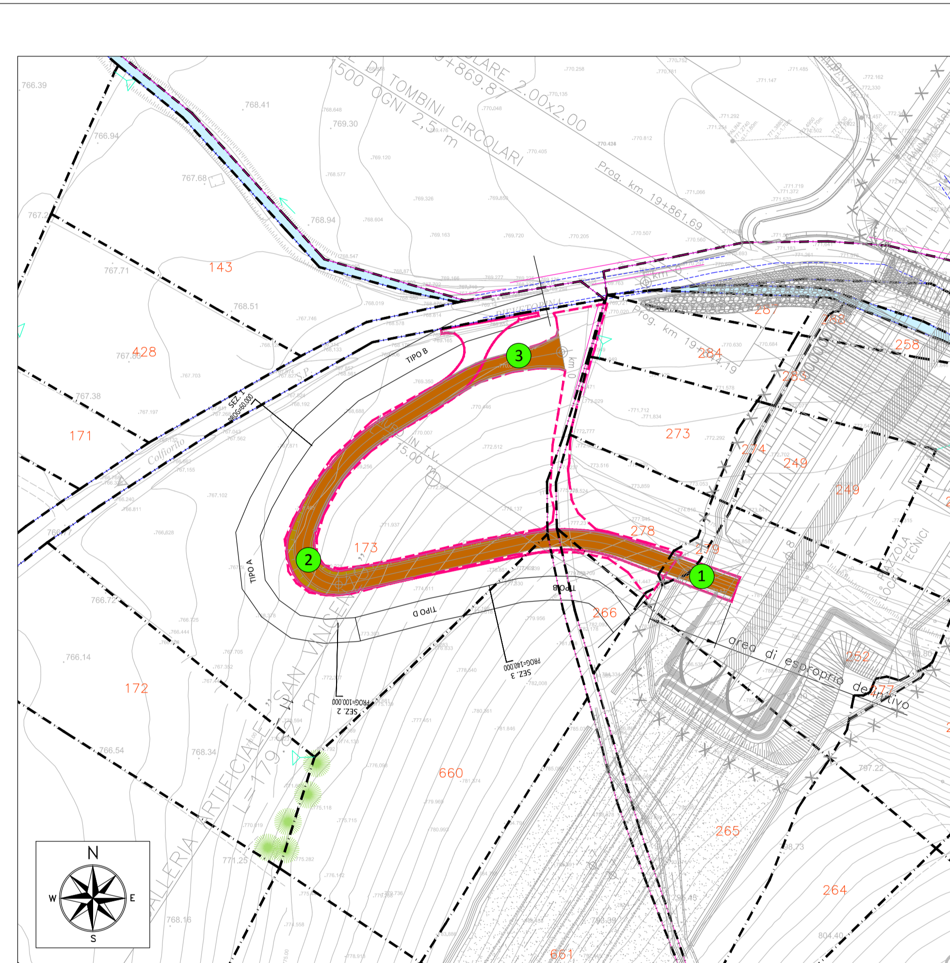
PLANIMETRIA STATO DI FATTO - SCALA 1:1000
