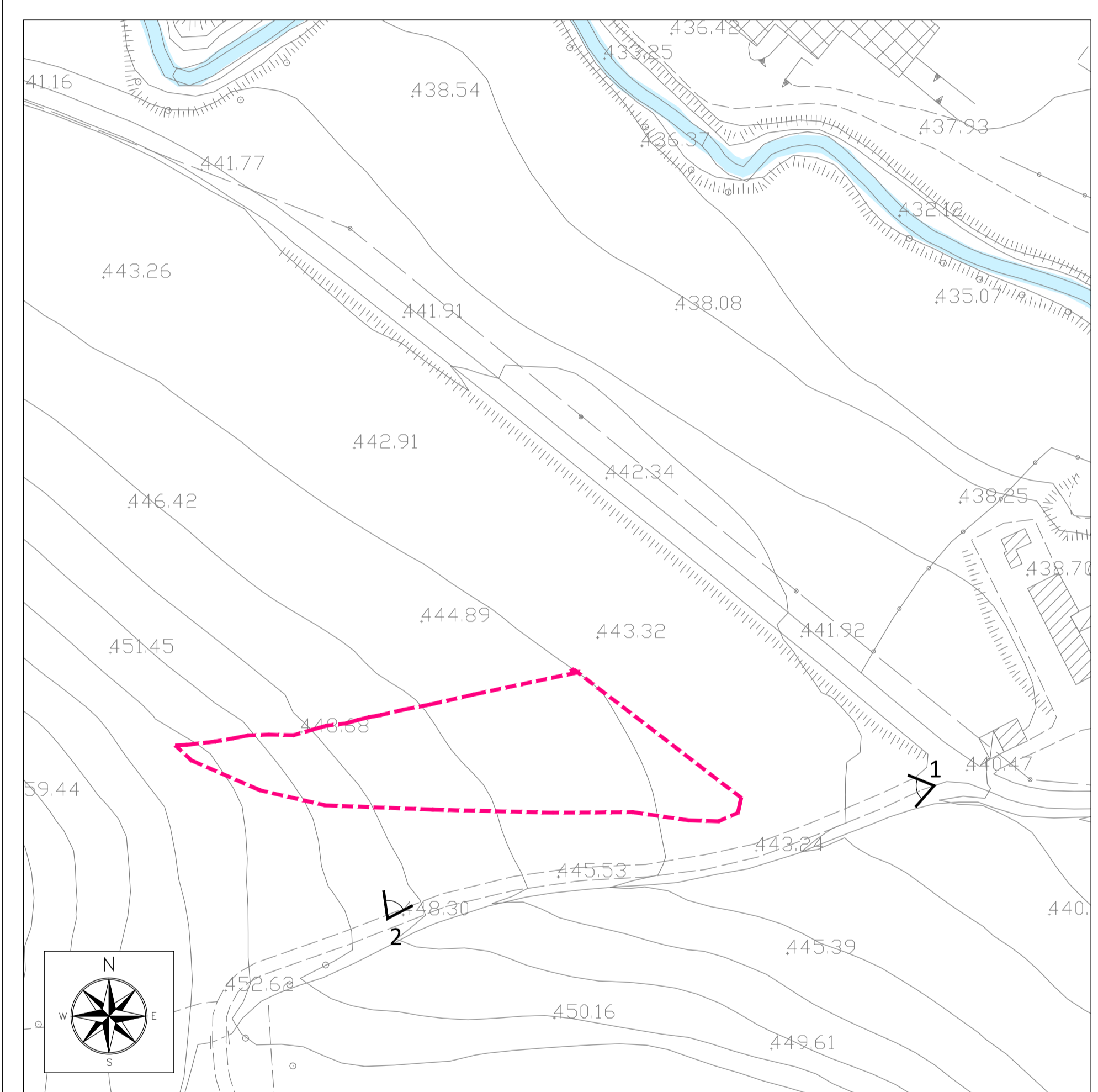
PLANIMETRIA STATO ANTE OPERAM - SCALA 1:1000
