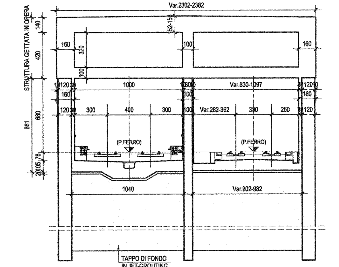
SEZIONE TIPO "H"-Scala 1:200
