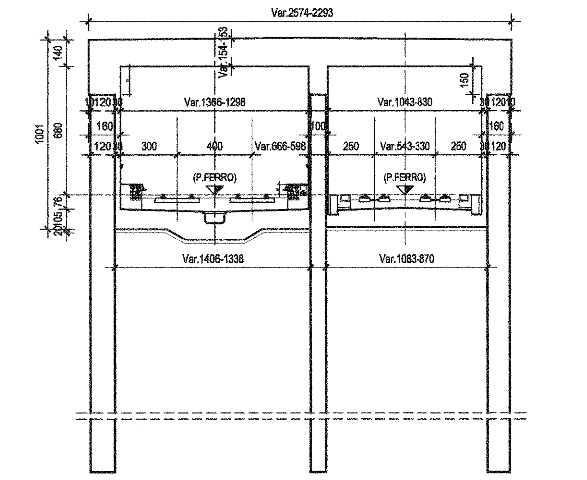
SEZIONE TIPO *P*-Scala 1:200
