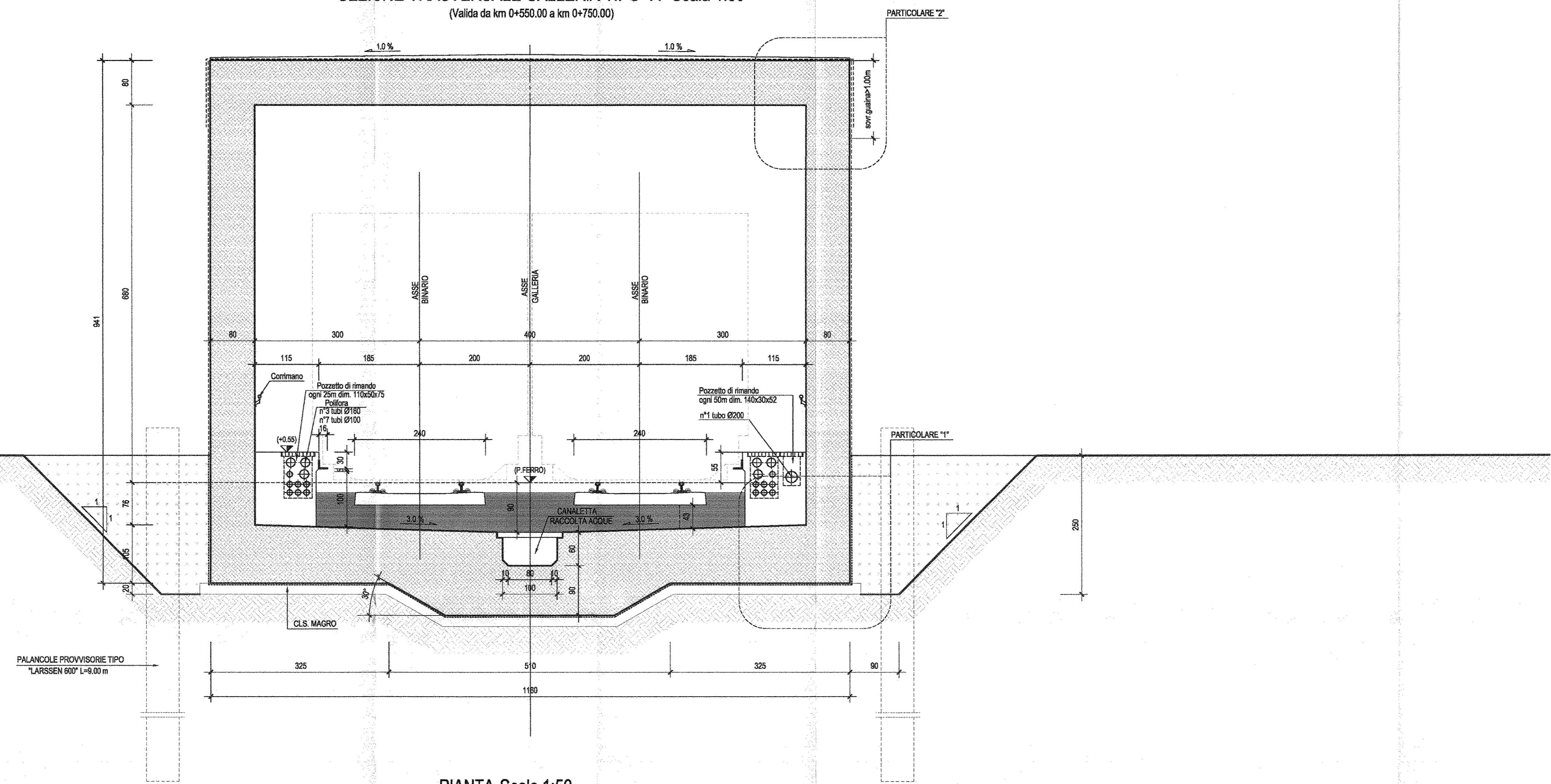
PIANTA-Scala 1:50
