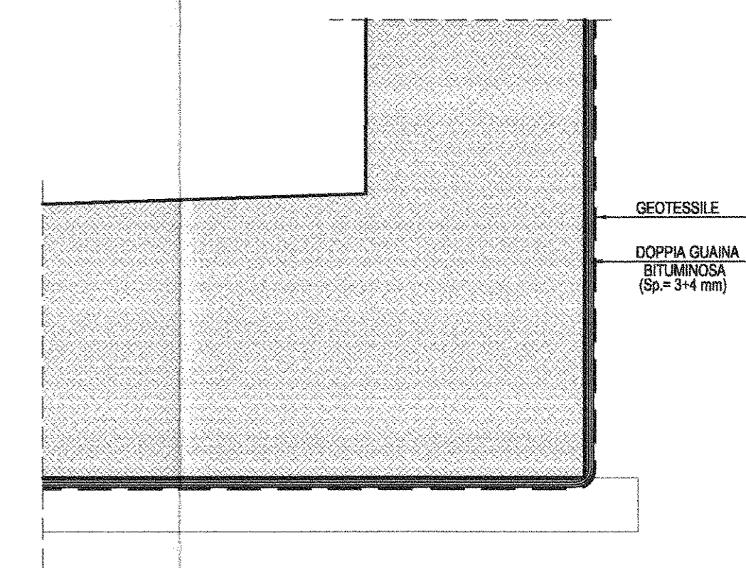
PARTICOLARE "2"-Scala 1:20
