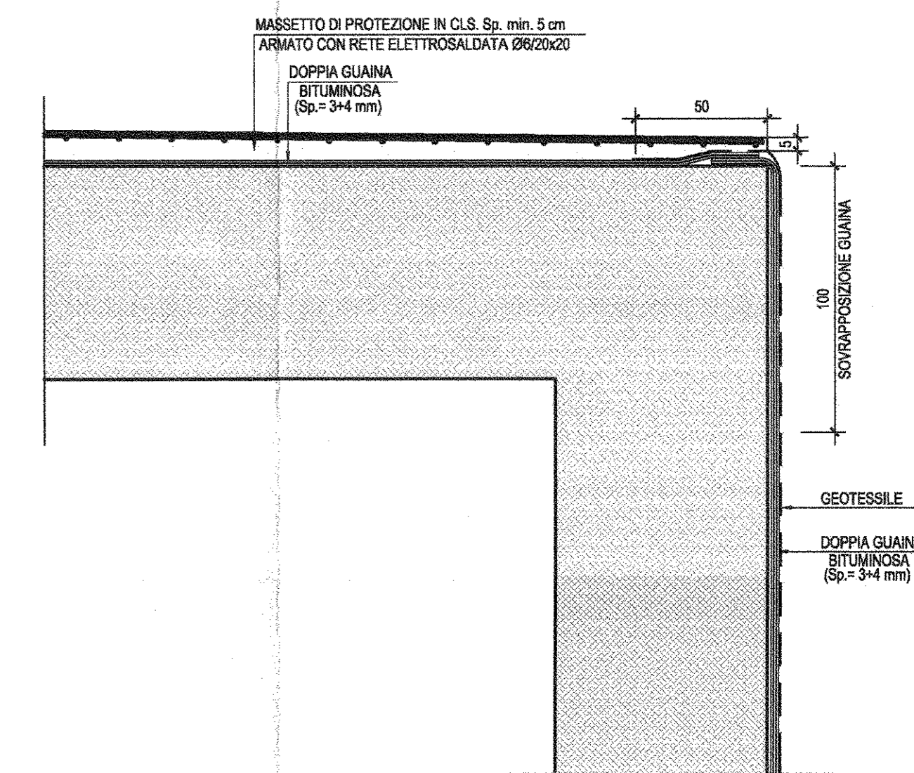
PARTICOLARE "2"-Scala 1:20
