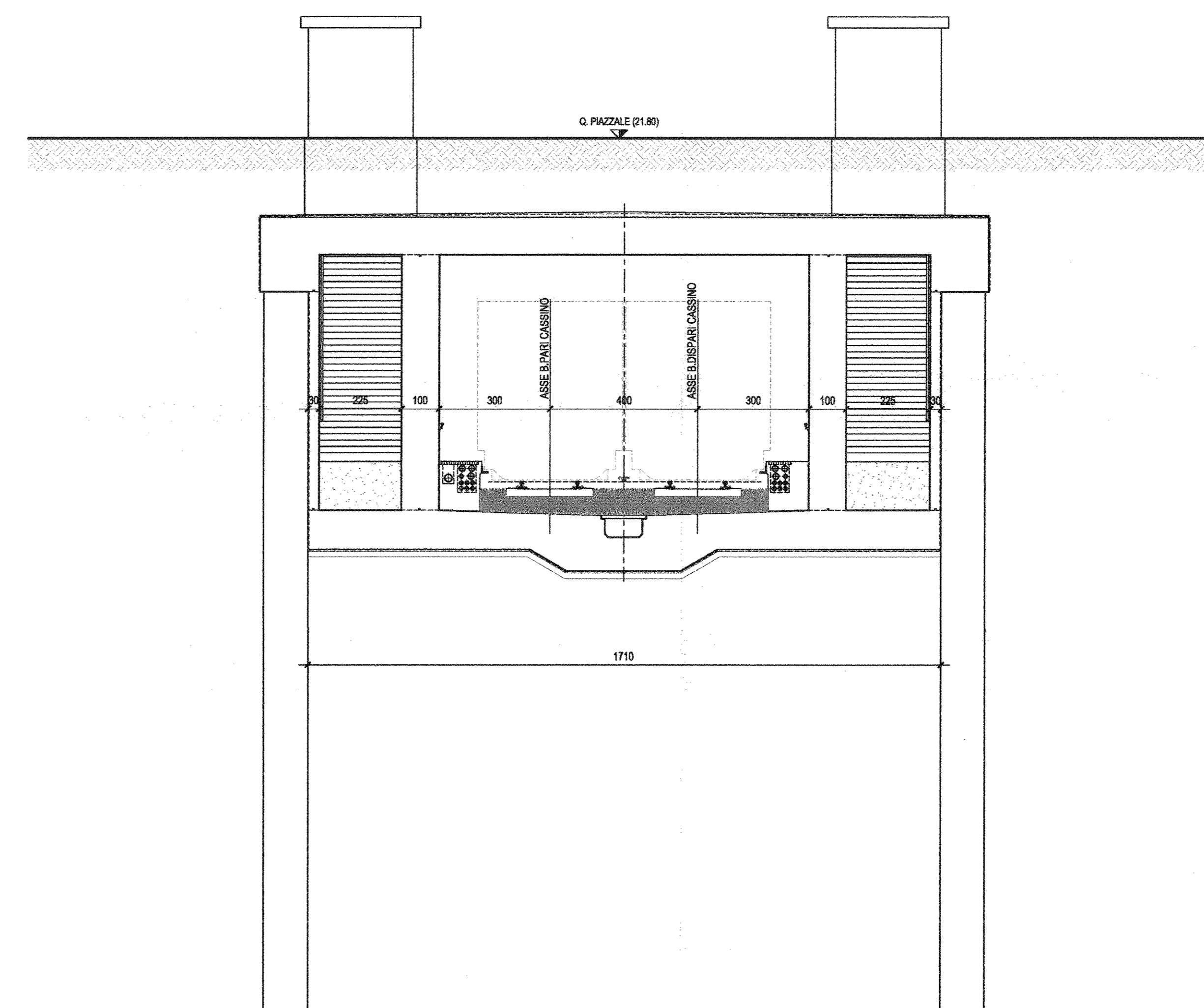
SEZIONE B-B-Scala 1:100
