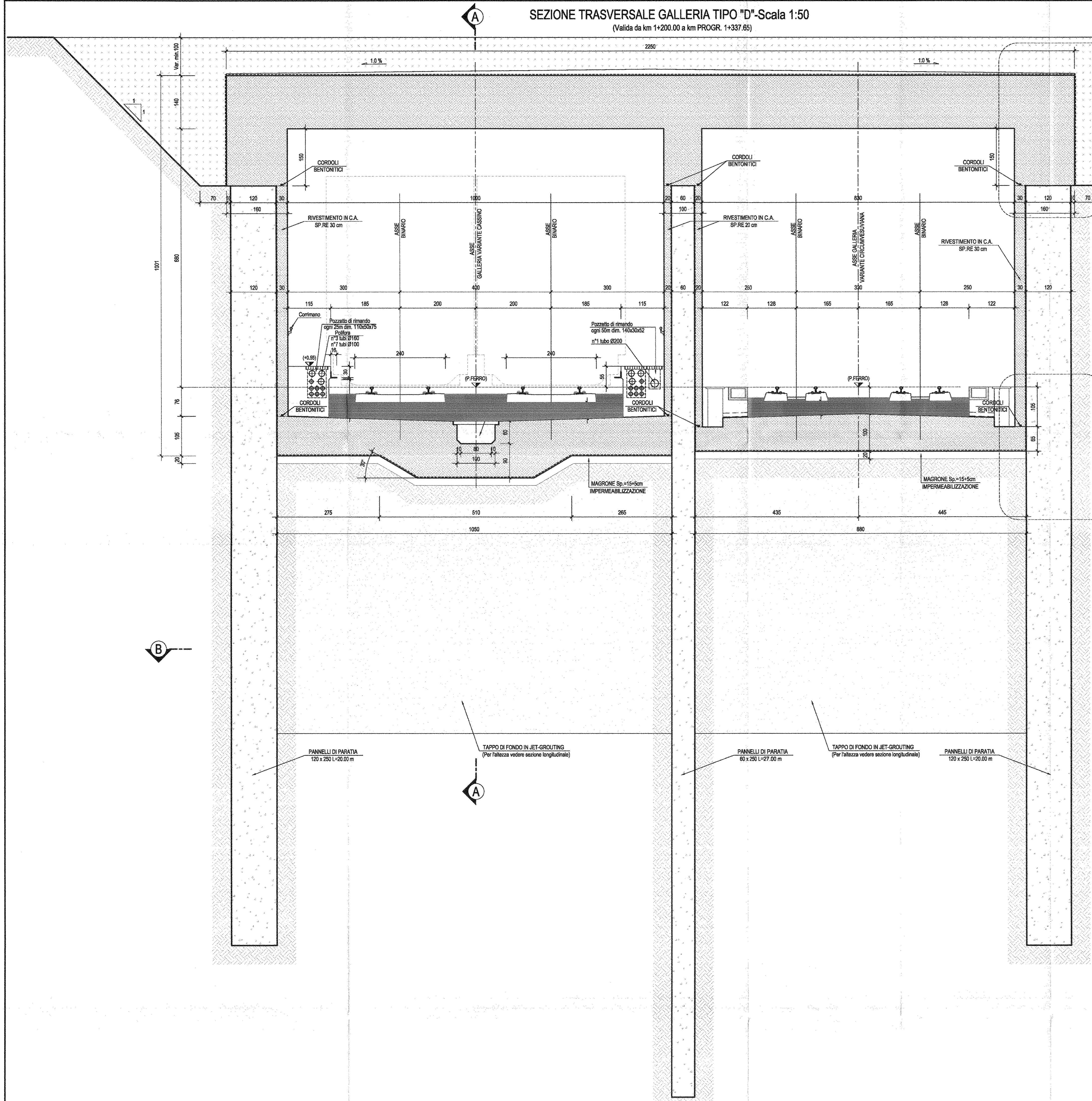
SEZIONE B-B-Scala 1:50
