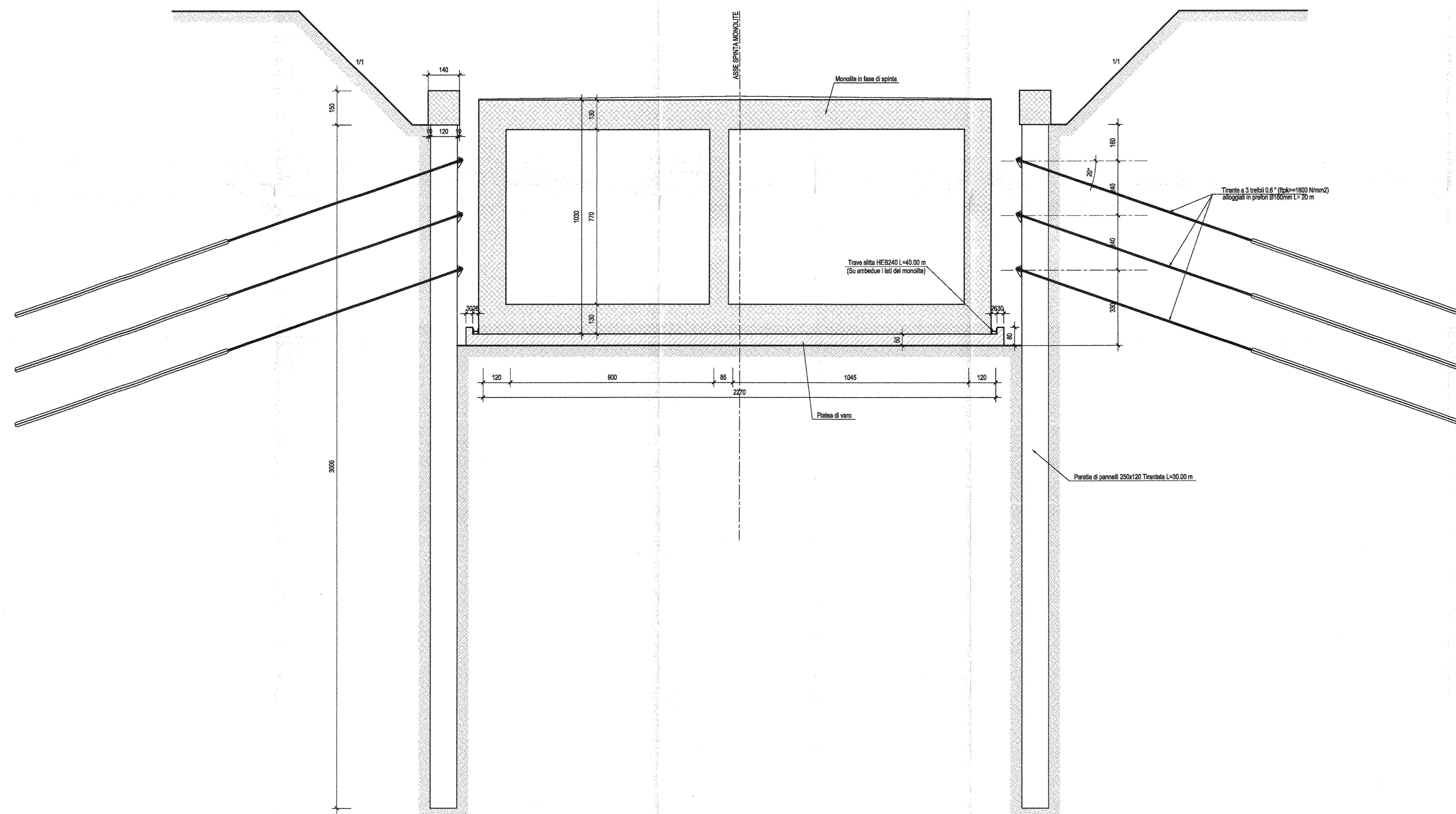
SEZIONE A-A-Scala 1:100
