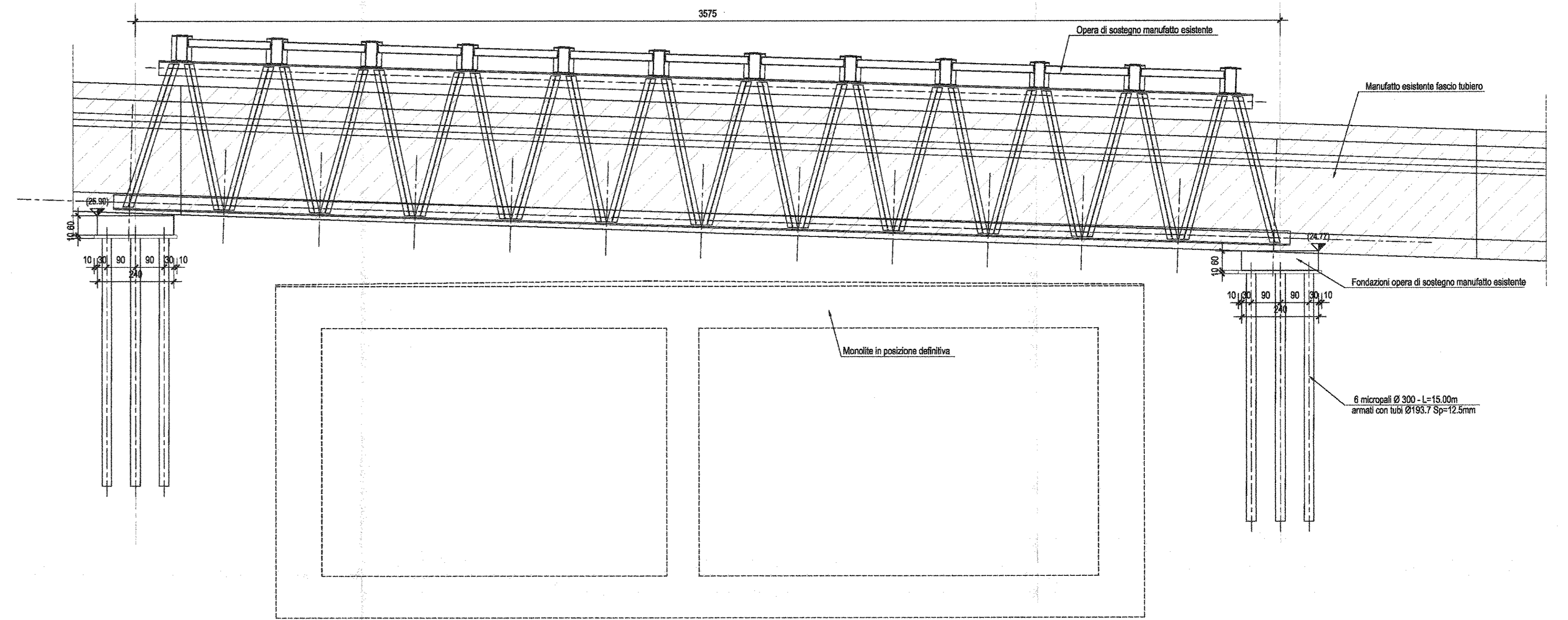
SEZIONE C-C-Scala 1:100
