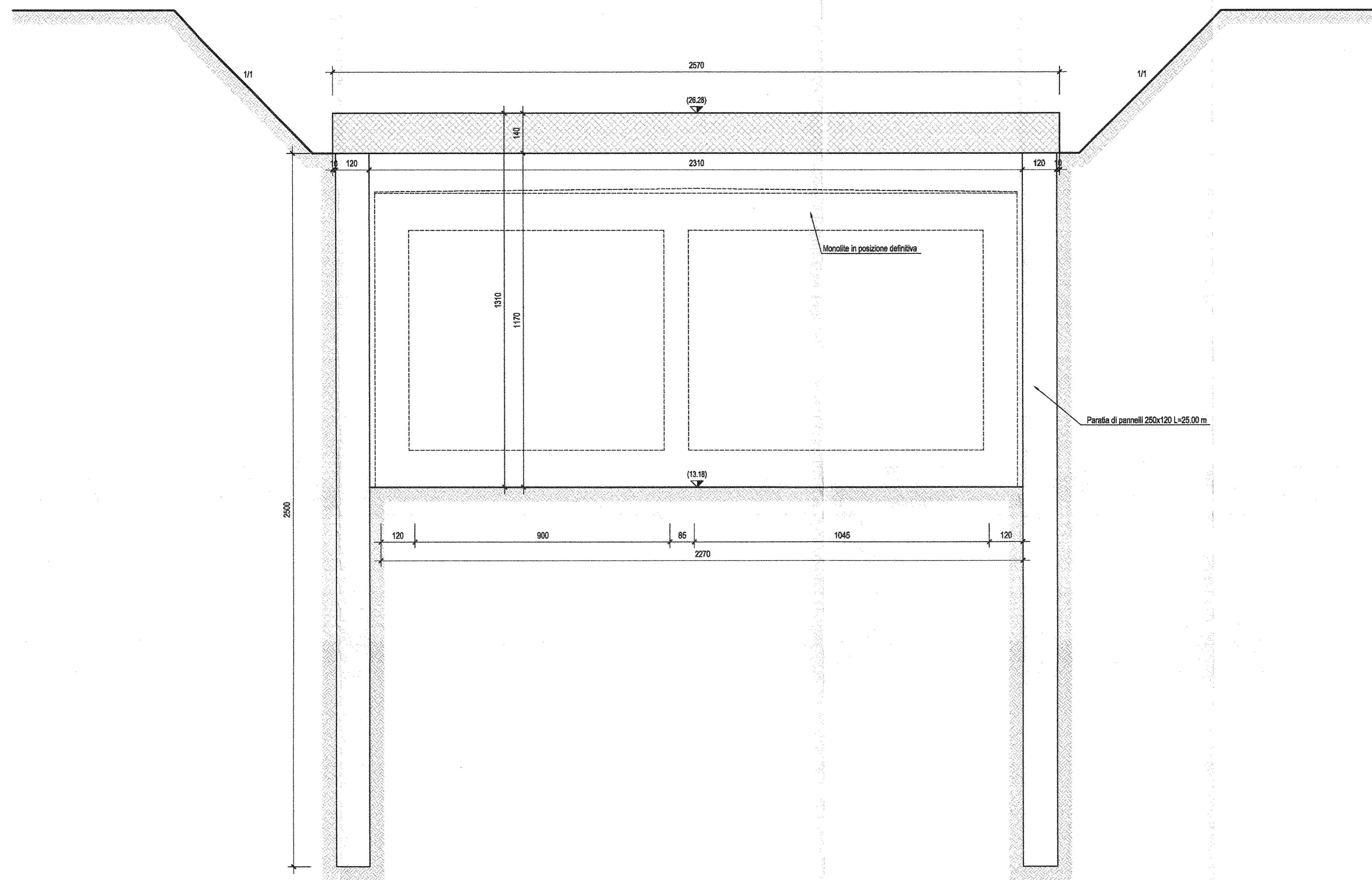
SEZIONE B-B-Scala 1:100
