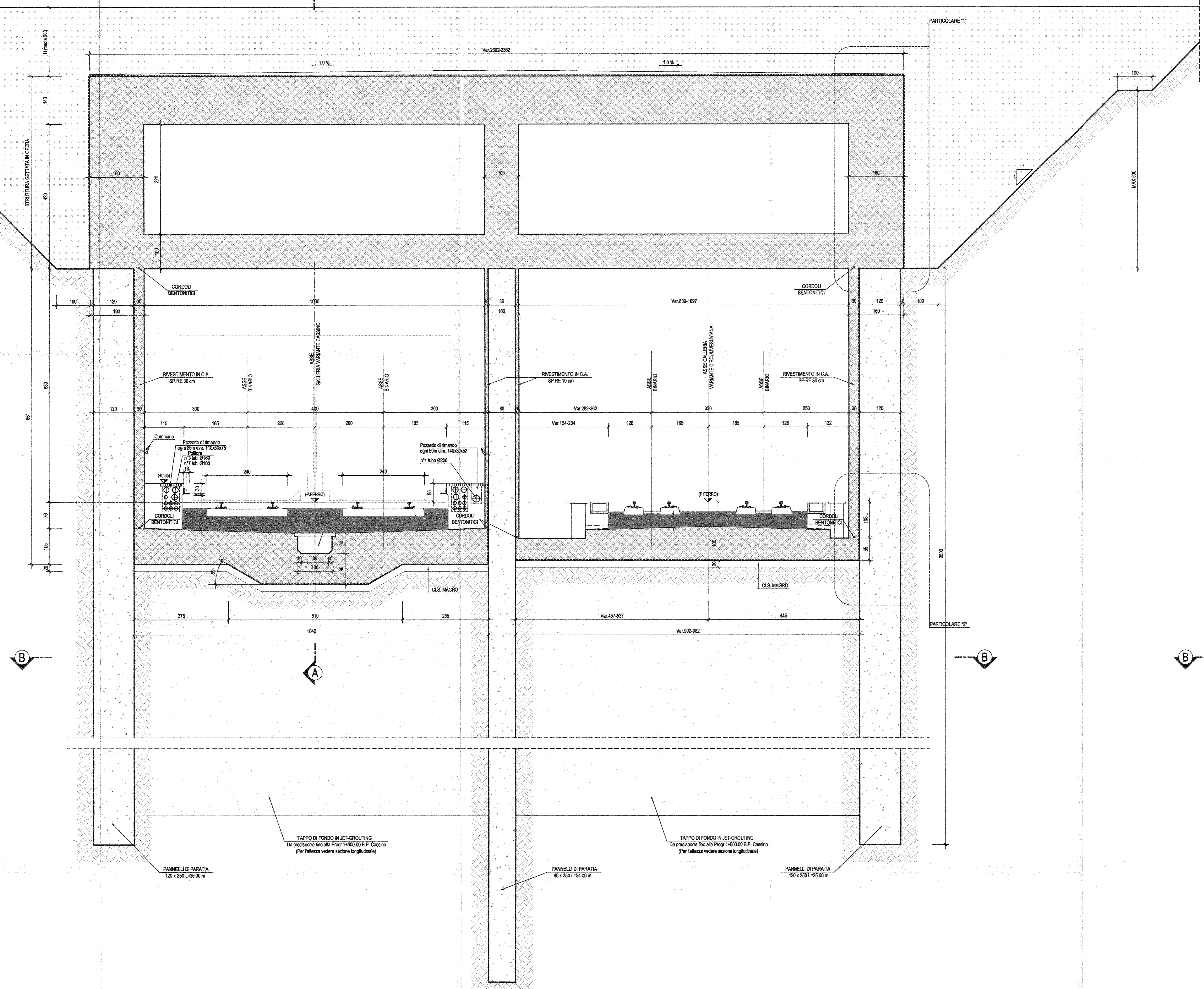
SEZIONE B-B-Scala 1:50
