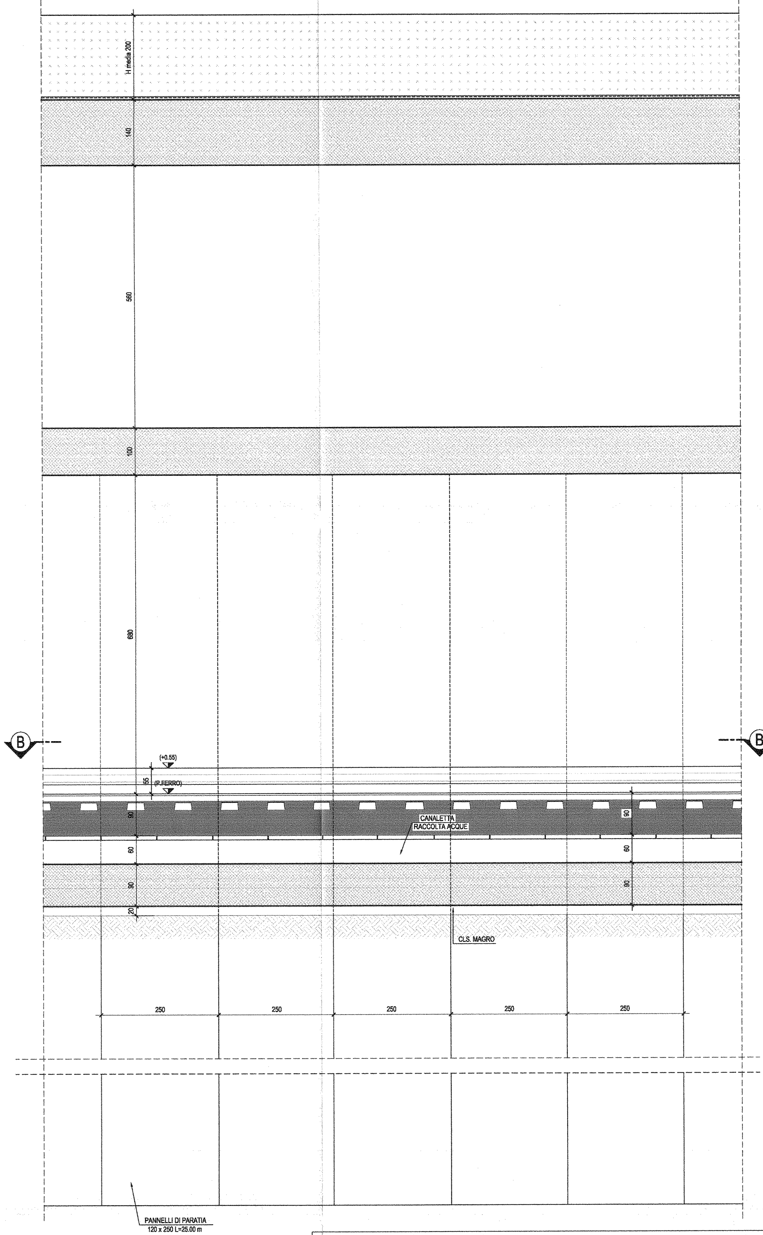
SEZIONE A-A-Scala 1:50
