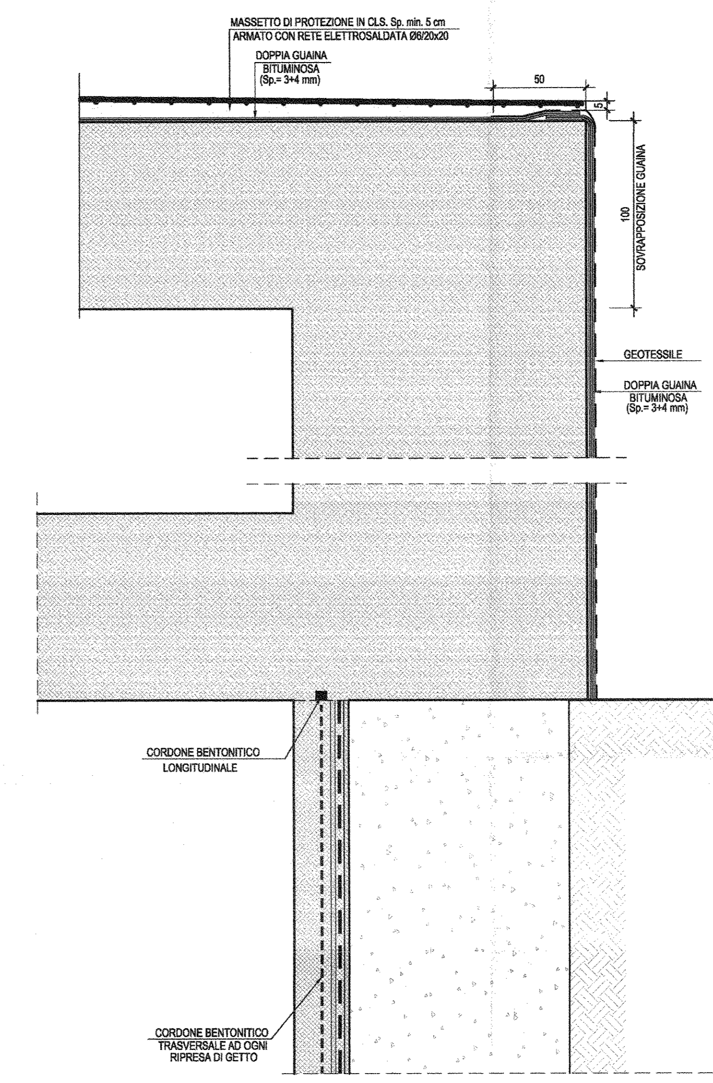
PARTICOLARE "2" - Scala 1:20
