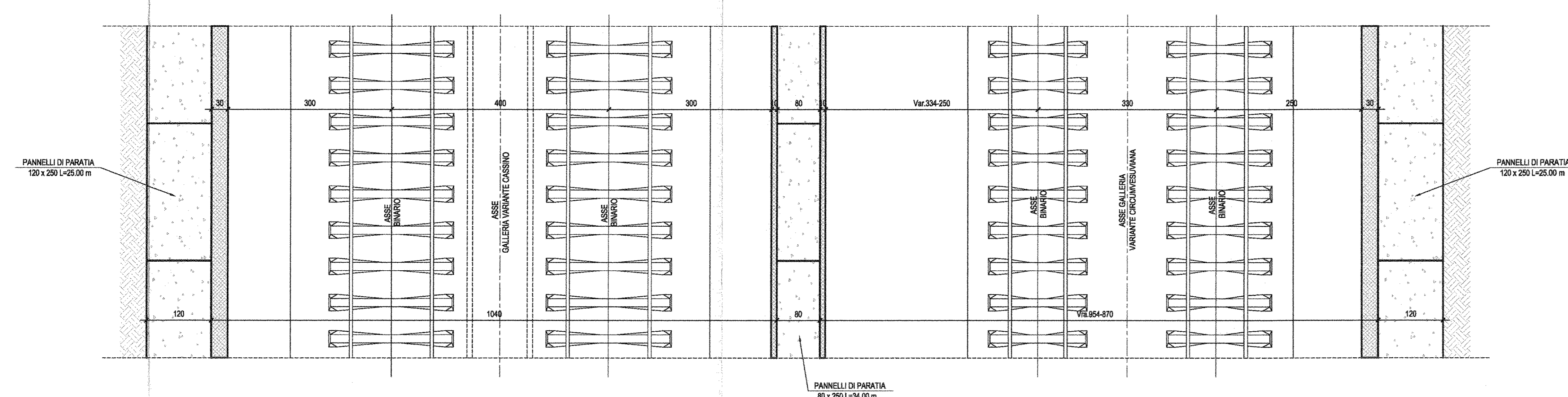
SEZIONE B-B-Scala 1:50
