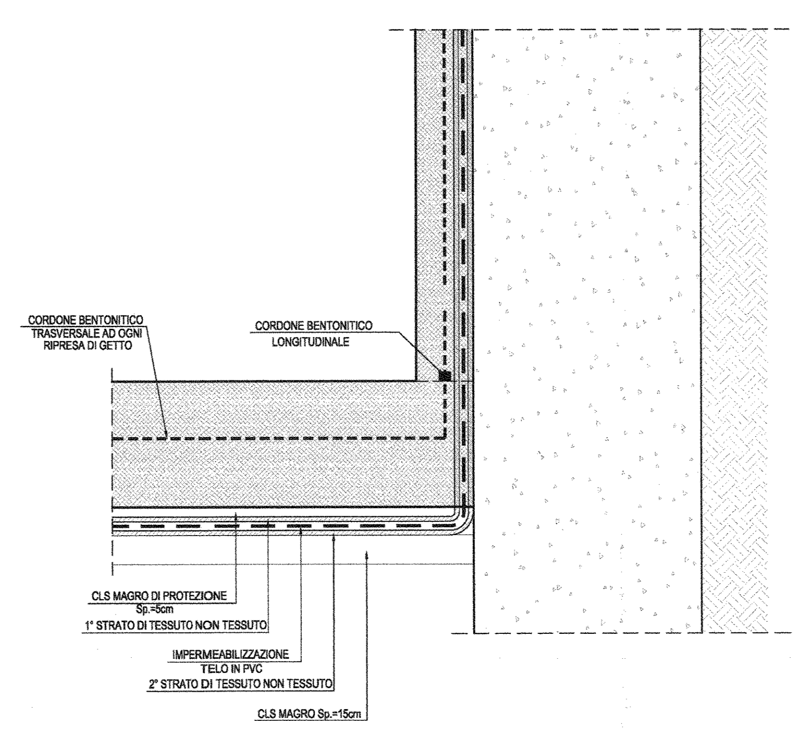
PARTICOLARE "2" - Scala 1:20
