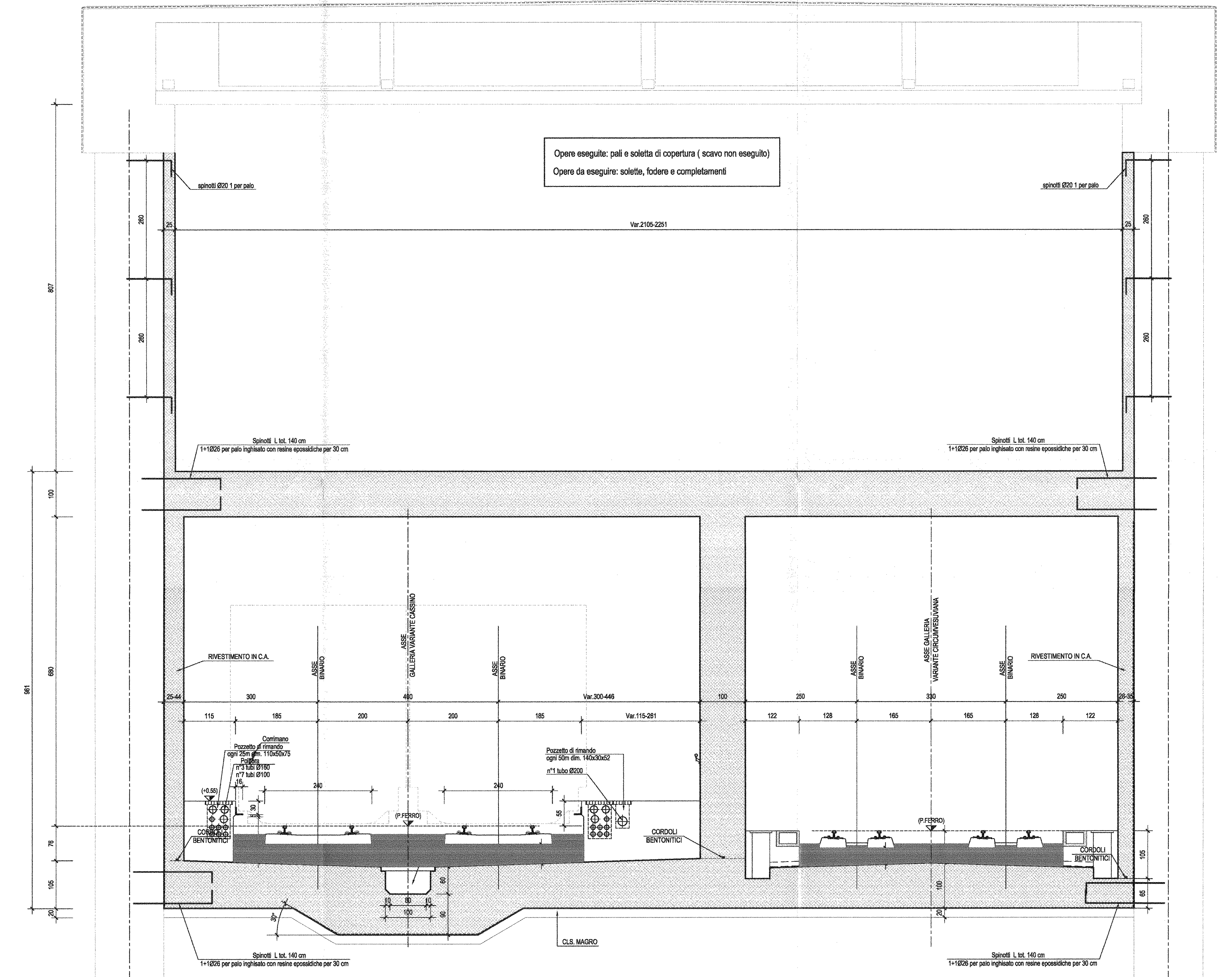
SEZIONE TRASVERSALE COMPLETAMENTO GALLERIA ESISTENTE (SEZIONE B-B)-Scala 1:50 (Valle da km 2+172,24 a km 2+271,14)
