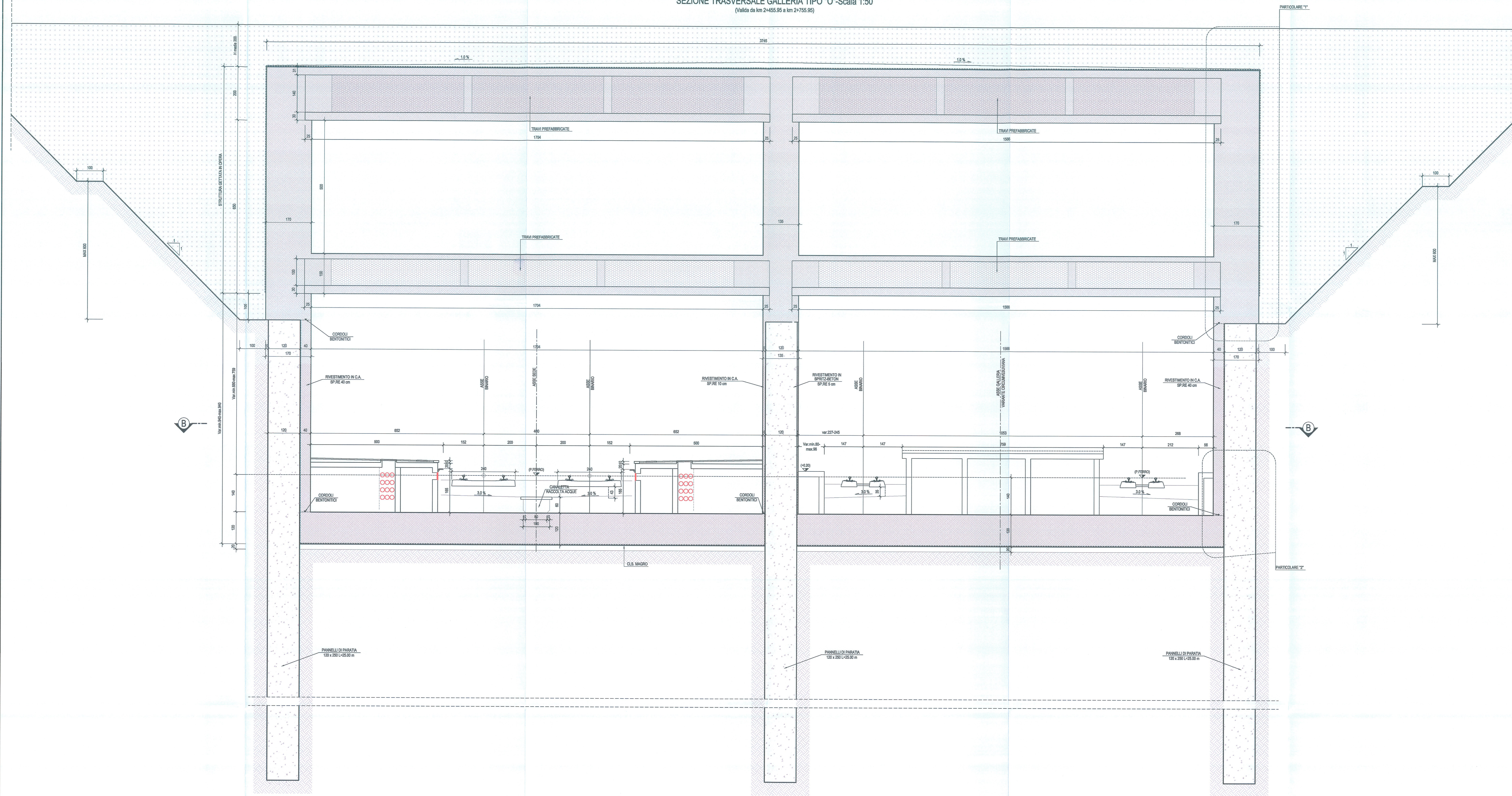
SEZIONE B-B - Scala 1:50
