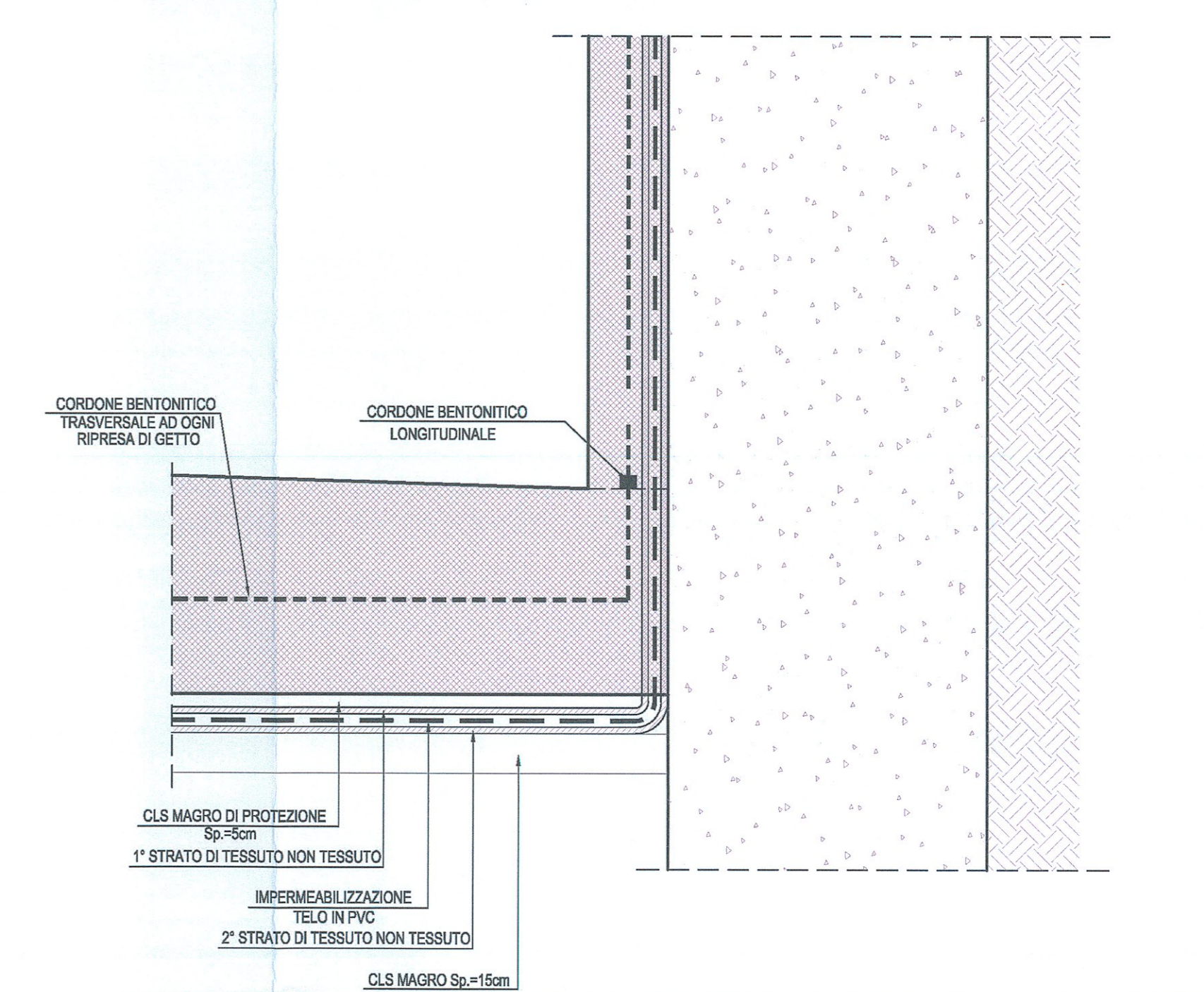
PARTICOLARE "2" - Scala 1:20
