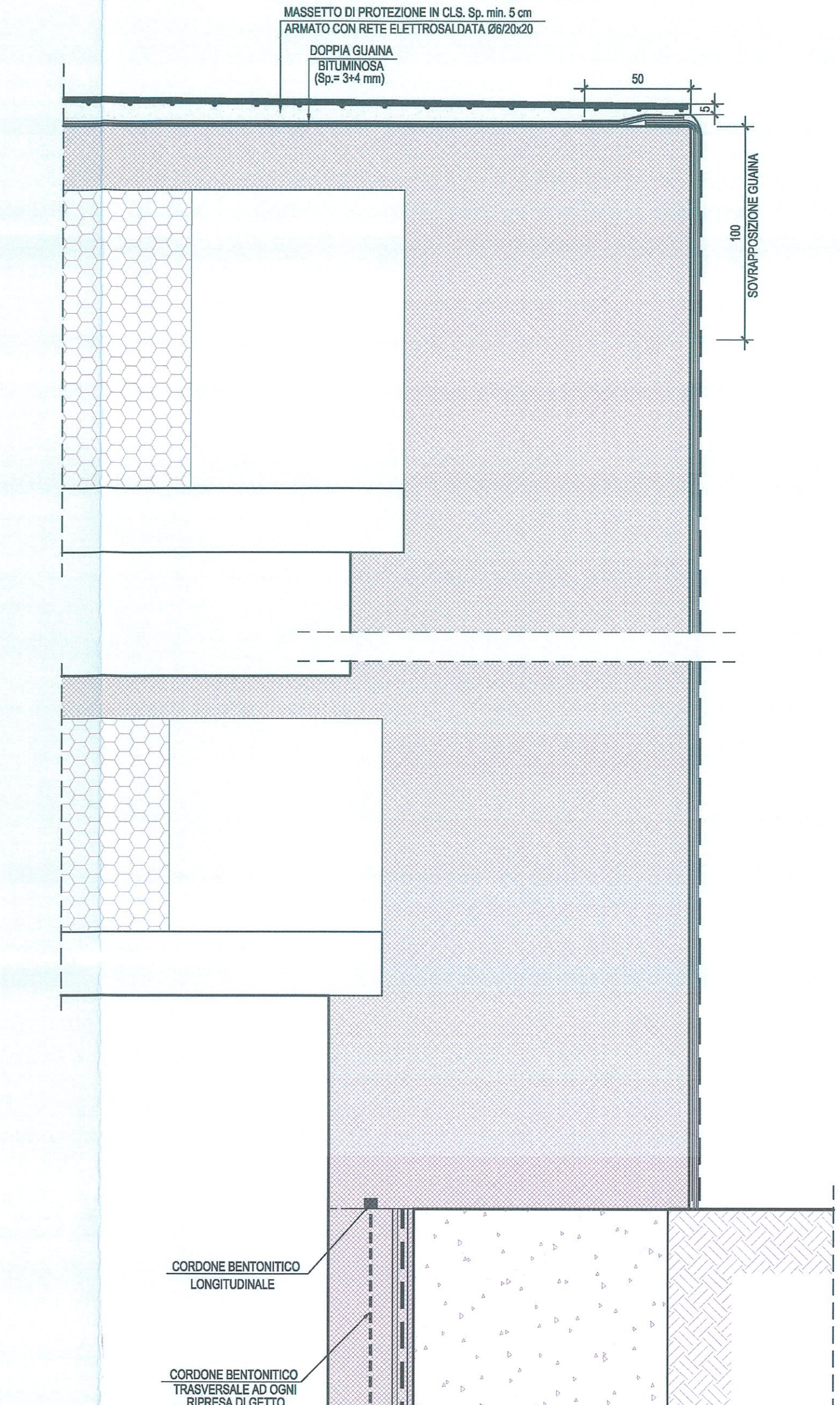
PARTICOLARE "2" - Scala 1:20
