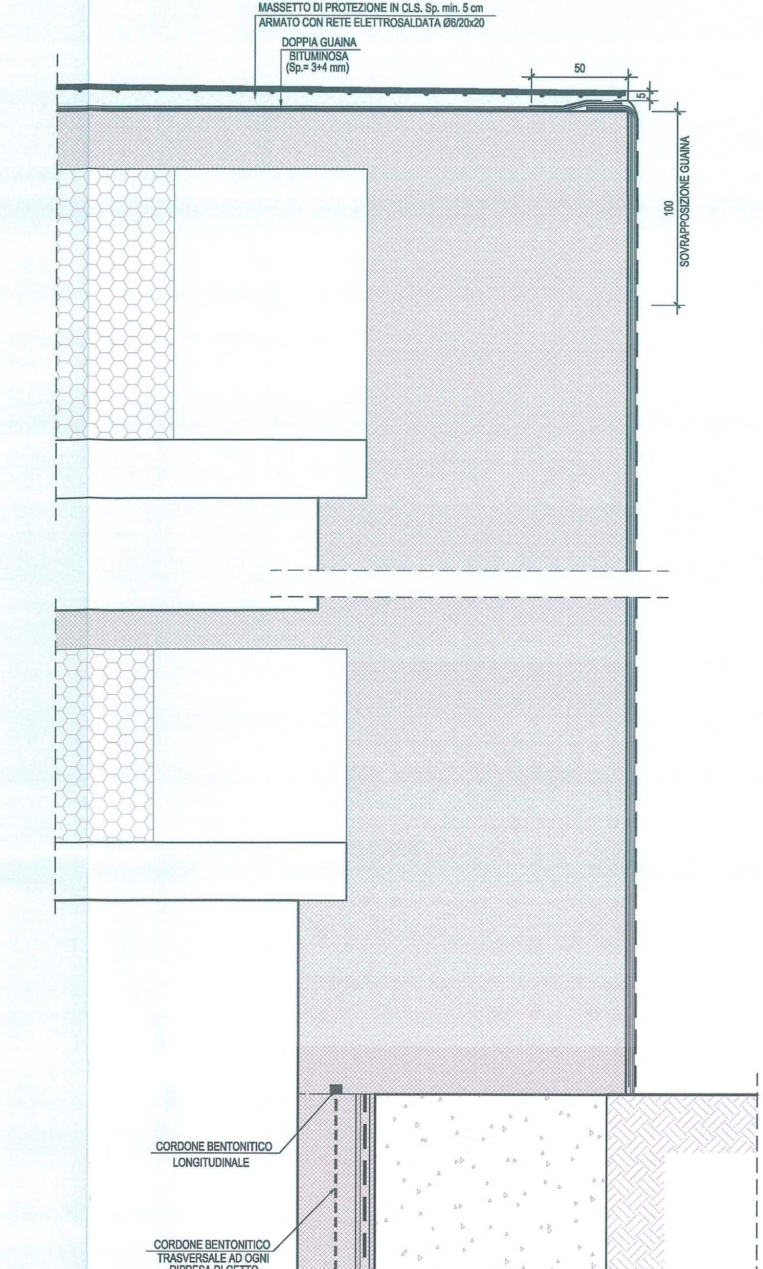
PARTICOLARE "2" - Scala 1:20
