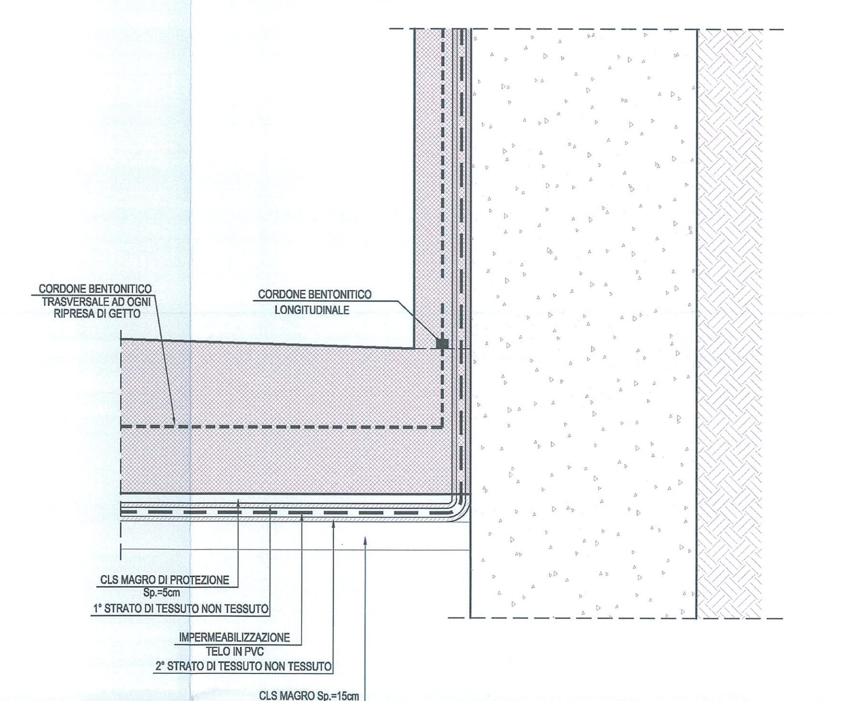
PARTICOLARE "2" - Scala 1:20
