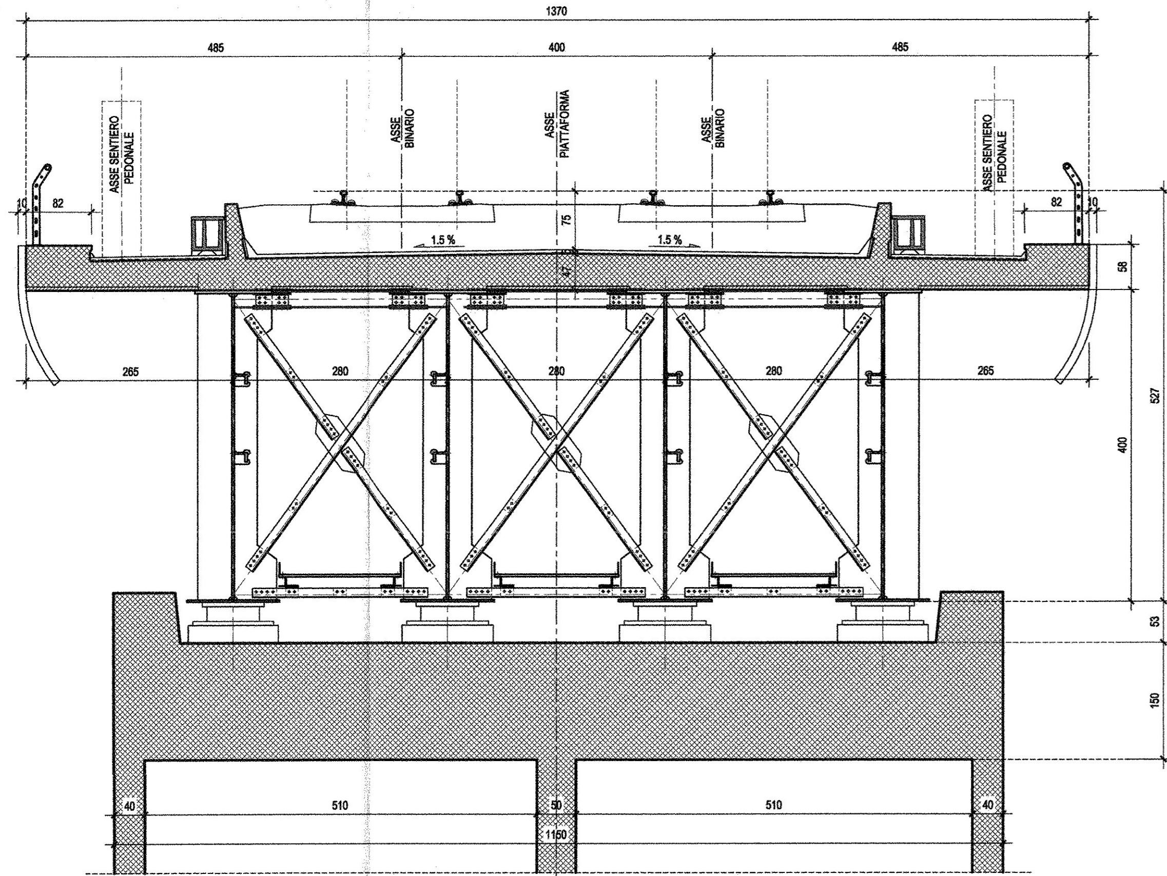
SEZIONE TRASVERSALE TIPO IN ASSE APOGGIO-Scala 1:50 (CAMPATA CONTINUA IN ACCIAIO PILE P21/P24)
