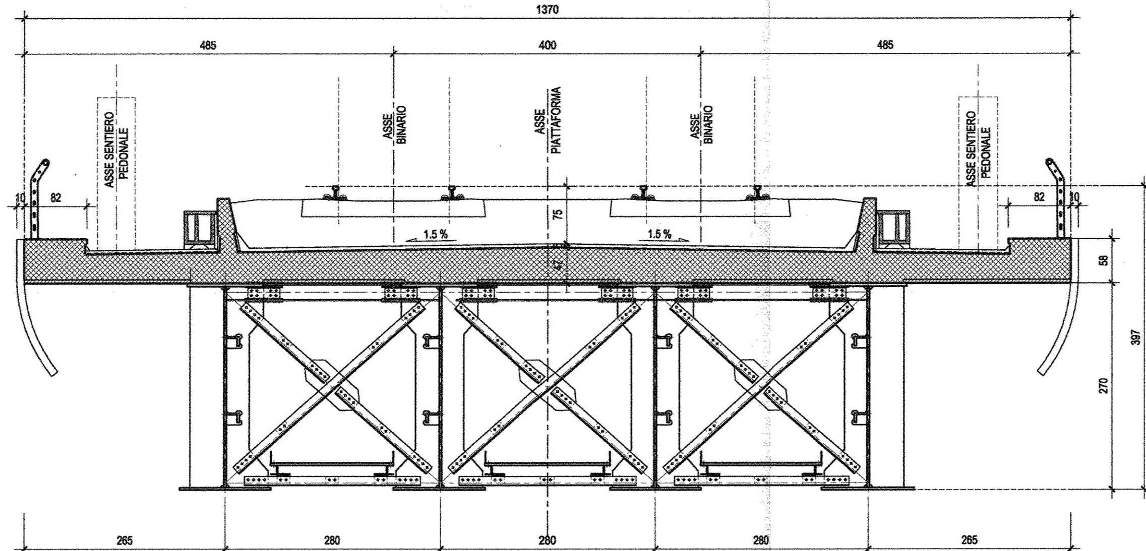
SEZIONE TIPO IN CAMPATA-Scala 1:50 (CAMPATA CONTINUA IN ACCIAIO PILE P21/P24)
