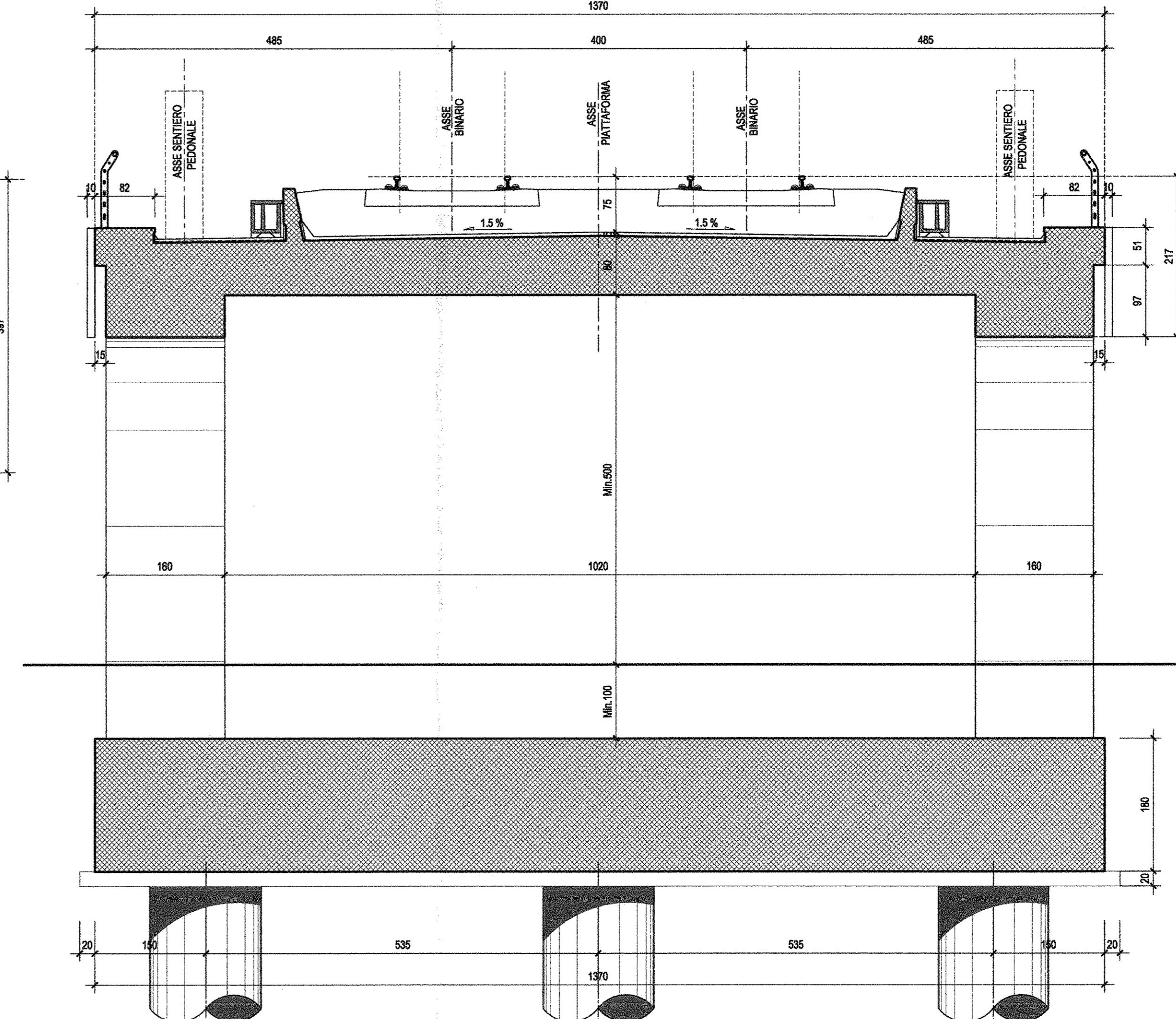
SEZIONE TIPO-Scala 1:50 (CAMPATE ARCHI)
