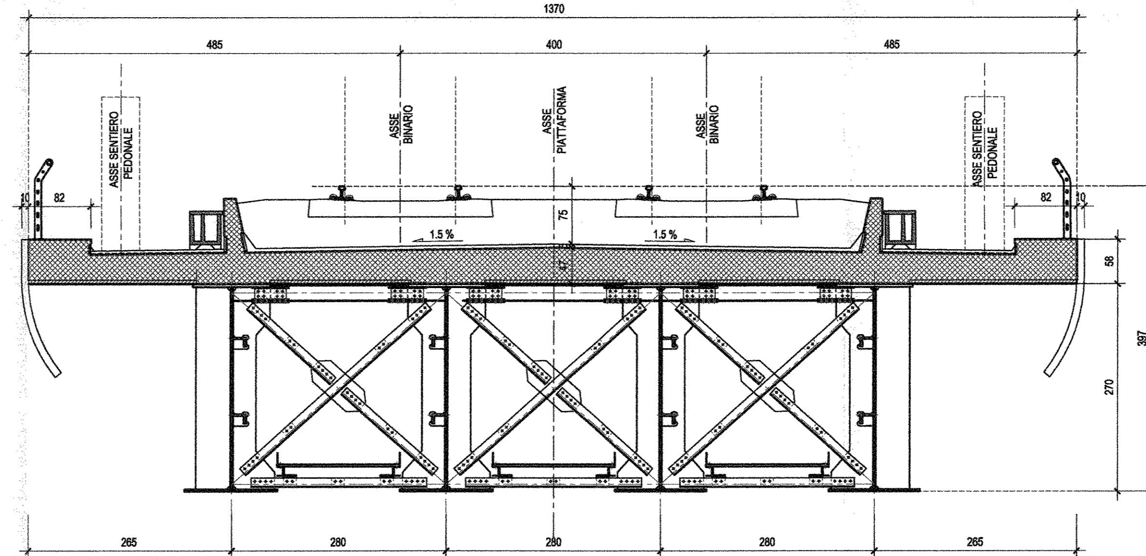
SEZIONE TIPO IN CAMPATA-Scala 1:50 (CAMPATA IN ACCIAIO FILE P42/P44)
