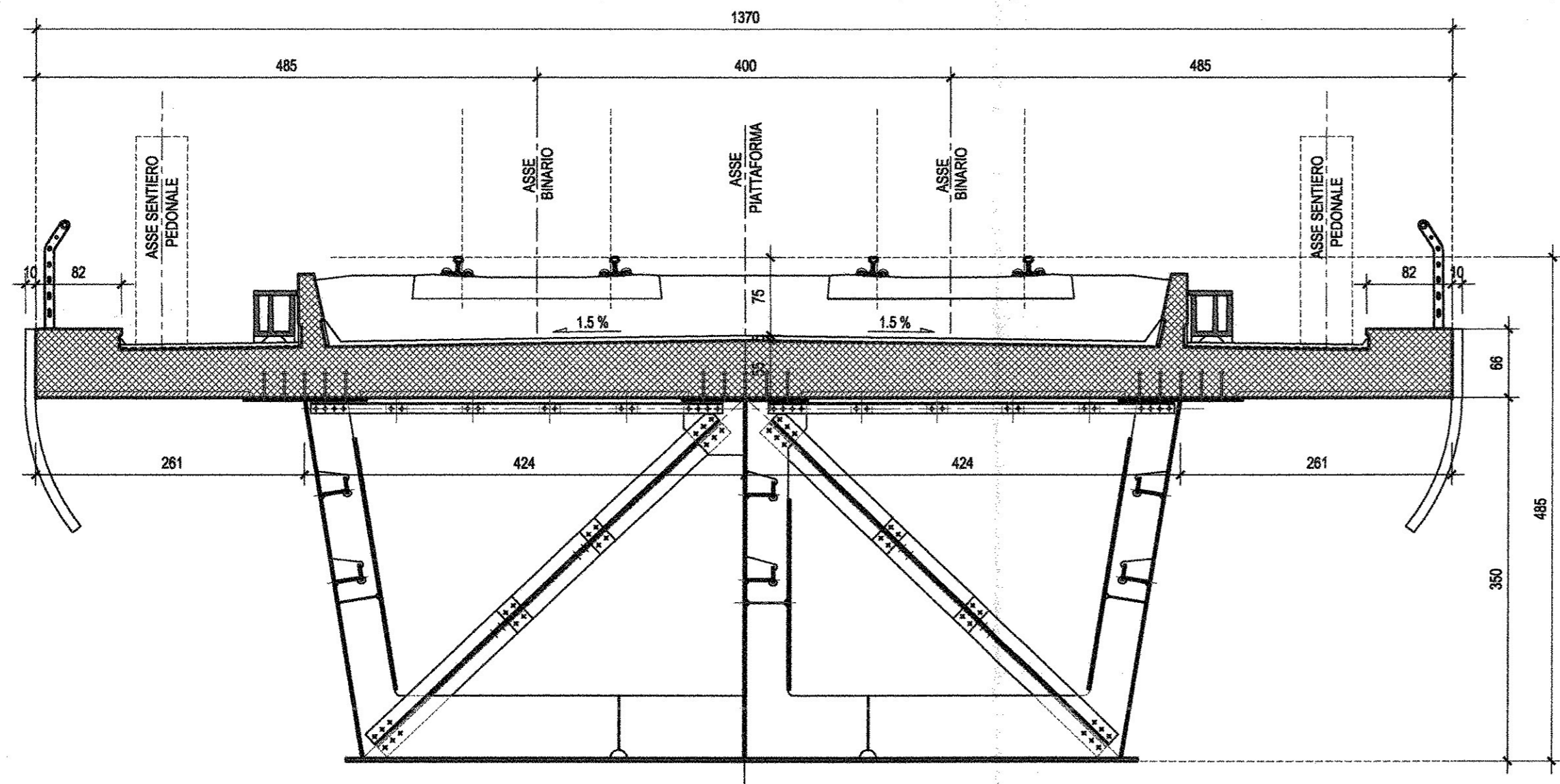
SEZIONE TIPO IN CAMPATA-Scala 1:50 (CAMPATA IN ACCIAIO FILE P41/P42)
