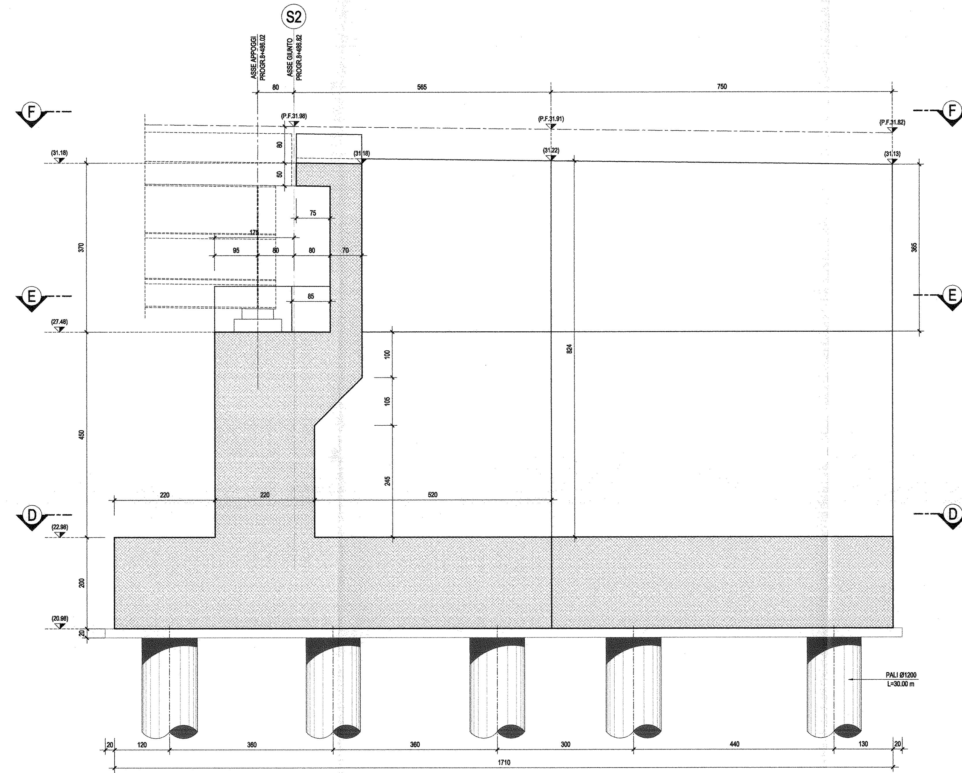
SEZIONE B-B-Scala 1:50
