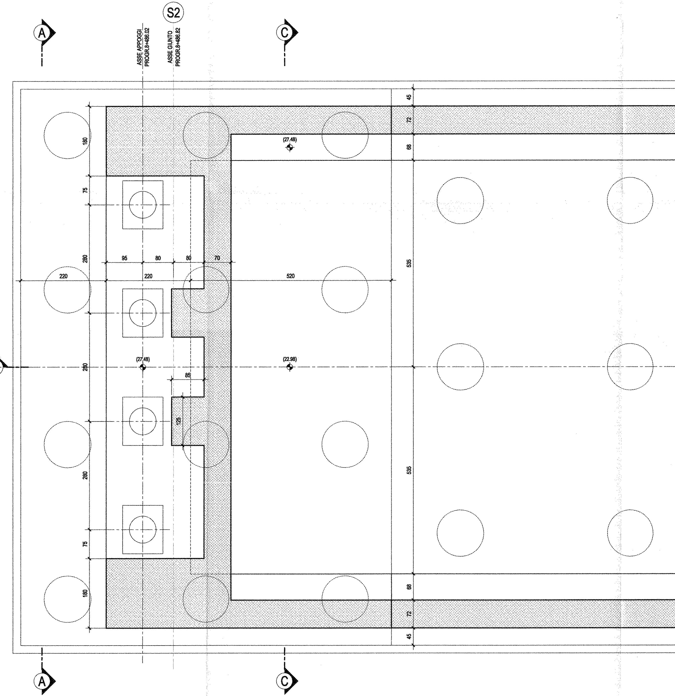
SEZIONE E-E-Scala 1:50
