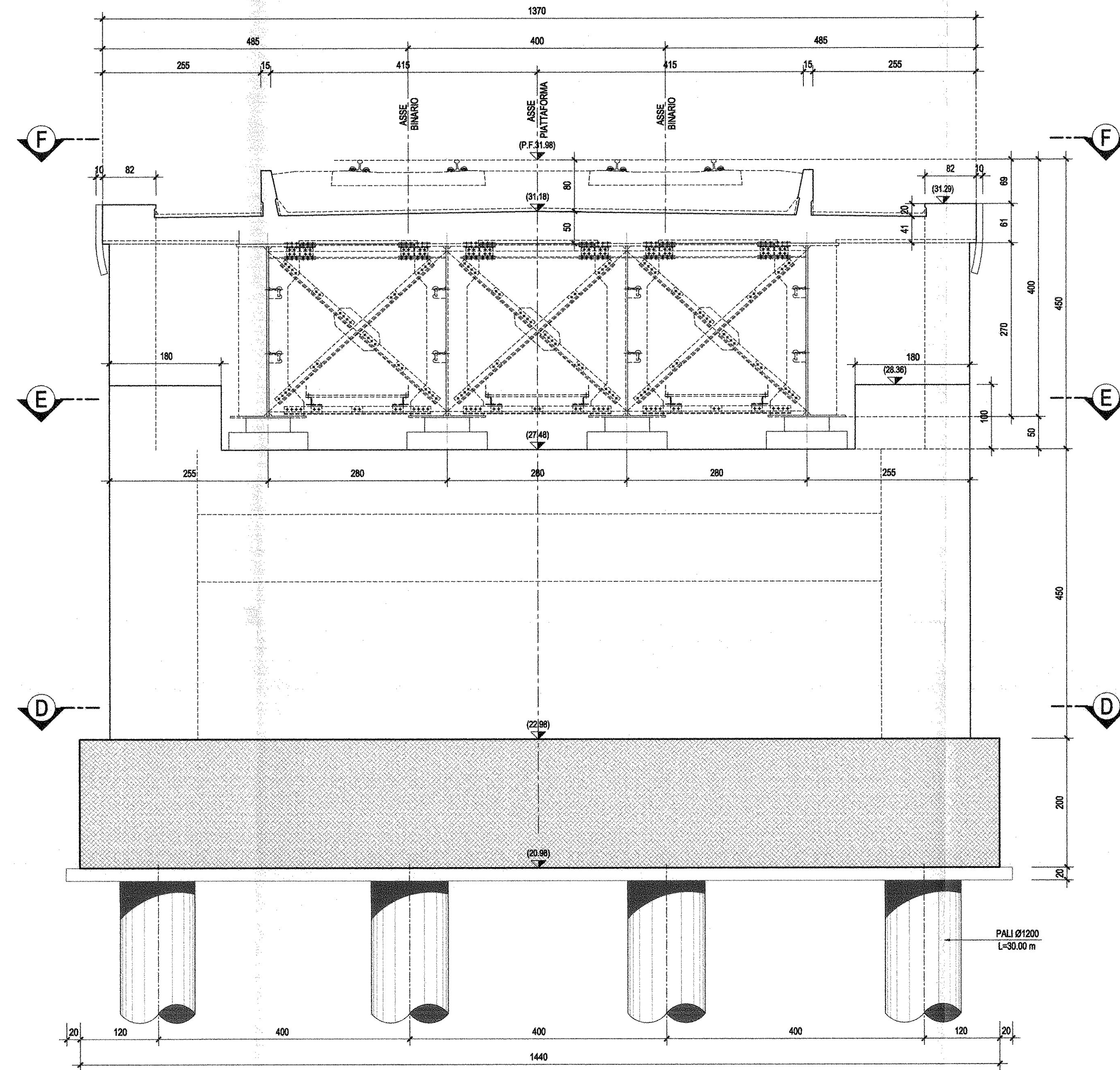
SEZIONE A-A-Scala 1:50
