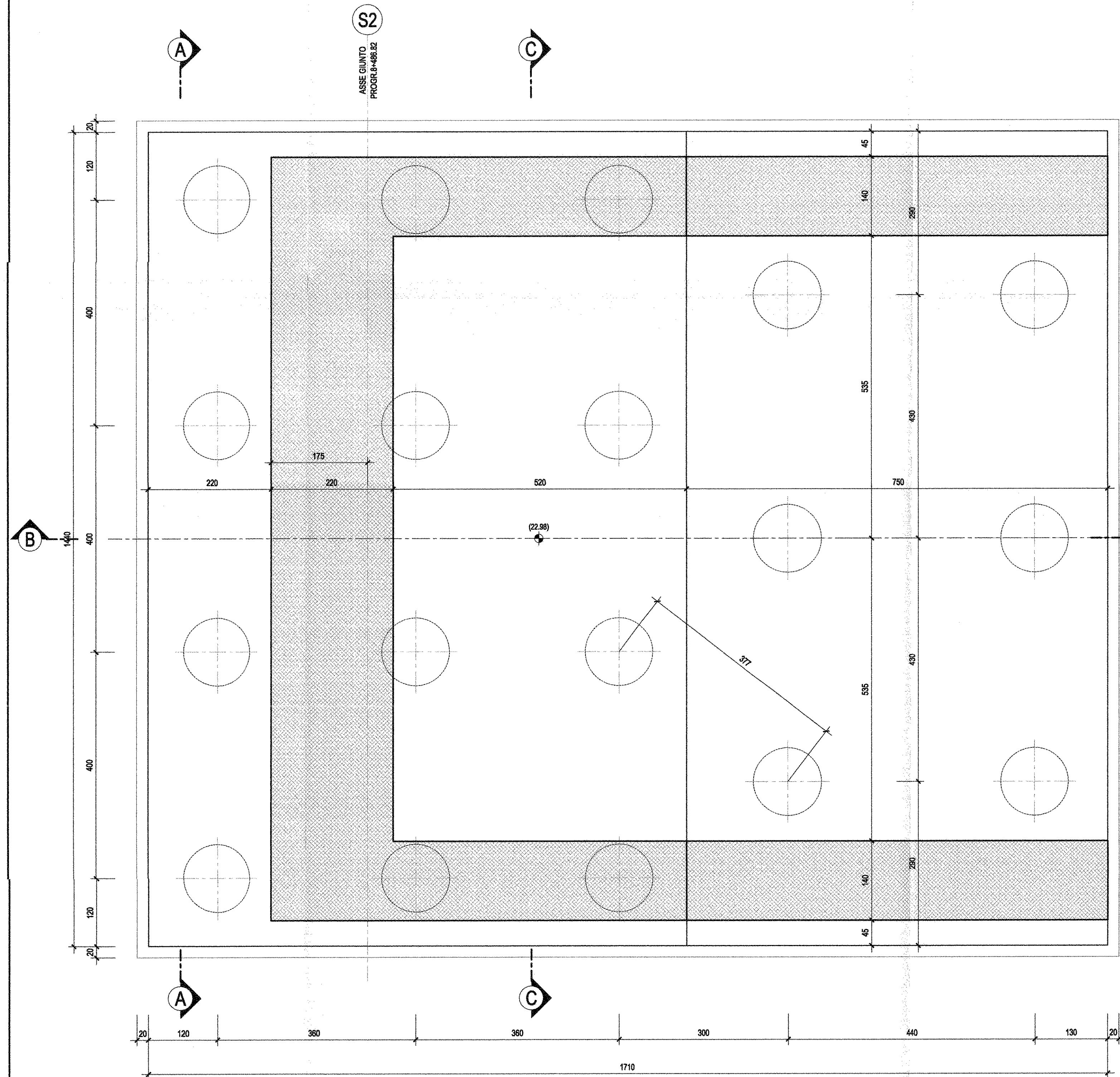
SEZIONE D-D-Scala 1:50
