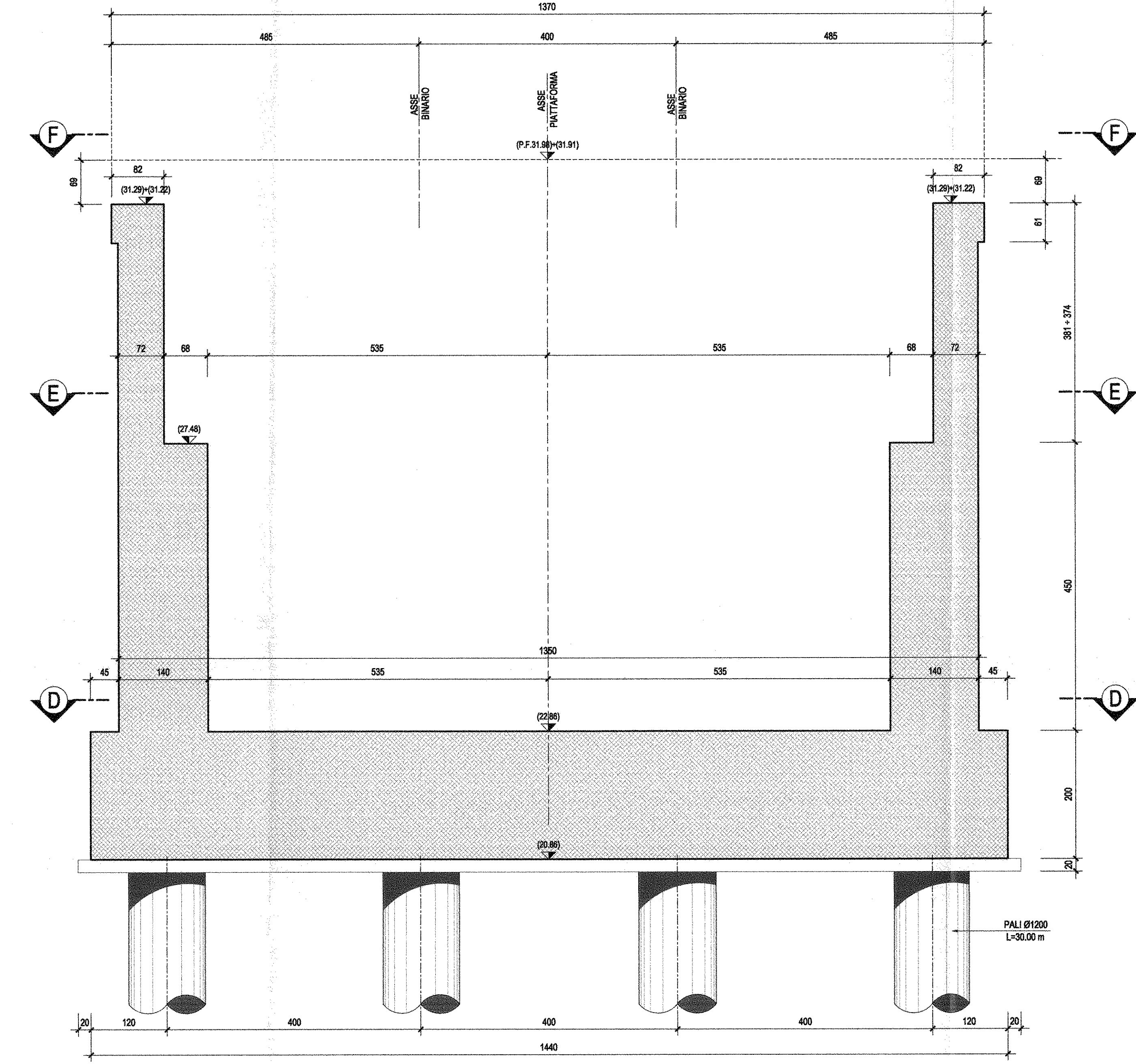
SEZIONE C-C-Scala 1:50
