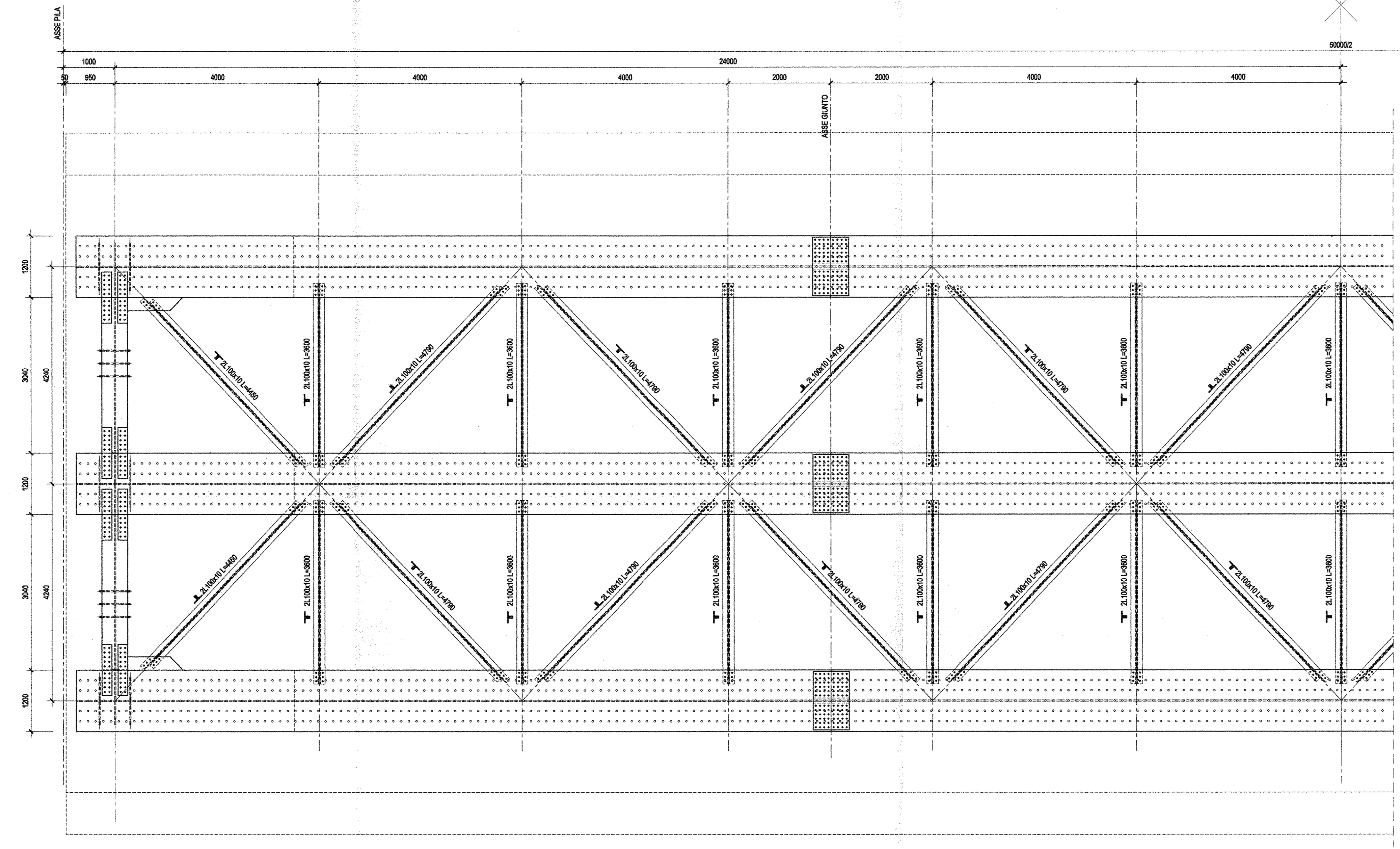
1/2 PIANTA PIATTABANDE SUPERIORI TRAVE-Scala 1:50
