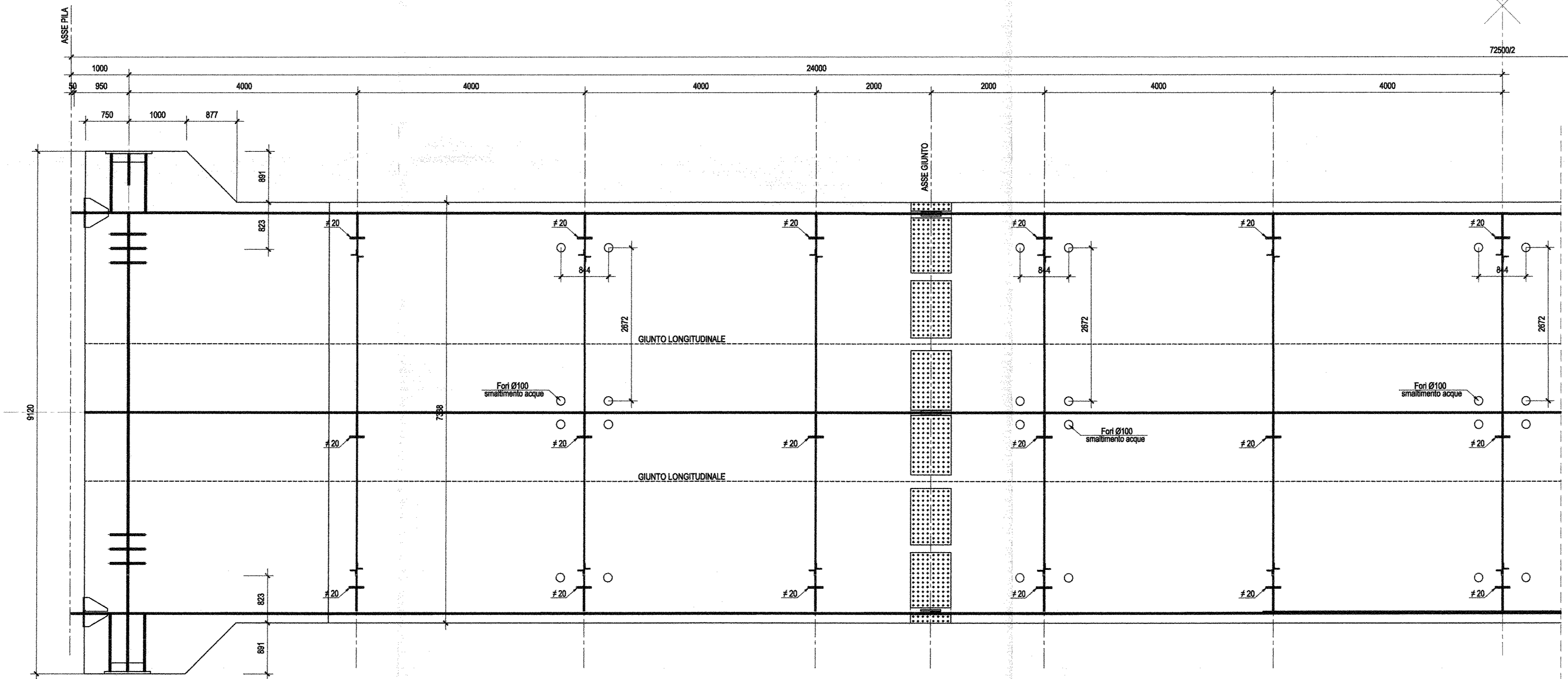
1/2 PIANTA PIATTABANDE INFERIORI TRAVE-Scala 1:50
